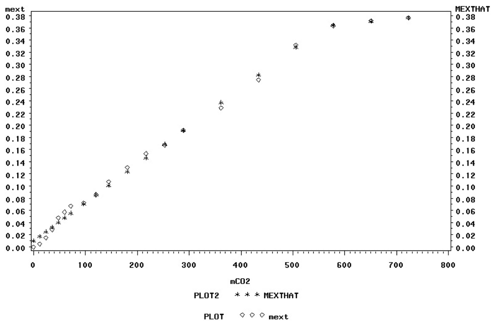
Figura IIIA.2 – Gráfico SAS de ajuste para ESC 100 bar/30 °C.
