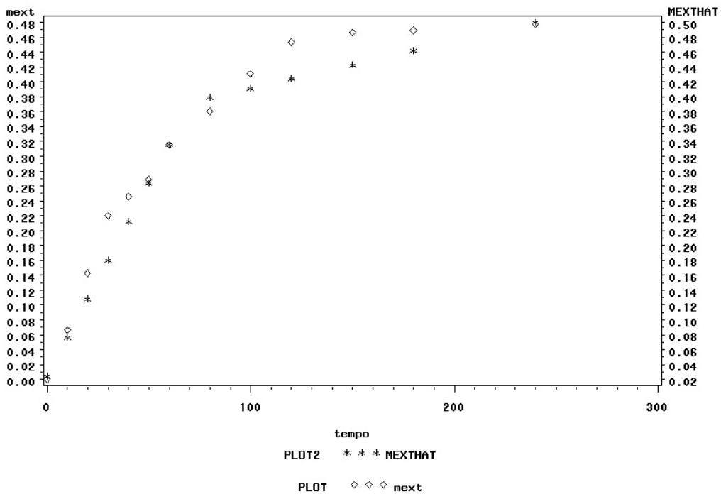
Figura IVE.2 – Gráfico SAS de ajuste para ESC 300 bar/40 °C.
