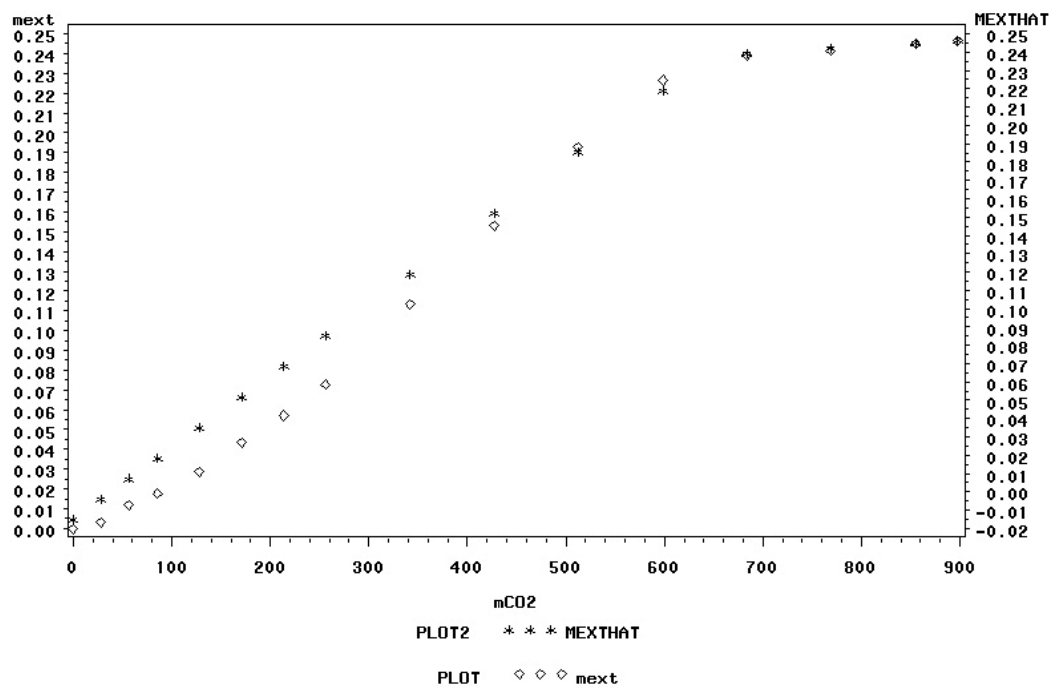
Figura IIB.2 – Gráfico SAS de ajuste para ESC 100 bar/40 °C.
