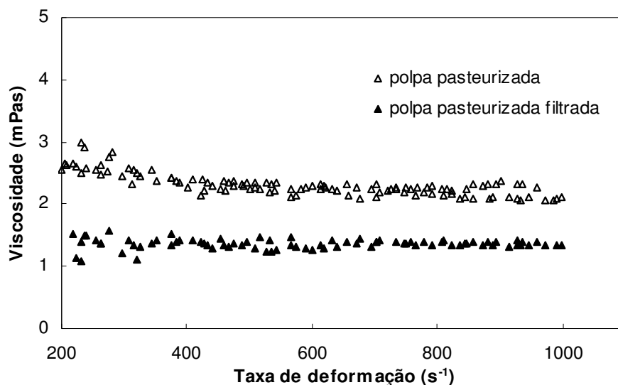
FIGURA 5.5 – Comportamento reológico da polpa pasteurizada não filtrada e filtrada.
