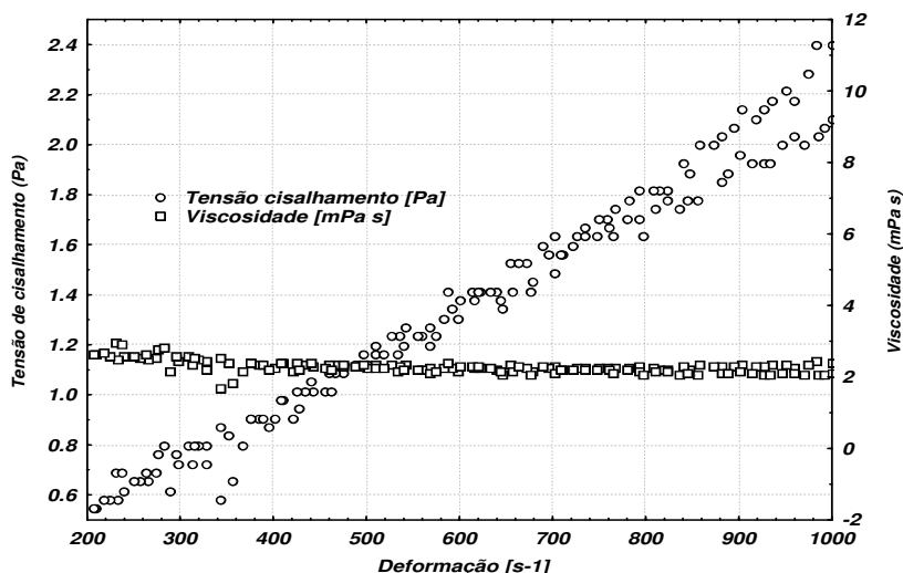
FIGURA 5.2 – Comportamento Reológico da polpa pasteurizada
