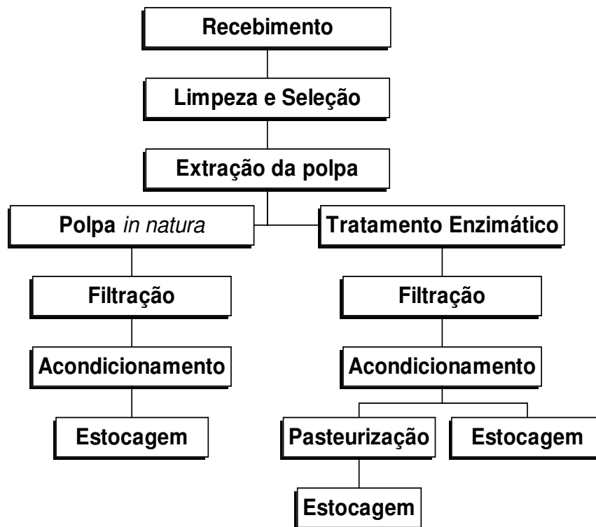
FIGURA 4.1 – Fluxograma de Produção da Polpa de Carambola.
