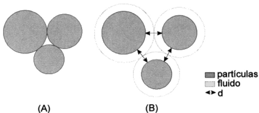
FIGURA 2.7 - Desenho esquemático da parcela de água ocupada no reconhecimento da superfície e preenchimento dos interstícios entre partículas em contato (a), e da parcela que promove a separação entre as partículas da suspensão (b) (ORTEGA, 1999).
