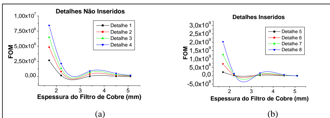
Figura 4.5 - Variação da FOM com a espessura do filtro de cobre para os detalhes não inseridos (a) e inseridos (b), para a peça de Al
