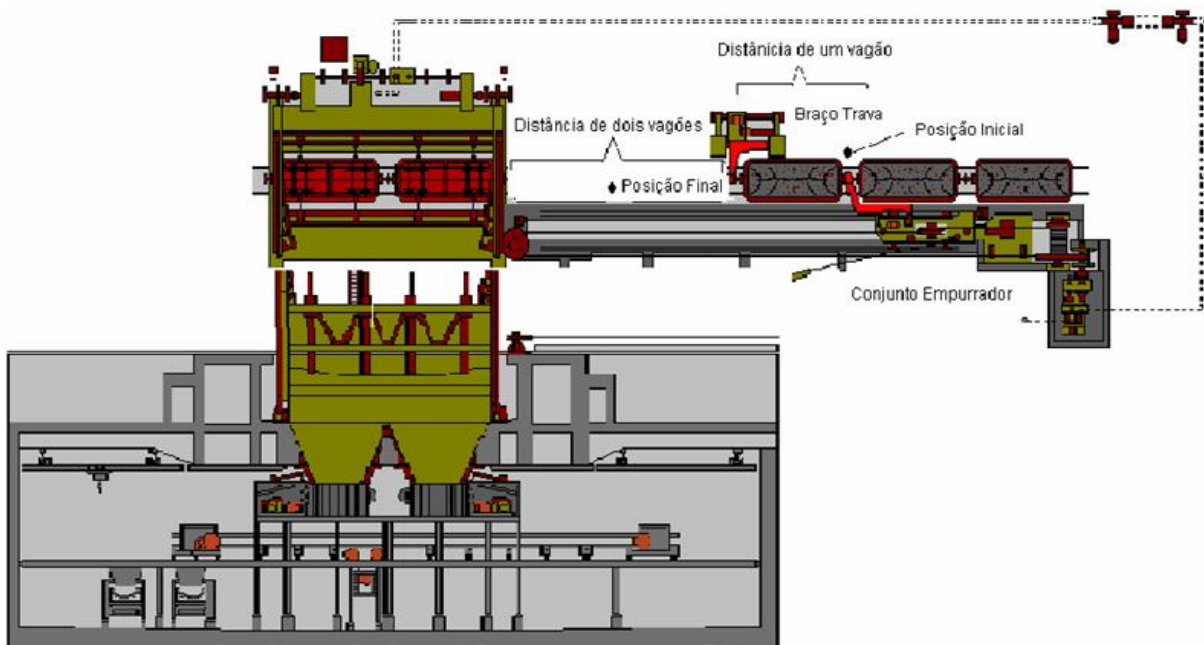
Figura 8 – Posicionamento inicial do carro posicionador e braço trava
