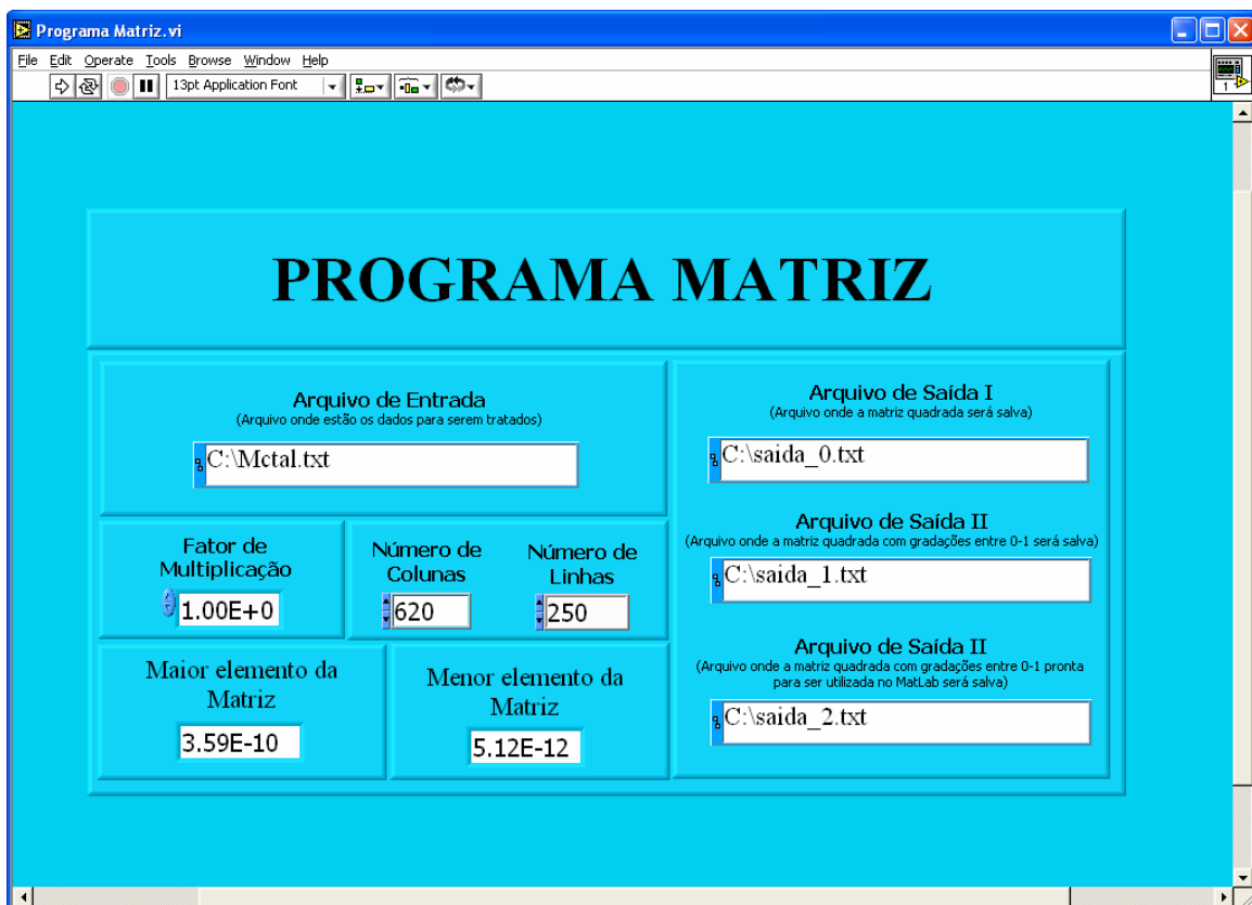
Figura 28 – Interface do PROGRAMA MATRIZ .
