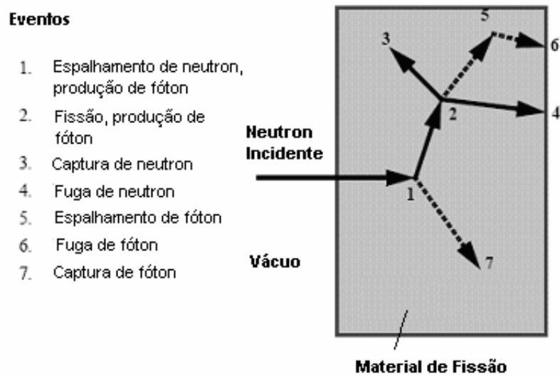
Figura 23 – Representação da história de um nêutron incidente em uma placa de material fissil.
