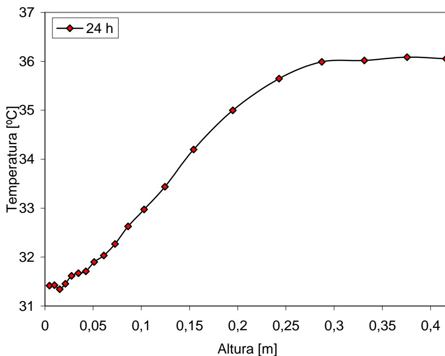
Figura 6.27 – Perfil de temperatura após 24 horas de resfriamento.
