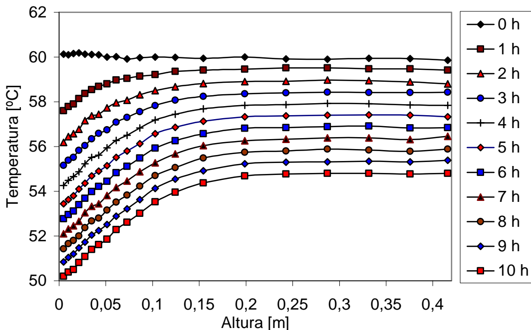
Figura 6.6 – Perfis experimentais de temperatura para 10 horas de resfriamento a partir de campo inicial a 60°C.
