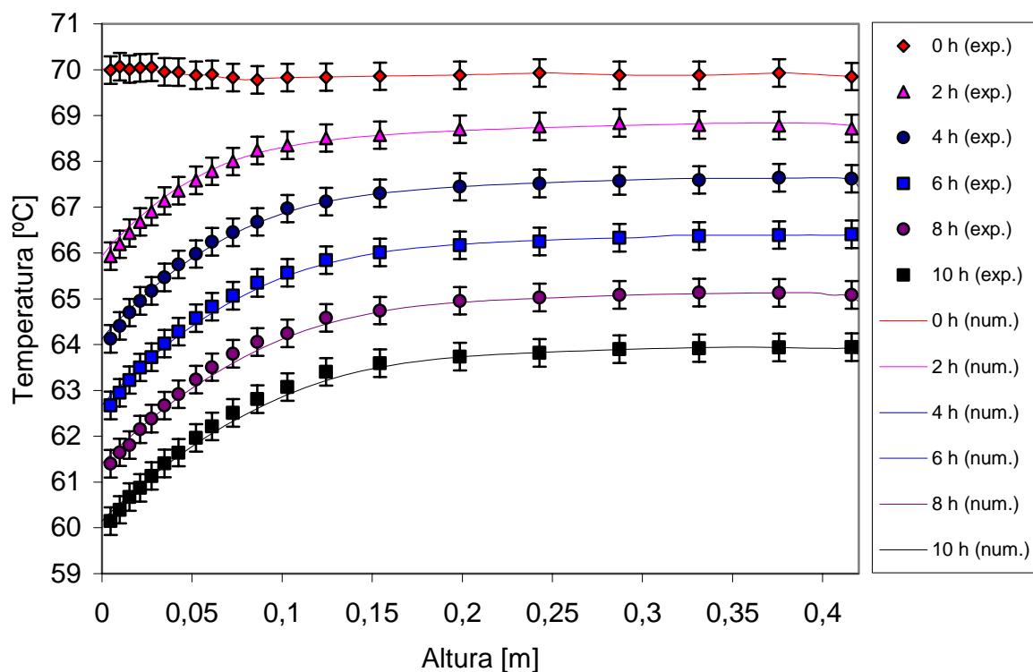
Figura 7.14 - Comparação entre os perfis de temperatura para um resfriamento com temperatura inicial de 70°C, com temperatura ambiente variável.
