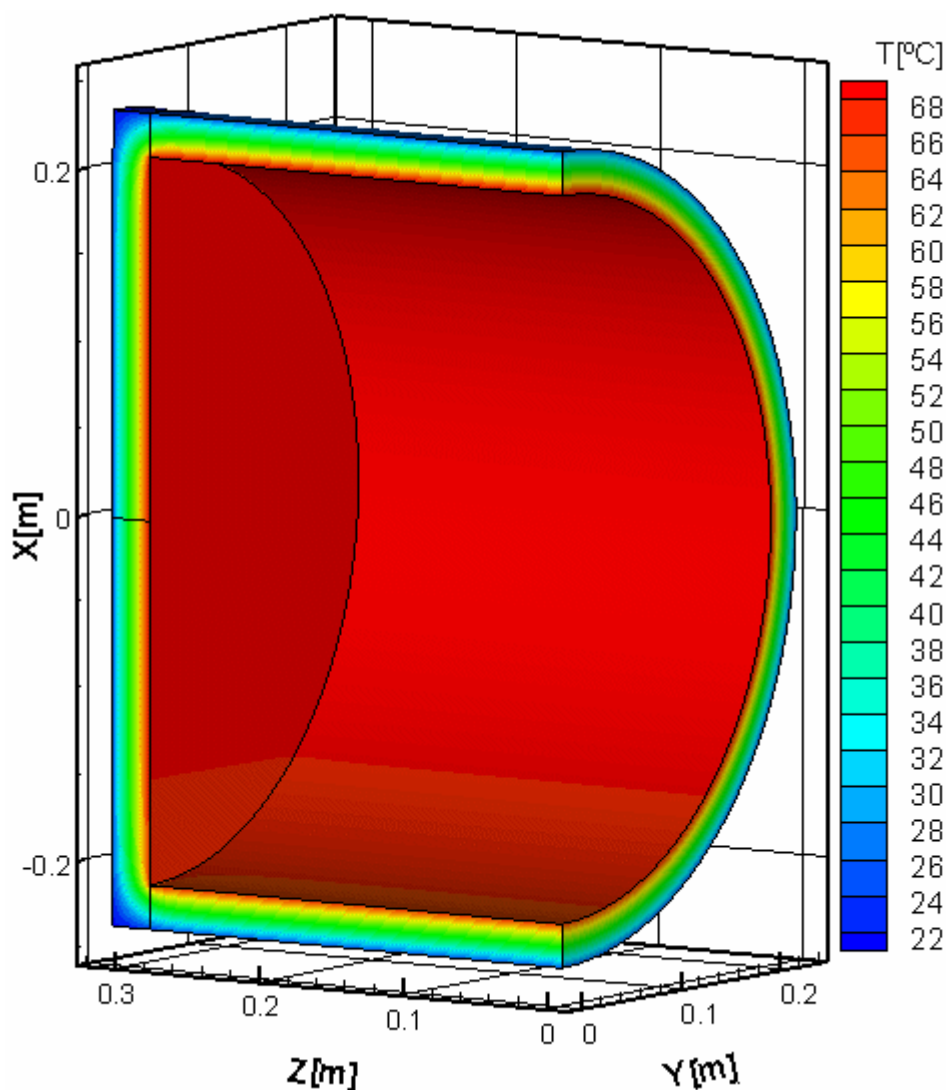
Figura 2 – Visão do campo de temperatura na região do isolamento térmico, excluía a região ocupada pelo fluido.
