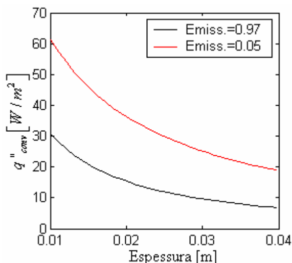
Figura 7.32 - Fluxo de calor por convecção.
