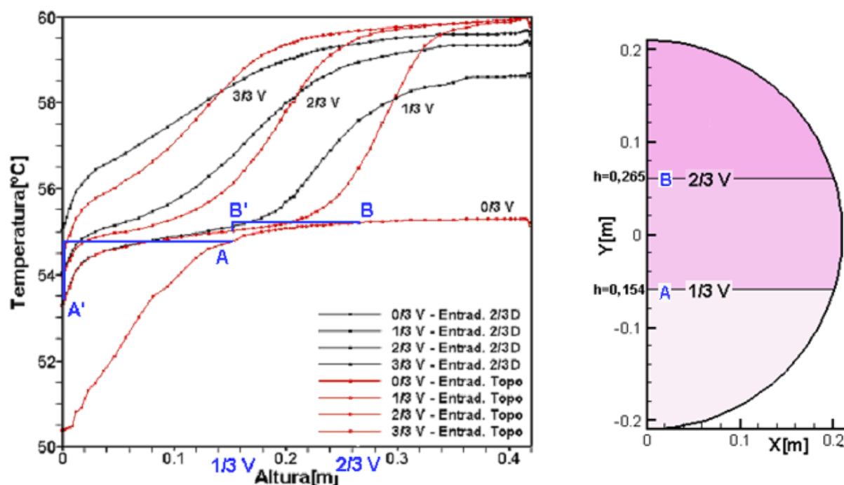
Figura 8.18 - Perfis de temperatura correspondentes ao ingresso de água a 60°C em volumes iguais a 1/3, 2/3 e 3/3 do volume total do reservatório, para os casos onde o jato de entrada situa-se numa altura a 2/3 do diâmetro e no topo. À direita, divisão do volume em três camadas.
