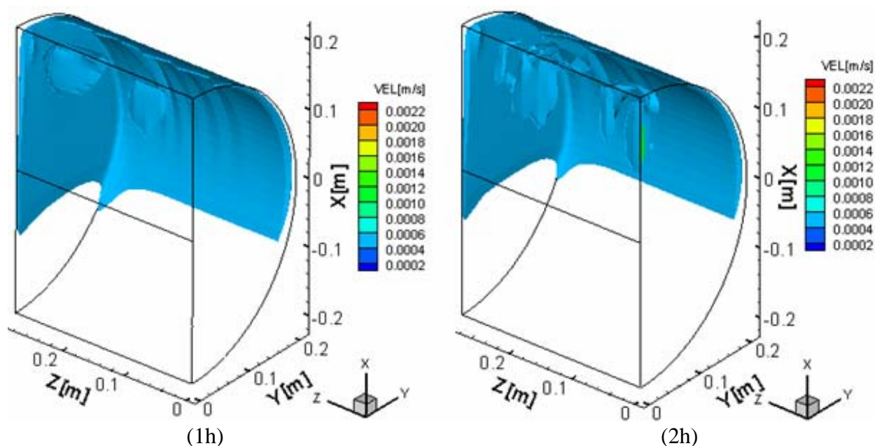
Figura 7.10 – Módulo das componentes do vetor velocidade para instantes 1h e 2h.
