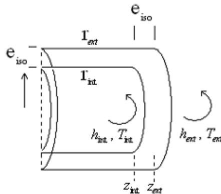
Figura 7.27 - Parâmetros envolvidos no cálculo do coeficiente global de perdas.
