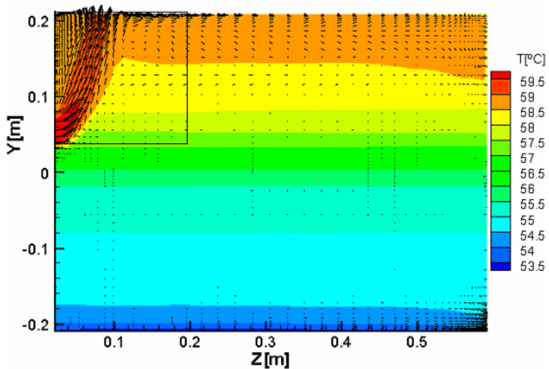
Figura 8.3 – Vista do campo de temperatura no plano de simetria para o caso sem anteparo, após ingresso de 26 litros de água a 60°C, ao longo de 26 min.
