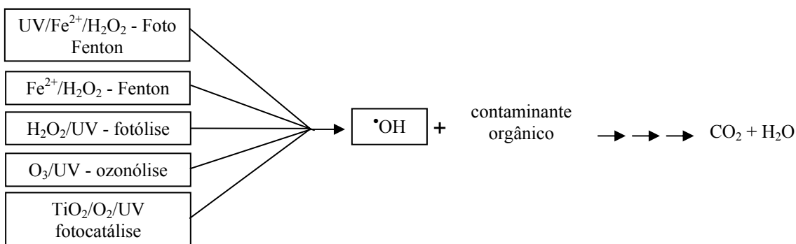
Figura 1.1: Esquema representativo dos POAs utilizados para a oxidação de contaminantes orgânicos.
