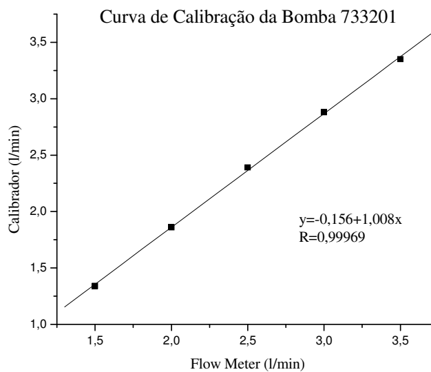
Figura A.8. Curva de calibração da bomba 8.
