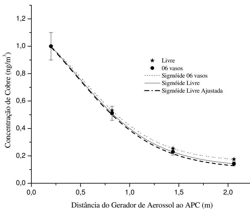
Figura 4.6. Ajuste de sigmóide do arranjo livre para o arranjo III.
