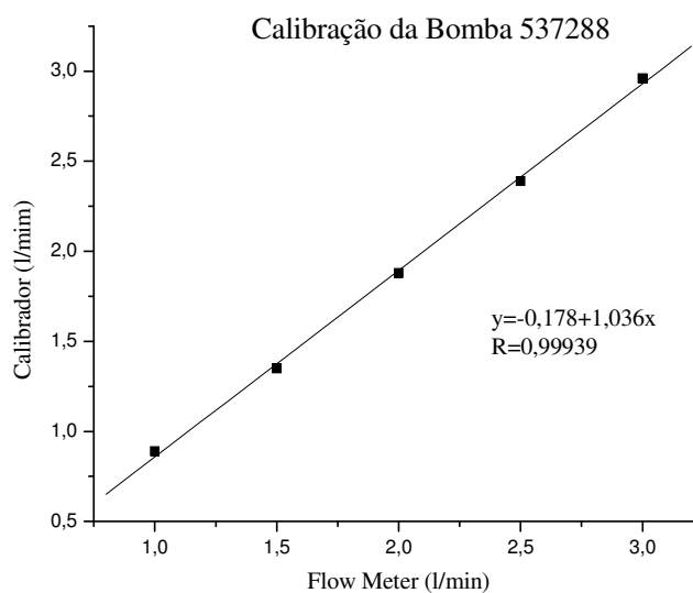
Figura A.6. Curva de calibração da bomba 6.
