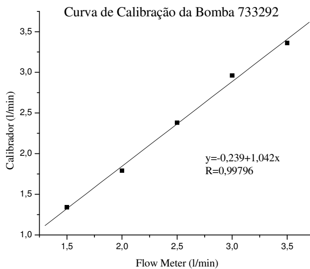
Figura A.9. Curva de calibração da bomba 9.
