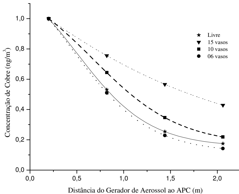
Figura 4.3. Curvas das sigmóides obtidas para os arranjos estudados.
