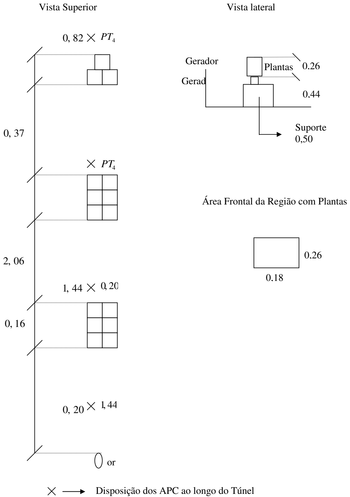
Figura 3.5. Disposição dos vasos de plantas no arranjo I.
