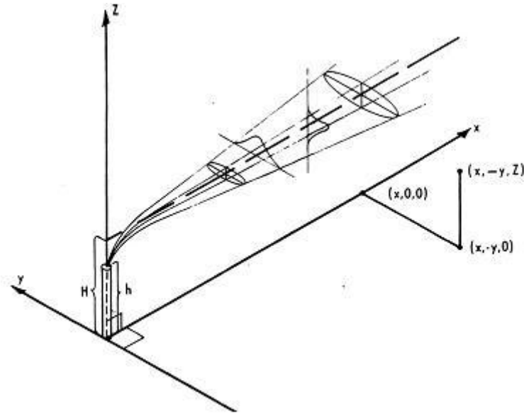
Figura 2.5. Esquema de coordenadas utilizadas nas equações de pluma gaussiana (EPA, 1970).
