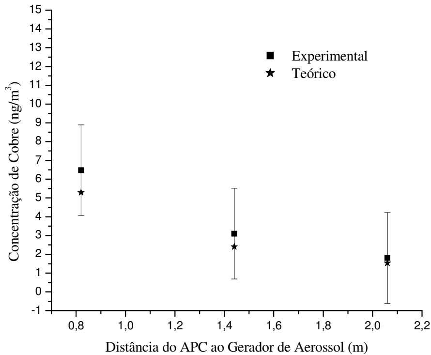
Figura 3.4. Comparação de resultados teóricos e experimentais do segundo teste sem plantas.
