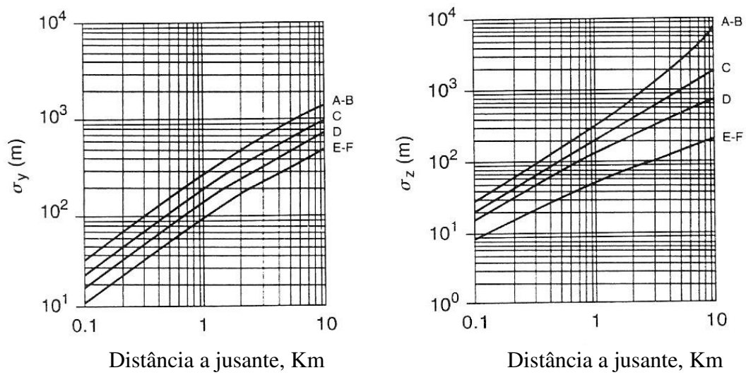
Figura 2.7. Coeficientes de dispersão para o modelo de pluma em área urbana, (CROWL E LOUVAR, 2002)
