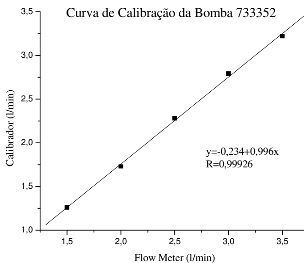
Figura A.11. Curva de calibração da bomba 11.
