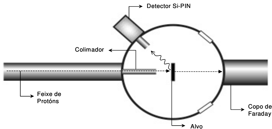
Figura 3.22. Esquema simplificado do arranjo experimental utilizado na técnica de PIXE.
