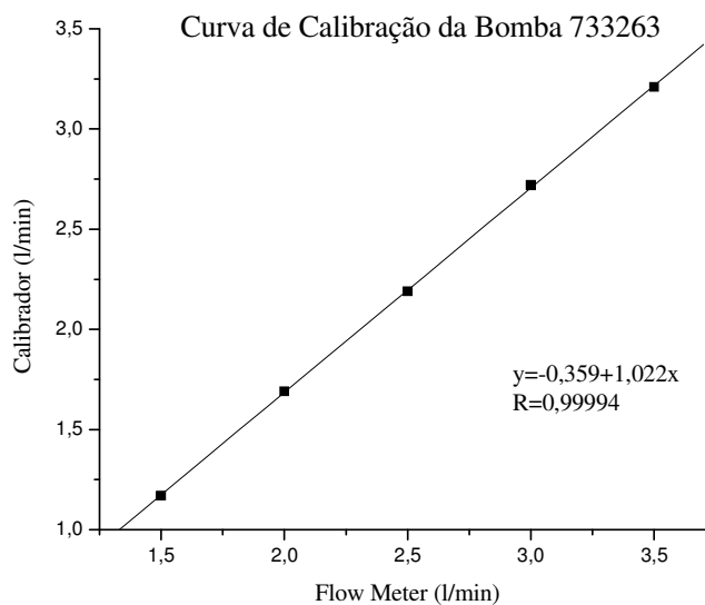
Figura A.7. Curva de calibração da bomba 7.
