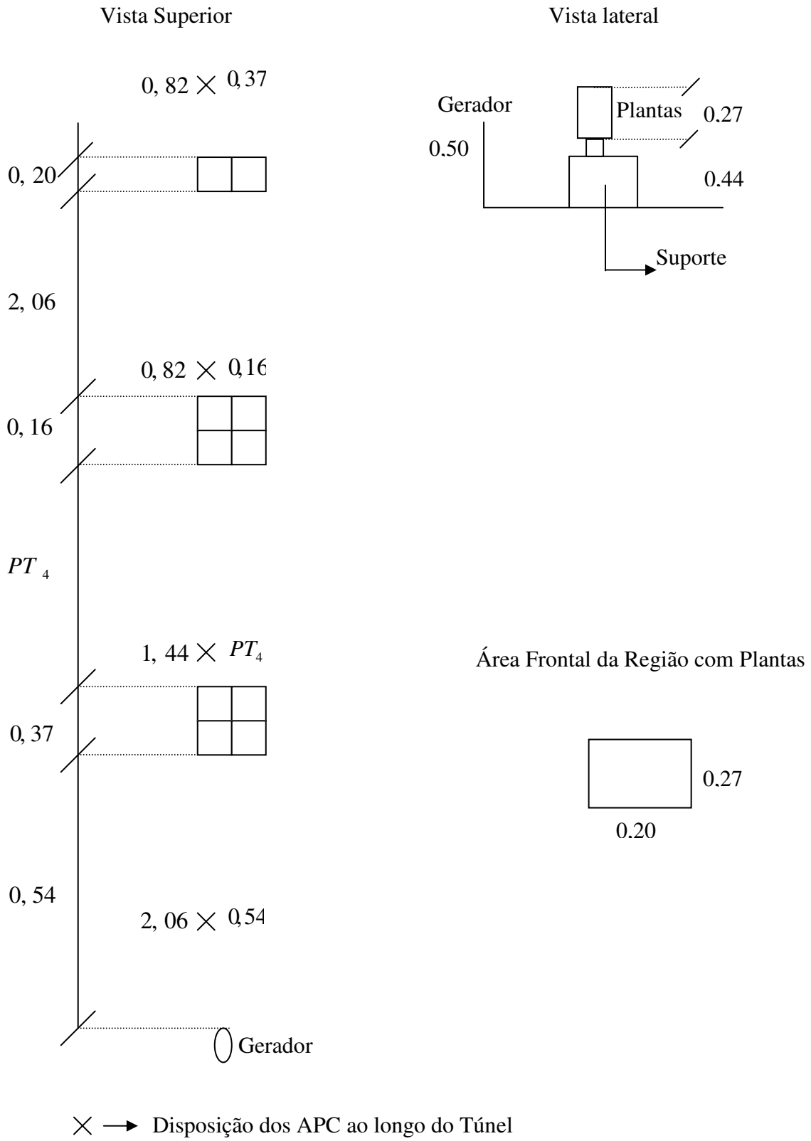
Figura 3.9. Disposição dos vasos de plantas no arranjo II.
