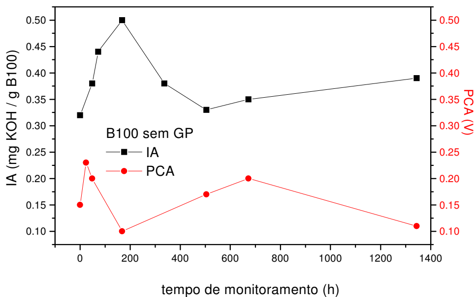
Figura 7: Evolução do índice de acidez ( —●— ) e do potencial de circuito aberto (chapa de aço como eletrodo de trabalho e platina como eletrodo de quase-referência) ( —●— ) para B100 de soja, sem antioxidante, durante 1344 h (8 semanas). Monitoramento a temperatura ambiente.
