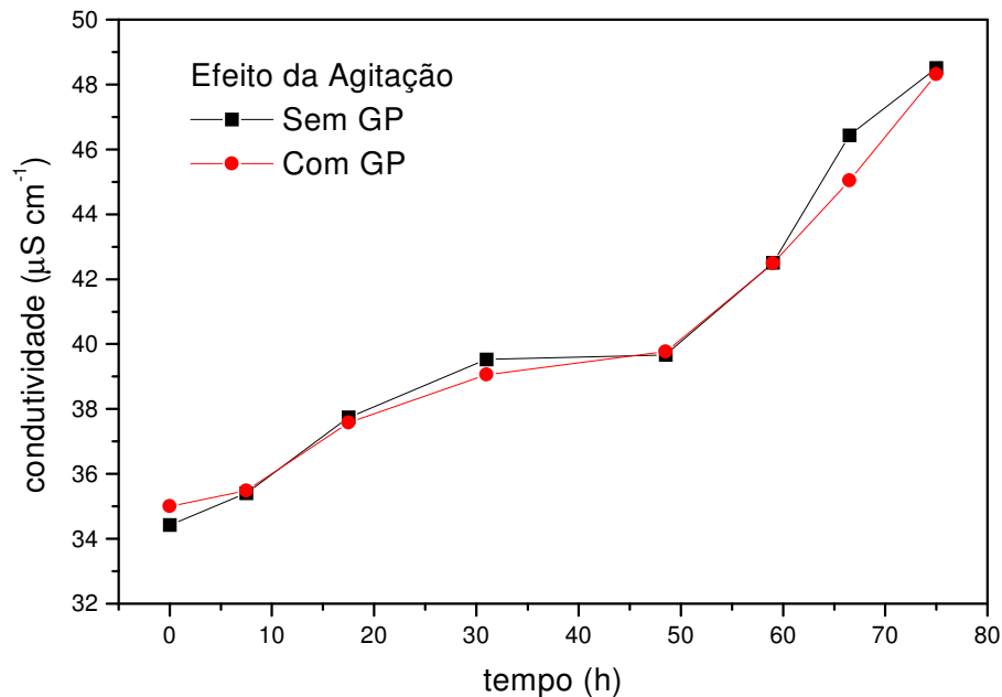
Figura 14: Valores de condutividade ( \mu\text{S cm}^{-1} ) vs tempo de imersão (h) para B100 A sem galato de propila (■) e com 1000 \text{ mg L}^{-1} de galato de propila (●), monitorados por 75 h, sob agitação e na presença de aço carbono ( 6 \text{ cm}^2 de área exposta). Monitoramento a temperatura ambiente.
