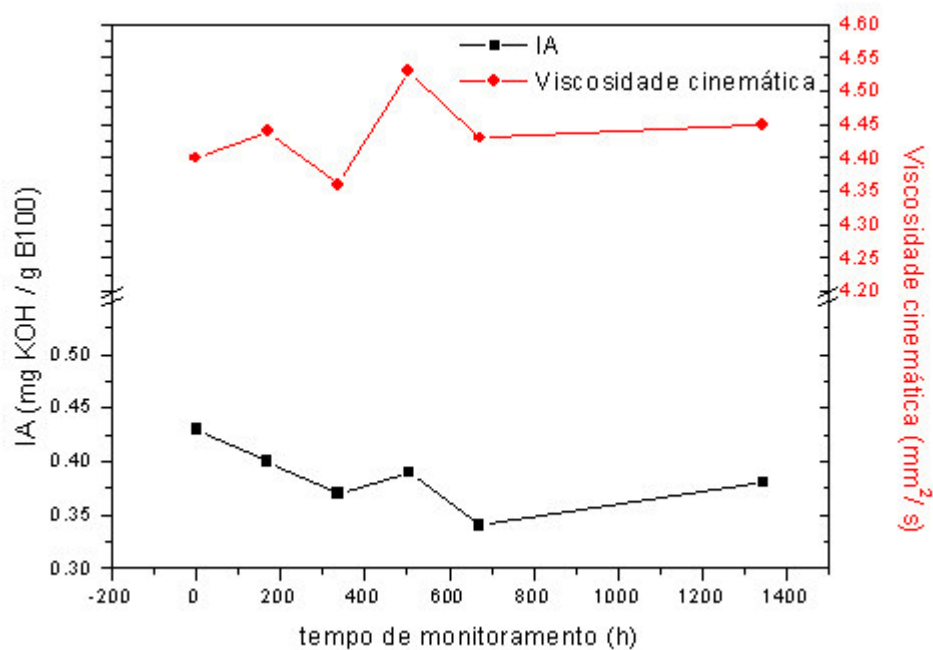
Figura 6: Evolução do índice de acidez (—●—) e da viscosidade cinemática (—●—) para o B100 com 1000 \text{ mg L}^{-1} de galato de propila, durante 1344 h (8 semanas). Monitoramento a temperatura ambiente.
