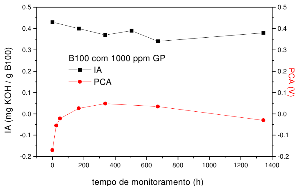
Figura 8: Evolução do índice de acidez ( —●— ) e do potencial de circuito aberto (chapa de aço como eletrodo de trabalho e platina como eletrodo de quase-referência) ( —●— ) para B100 de soja com adição de 1000 mg L -1 de galato de propila como antioxidante, durante 1344 h (8 semanas). Monitoramento a temperatura ambiente.
