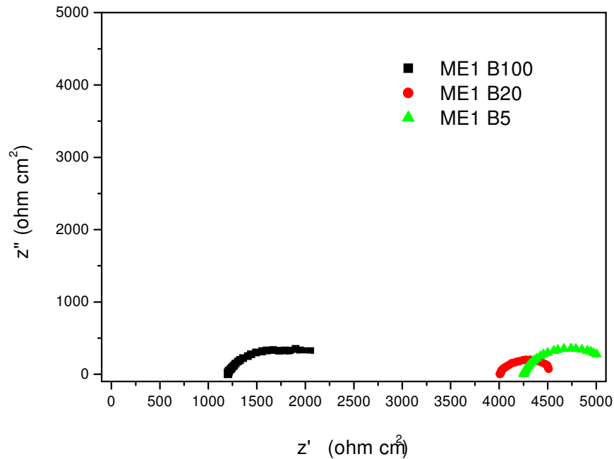
Figura 21. Diagramas de EIE representados em Nyquist para chapas de aço carbono 1020 imersas em: ( ■ )ME1B100,( ● ) ME1 B20 e ( ▲ ) ME1 B5, cujas composições são mostradas na Tabela VII. Eletrodos de platina como contraeletrodo e quase-referência.
