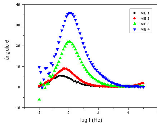
Figura 19. Variação do ângulo \theta vs \log \log f para chapas de aço carbono imersas nas microemulsões: ( ■ )ME1, ( ● ) ME2, ( ▲ ) ME3 e ( ▼ )ME 4, cujas composições são mostradas na Tabela VI. Eletrodos de platina como contraeletrodo e quase-referência.
