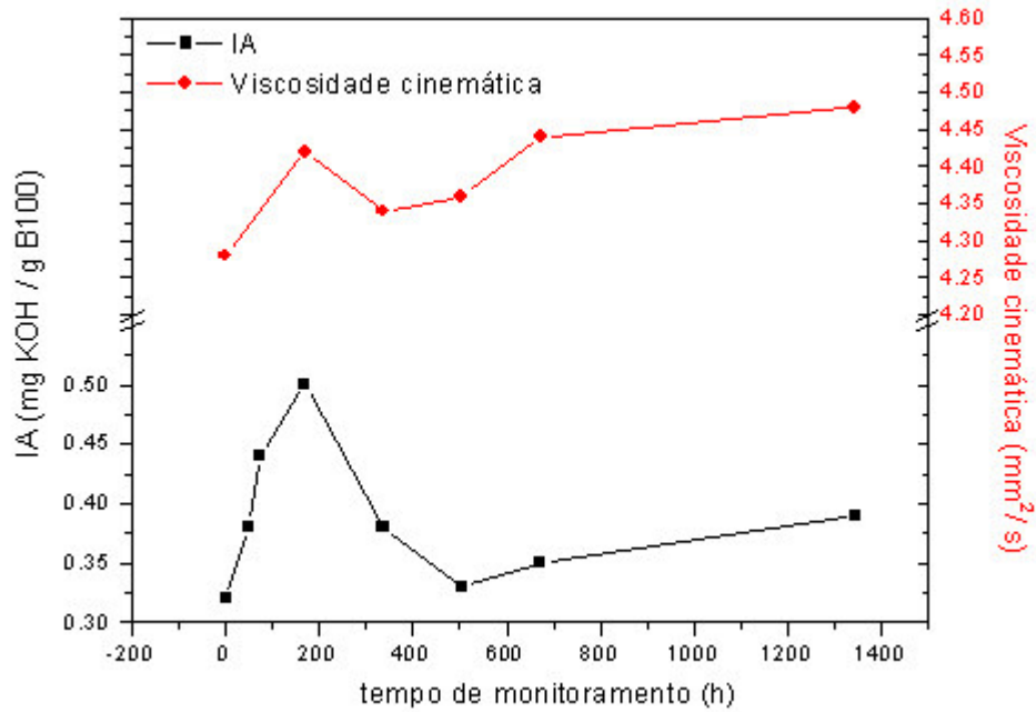
Figura 5: Evolução do índice de acidez (—●—) e da viscosidade cinemática (—●—) para B100, sem adição de antioxidante, durante 1344 h ( 8 semanas). Monitoramento a temperatura ambiente.
