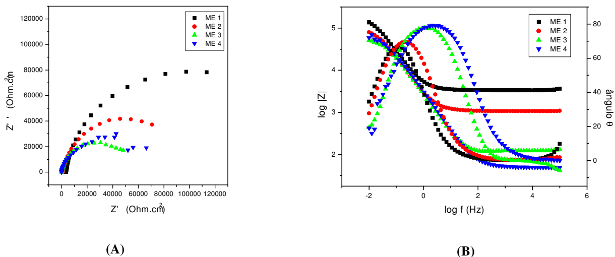
Figura 20. Diagramas de EIE representados em (A) Nyquist e (B) Bode para platina imersa nos meios microemulsionados: ( ■ ) ME1, ( ● ) ME2, ( ▲ ) ME3 e ( ▼ ) ME 4, cujas composições são mostradas na Tabela VI. Eletrodos de platina como contraeletrodo e quase-referência.
