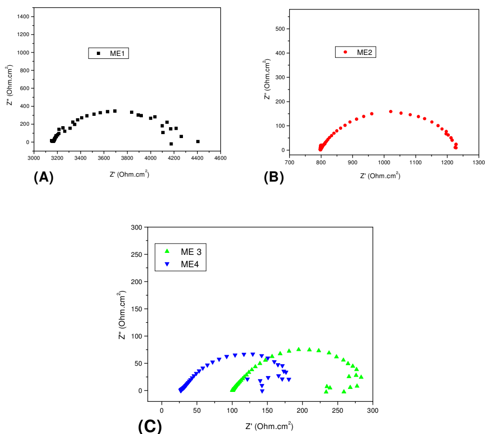
Figura 17. Diagramas de Nyquist para chapas de aço carbono imersas em (A) ME1, (B) ME2 e (C) ME3 e ME 4, cujas composições são mostradas na Tabela VI. Eletrodos de platina como contraeletrodo e quase-referência.
