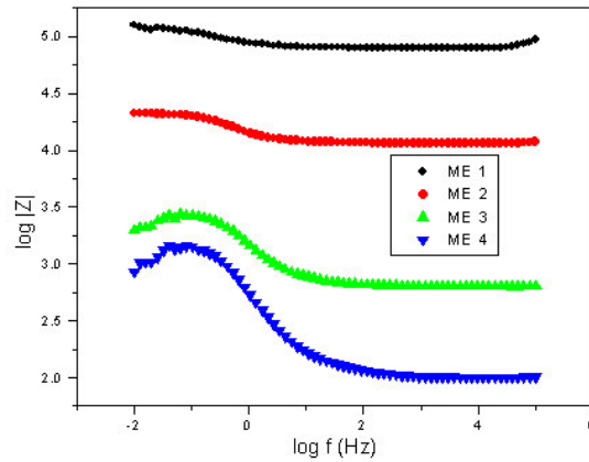
Figura 18. Variação do \log|Z| vs \log f para chapas de aço carbono imersas nas microemulsões: ( ■ )ME1, ( ● ) ME2, ( ▲ ) ME3 e ( ▼ )ME 4, cujas composições são mostradas na Tabela VI. Eletrodos de platina como contraeletrodo e quase-referência.
