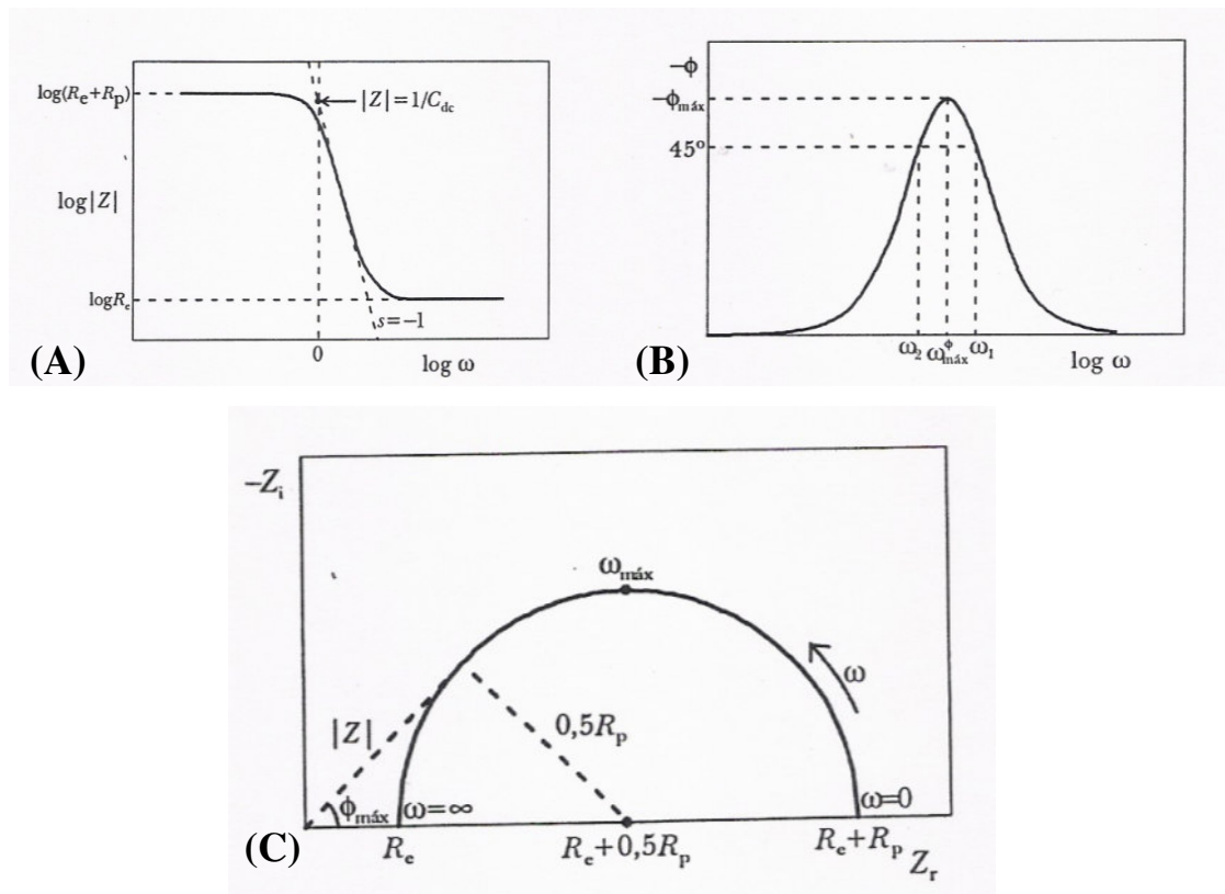
Figura 3. Representação de um gráfico de espectroscopia de impedância eletroquímica, onde: (A) Diagrama de Bode com representação do \log |Z| vs o \log \omega (ou \log f ), (B) Diagrama de Bode com representação do \log |Z| vs ângulo \theta e em (C) Diagrama de Nyquist. 43
