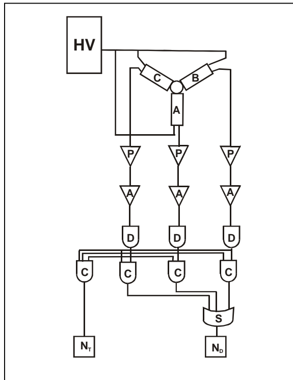
Figura 2.1 Esquema simplificado do Sistema TDCR.
