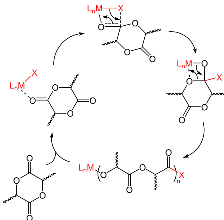
Esquema 10. Ciclo catalítico da polimerização por abertura de anel, onde X = \text{OR}, \text{OSiMe}_3, \text{NR}_2 , e M = \text{Zn, Ca, Mg} .
