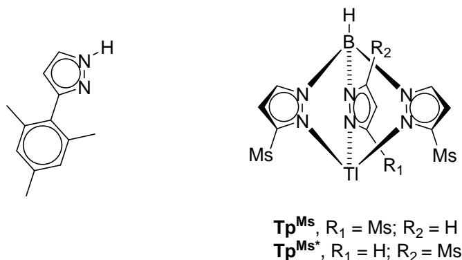
Figura 5. Representação de 3-mesitilpirazol, e seus complexos derivados de Tl(I): \text{Tl}[\text{Tp}^{\text{Ms}}] e \text{Tl}[\text{Tp}^{\text{Ms*}}] .
