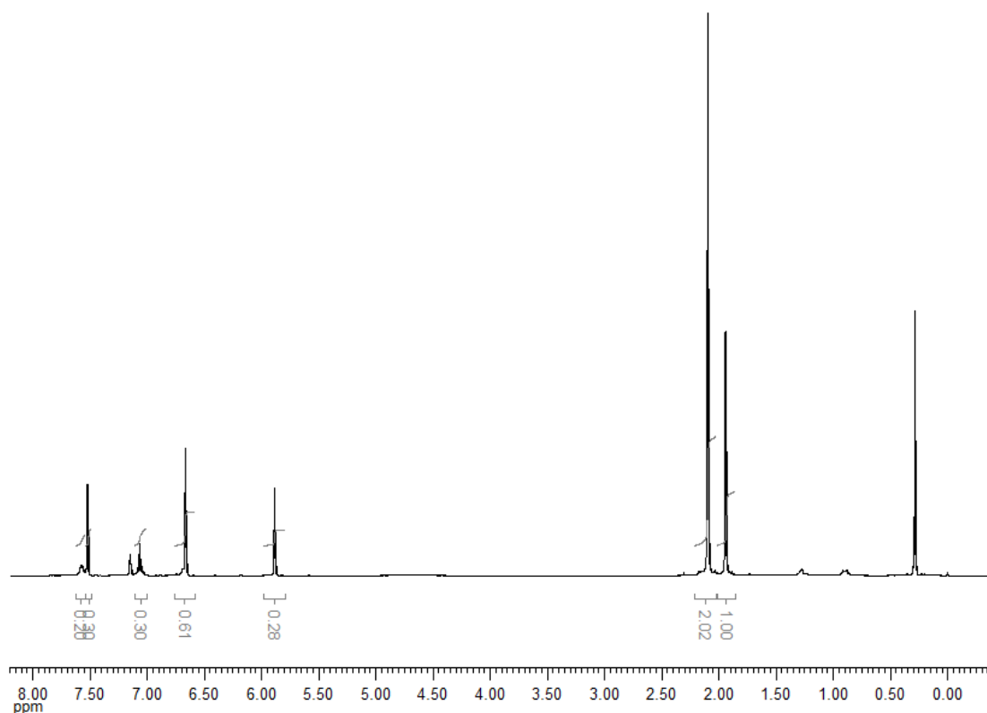
Figura 20. Espectro de RMN de ^1\text{H} do complexo \text{Tp}^{\text{Ms}}\text{ZnOCOPh} ( 6 ) em \text{C}_6\text{D}_6 .
