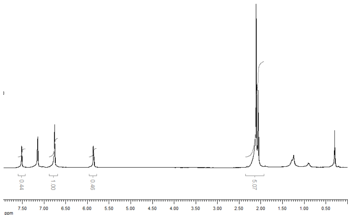
Figura 19. Espectro de RMN de ^1\text{H} do complexo \text{Tp}^{\text{Ms}}\text{ZnOAc} ( 5 ) em \text{C}_6\text{D}_6 .
