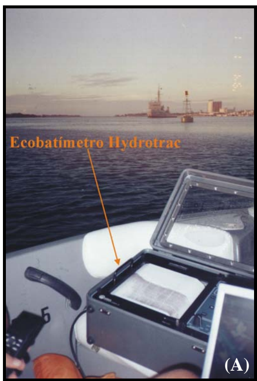
Figura 2.4 - A) Ecobatímetro modelo HYDROTRAC da Odom , operando na frequência de 200 kHz e B) Antena do DGPS Starlink acoplado ao HYDROTRAC (Fotos: Frazão, set. 2001).
