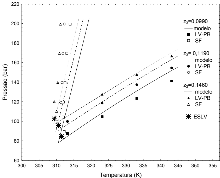
Figura 5.25 Diagrama PT das do equilíbrio SL, LV e SLV para o sistema ternário de \text{CO}_2(1) + etanol(2) + ácido palmítico(3) para as composições globais de ácido palmítico: z_3=0,0990 ; z_3=0,1190 e z_3=0,1460 .
