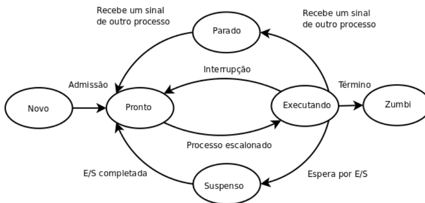
Figura 8.3: Diagrama de estados de um processo
