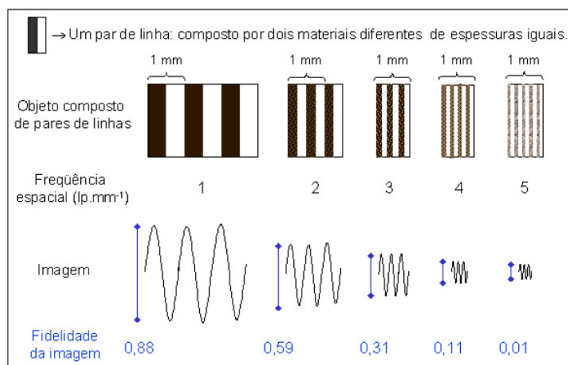
Figura 2.12 Pares de linhas representando a frequência espacial considerada na análise da resolução espacial de imagens de TC.
