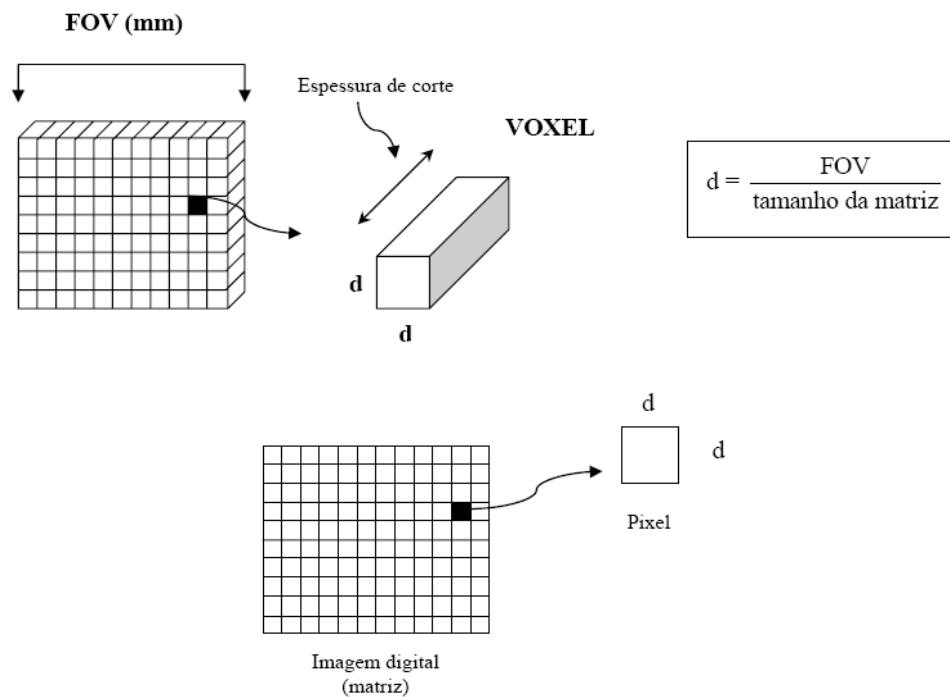
Figura 2.7 Matriz de imagem em TC
