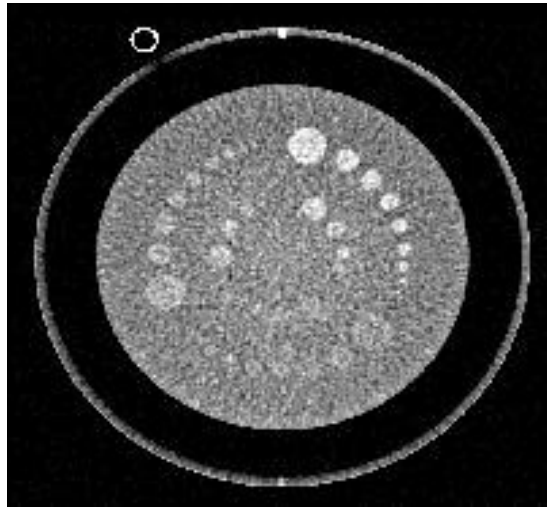
Figura 2.13 Imagem de objeto de teste para avaliação de baixo contraste.
