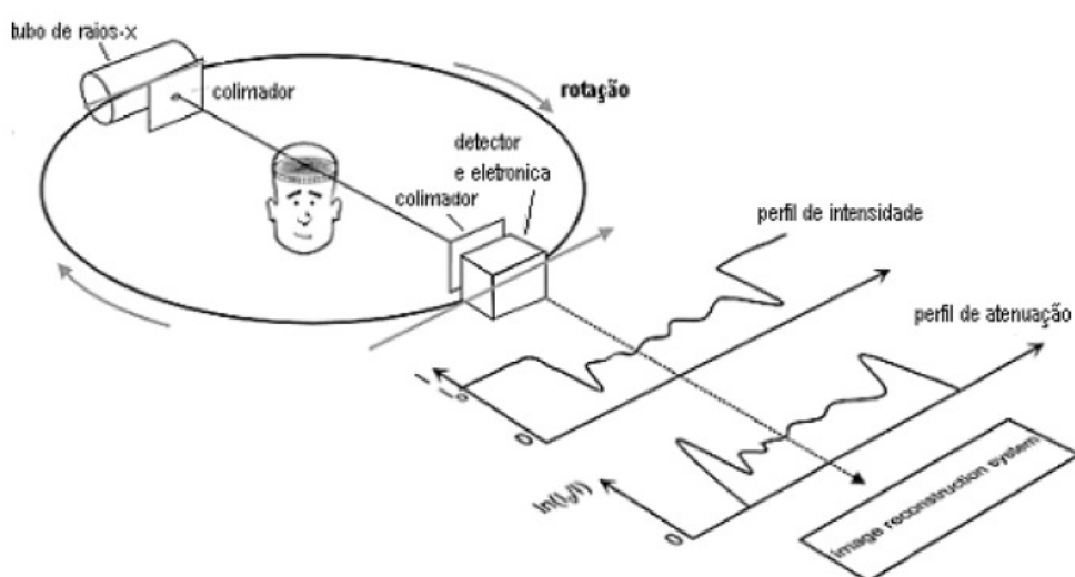
Figura 2.6 Perfil de atenuação e de intensidade para um determinado ângulo.
