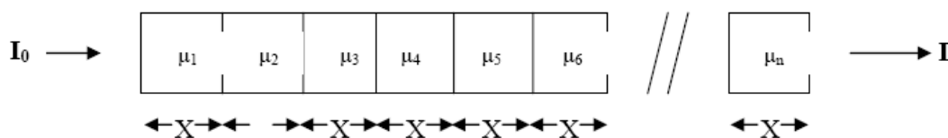
Figura 2.4 Representação da passagem do raio através dos distintos materiais de uma seção de corte.
