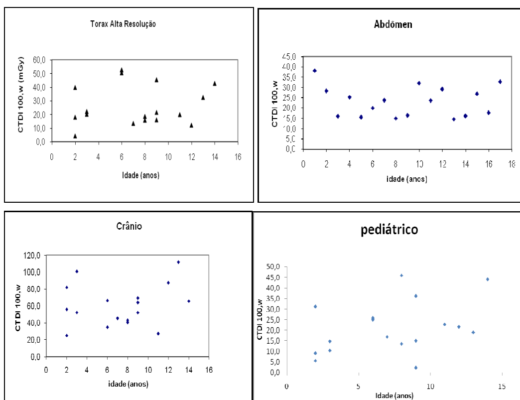
Figura 4.14 Representação da dependência do CTDI_{100,W} em relação a idade do TC para protocolos de: a) tórax; b) abdômen; c) crânio; d) abdômen pediátrico
