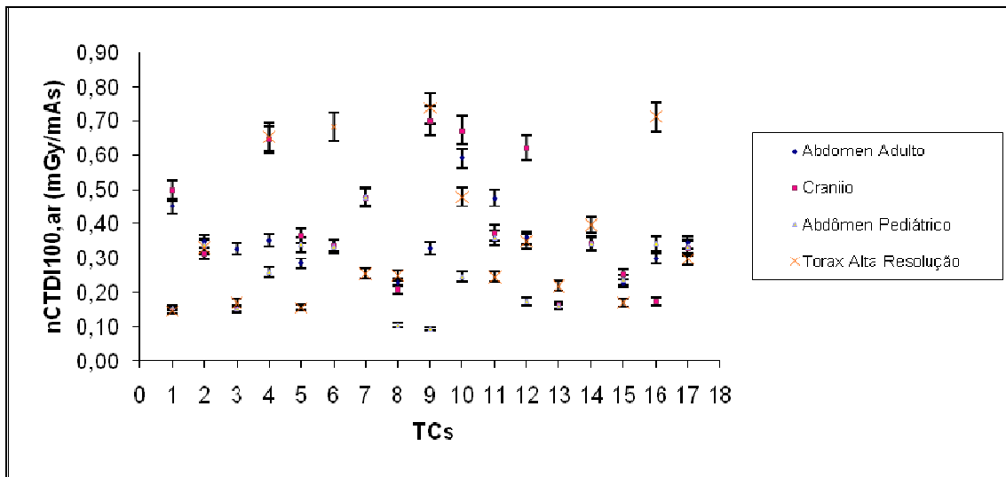
Figura 4.4 Distribuição do CTDI_{100,ar} para os TCs avaliados
