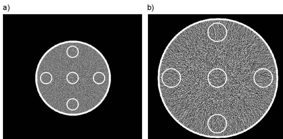
Figura 2.14 imagem do objeto de teste para determinação da homogeneidade do número de TC.
