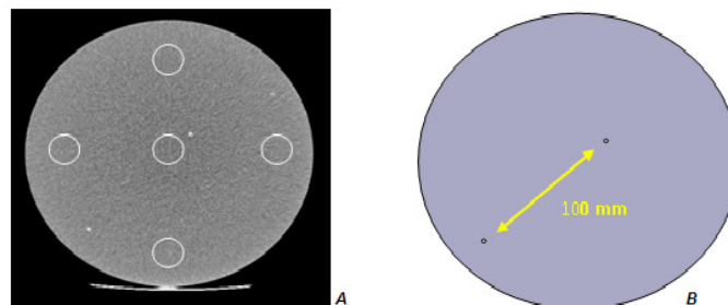
Figuras 3.5 a) Posicionamento dos ROIs para medida de uniformidade do número de CT e exatidão da distância no módulo 3. b) avaliação do indicador de distancia.
