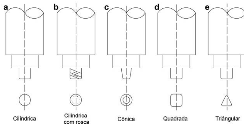
Figura 3.17. Diferentes geometrias de pinos [Elangovan e Balasubramanian., 2007a].
