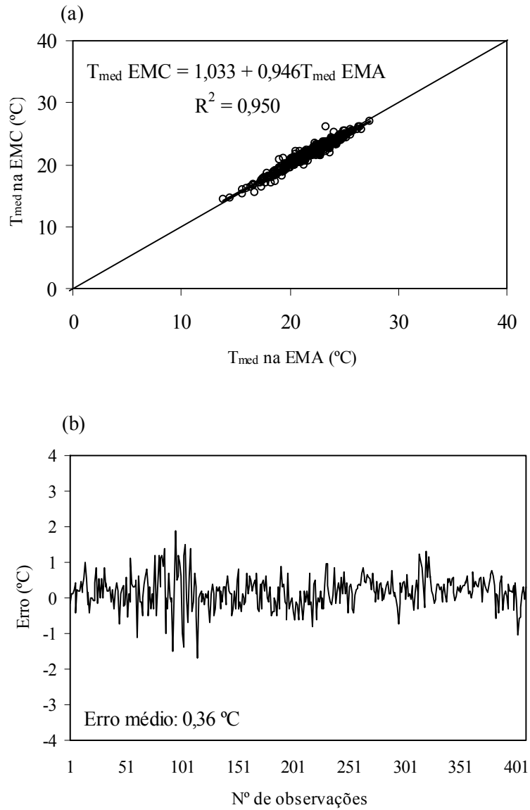
FIGURA 1. Relação entre dados meteorológicos diários: (a) temperatura média do ar ( T_{med} ) e (b) erro da temperatura média do ar, observados na EMA e EMC, entre os anos de 2005 e 2008, em Lavras, MG.
