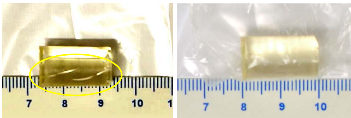
Figura 54 – Fotos da trinca e do xerogel regenerado da amostra 90F1, respectivamente. Em detalhe, as indicações das trincas ocasionadas em 10 segundos de exposição ao ar.
