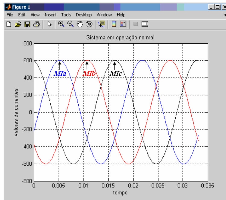
Figura 6.4.1. Correntes trifásicas para o sistema em operação normal.
