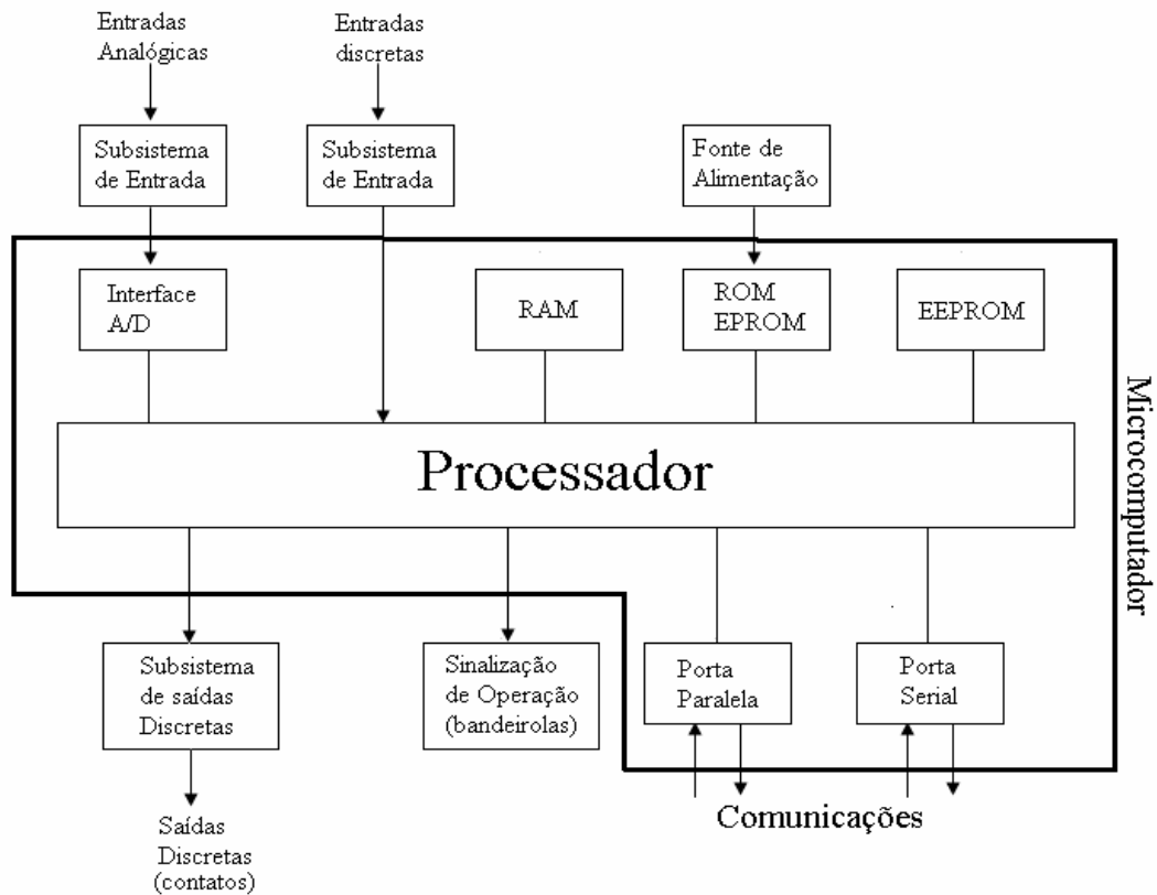
Figura 4.2.5.1. Diagrama de blocos de um relé digital.
