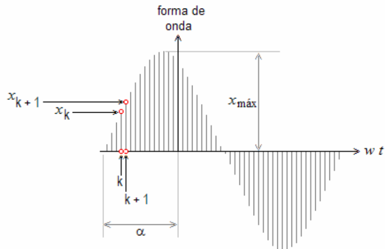
Figura 6.3.1.1. Forma de onda discretizada, considerando-se uma taxa de amostragem m .
