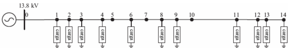
Figura 7.3.1. Diagrama unifilar do alimentador radial.
