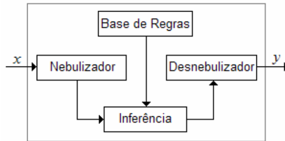
Figura 5.4.1. Sistema fuzzy .
