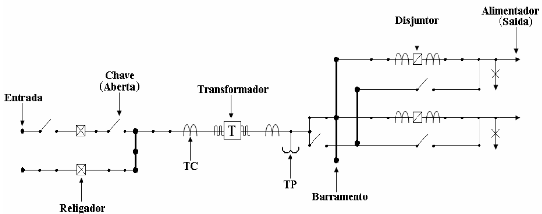
Figura 3.2.1. Subestação e seus componentes.
