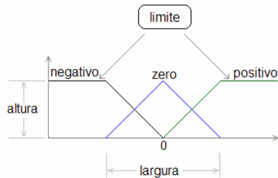
Figura 5.3.1. Função de pertinência triangular.
