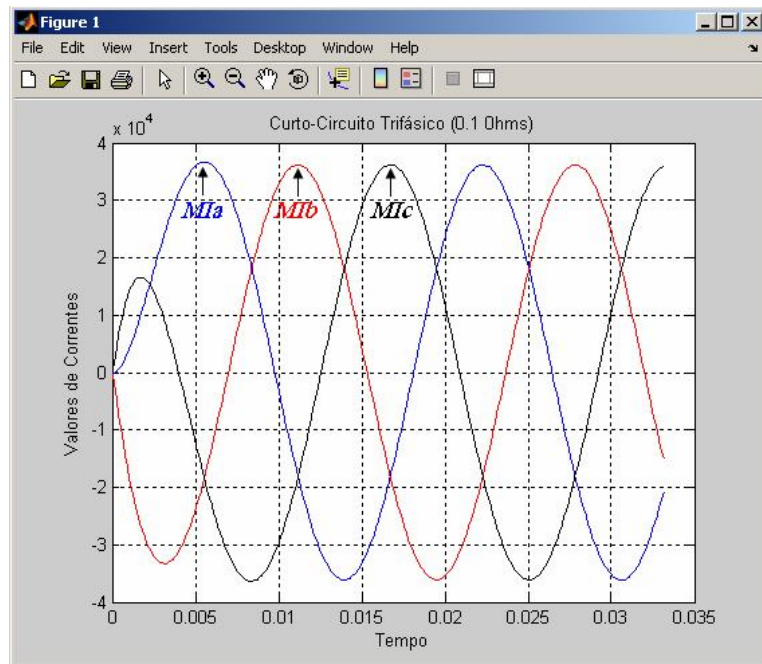
Figura 6.4.2. Correntes associadas a um curto-circuito trifásico.
