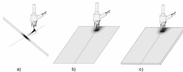
Fig. 3.1 modelos usados na análise de soldas: a) Estado plano de deformações, b) Modelo de Casca, c) Modelo Tridimensional sólido.
