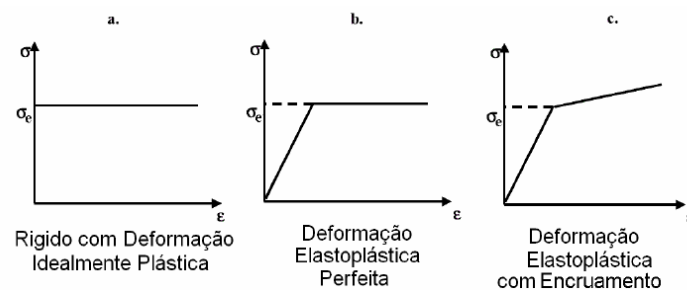
Fig. 5.1 modelos de curvas Tensão x Deformação.
