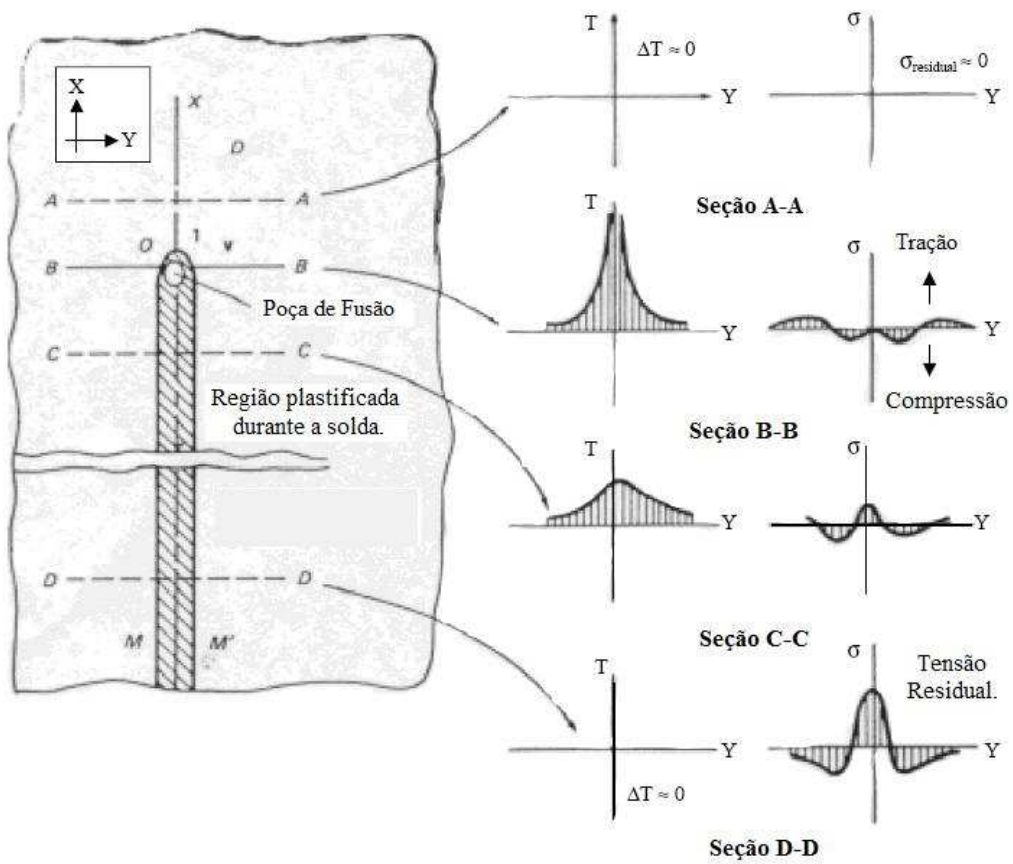
Fig. 2.5 representação esquemática de uma solda de topo.
