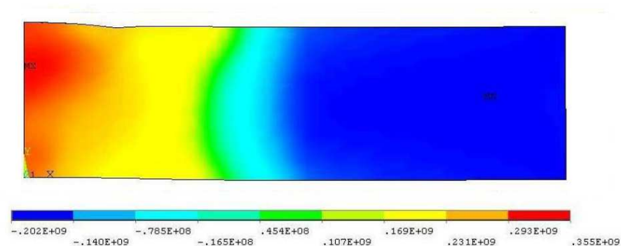
Fig. 6.9 tensões longitudinais, S_{33} , valores em pascais.
