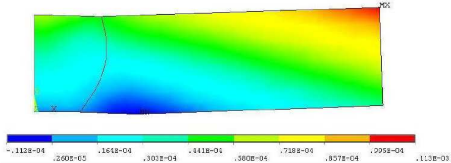
Fig. 6.8 deslocamentos após 2000s, valores em metros.
