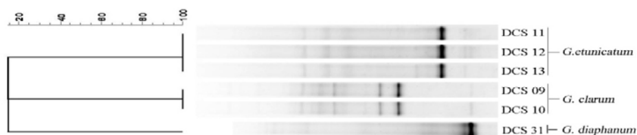
FIGURA 17 Dendrograma mostrando a similaridade entre perfis de bandas de PCR-DGGE de 6 estirpes de Glomus . A escala indica a similaridade entre os perfis de bandas através do Coeficiente de Jaccard (Tol 1.0% -1.0%) (H>0.0% S>0.0%)[0.05 – 100%].
