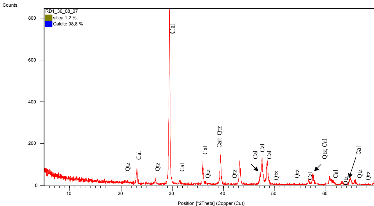
FIGURA 43. Difratograma do calcário RD. Cal: calcita; Qtz; quartzo.
