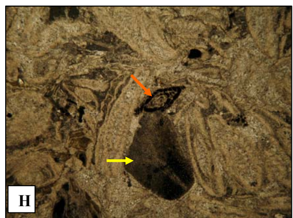
FIGURA 33. Bioclastos dos calcários da Formação La Tampa. A) Foraminíferos: (→) Globigerinoides; (→) nummulítido; (→) Siphogenerinoides sp. B) (→) Algas; (→) carapaça de gasterópodo; (→) globigerinoide. C) (→) alga; (→) carapaça de bivalvo. D) Equinodermo. E) Foram. numulítido. F) (→) carapaça de bivalvo; (→) foraminífero; (→) alga. G) (→) Foram. miliólido. H) (→) foram. numulítido; (→) alga. Aumento 2,5X10.
