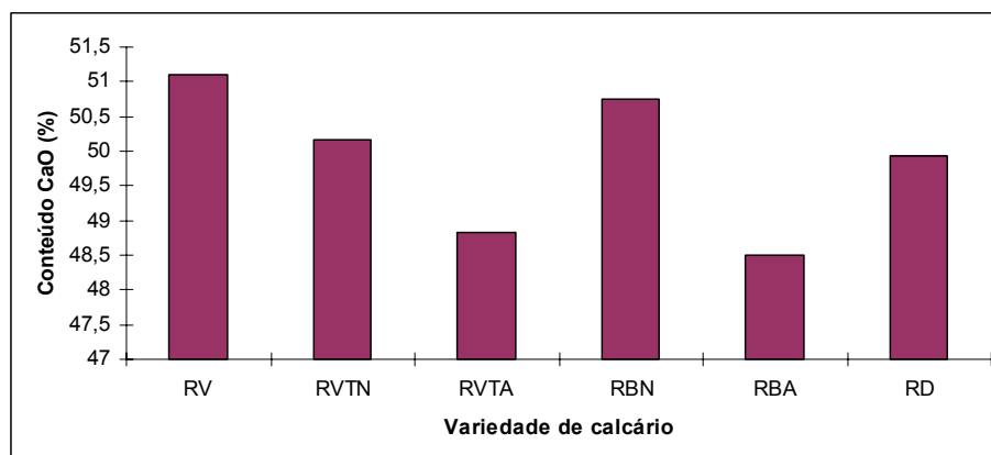
FIGURA 48. Representação gráfica do conteúdo de óxidos de cálcio (CaO) determinado por Espectrometria de Emissão por Plasma ICP
