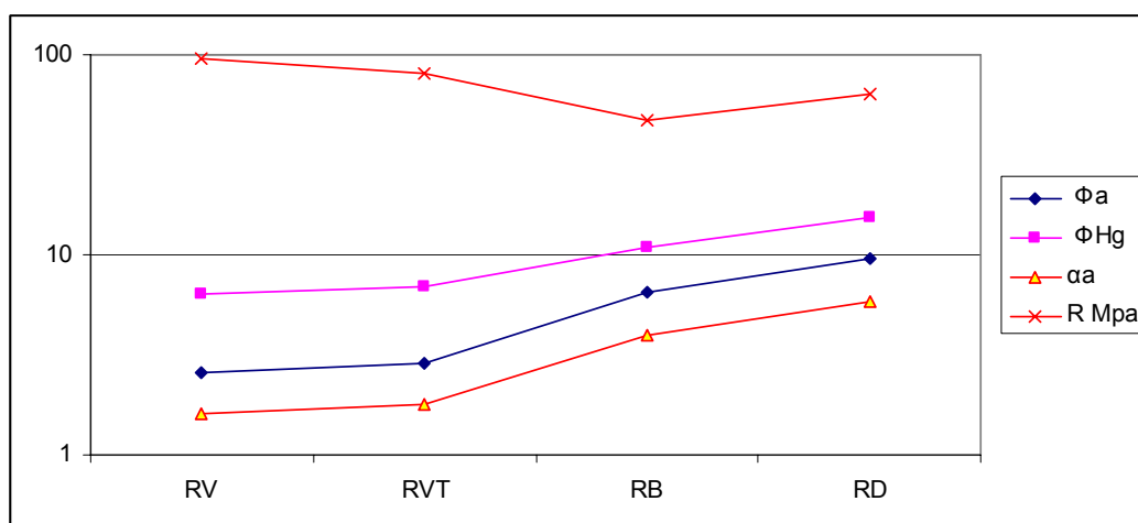
FIGURA 78. Relação entre a resistência à compressão uniaxial (RMPa), porosidade ( \Phi_a e \Phi_{Hg} ) e absorção de água aparente \alpha_a nos calcários pesquisados. (RV: Royal Verde; RVT: Royal Veta; RB: Royal Bronze; RD: Royal Dorado).
