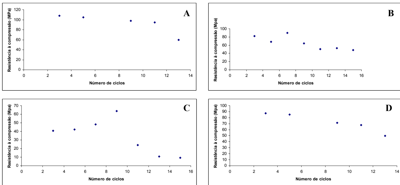
FIGURA 103. Avaliação da resistência aos esforços compressivos após diferente número de ciclos de cristalização de sais. (A) calcário RV; (B) calcário RVT; (C) calcário RB; (D) calcário RD.
