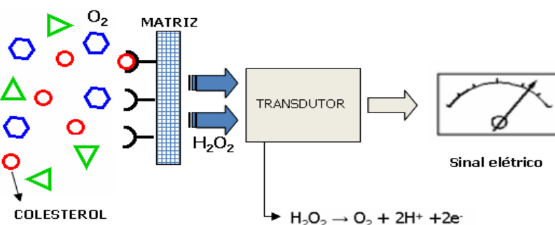
Figura 2.2. Esquema de um biossensor de colesterol.
