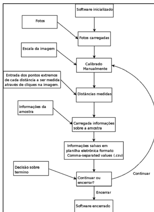
Figura 15 – Fluxograma do funcionamento do software
