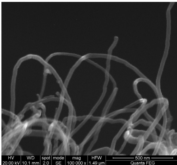
FIGURA 4.55. Micrografia da amostra 2,5\text{Co-NTC-0,5h/25C}_2\text{H}_2\text{-P} de outra região e ampliação de cem mil vezes.
