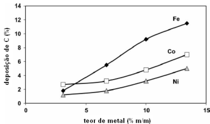
FIGURA 2.25. Atividades catalíticas para Fe, Co e Ni para produção de SWCNTs e DWCNTs a partir de solução de óxidos metálicos – fonte de carbono: CH 4 – tempo de reação: 6 min (GOVINDARAJ et al. , 1999).
