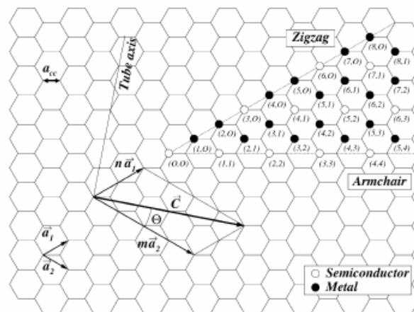
FIGURA 2.6. Definição do vetor quiral C_n , do ângulo quiral \theta e dos vetores unitários a_1 e a_2 em uma camada de grafeno (SEE et al. , 2007).
