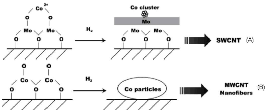
FIGURA 2.24. Mecanismo para a formação de NTCs de parede única em Co-Mo/SiO 2 (A) e mecanismo para a formação de NTCs de paredes múltiplas e nanofibras (B) em Co/SiO 2 (LAMOUROUX et al. , 2007).
