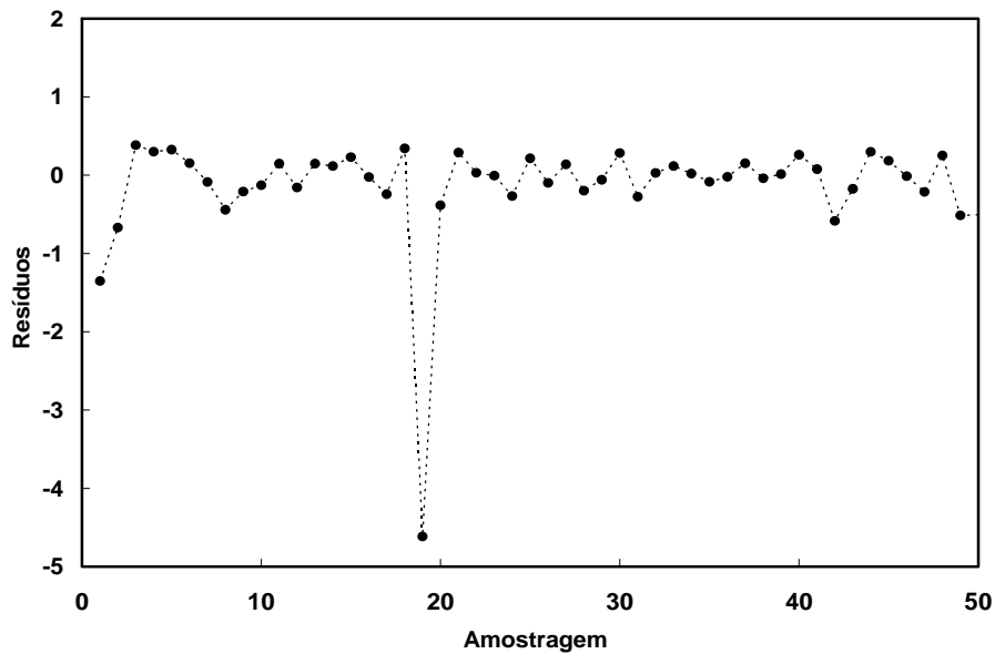
Figura 4.24: Comportamento dos resíduos.
