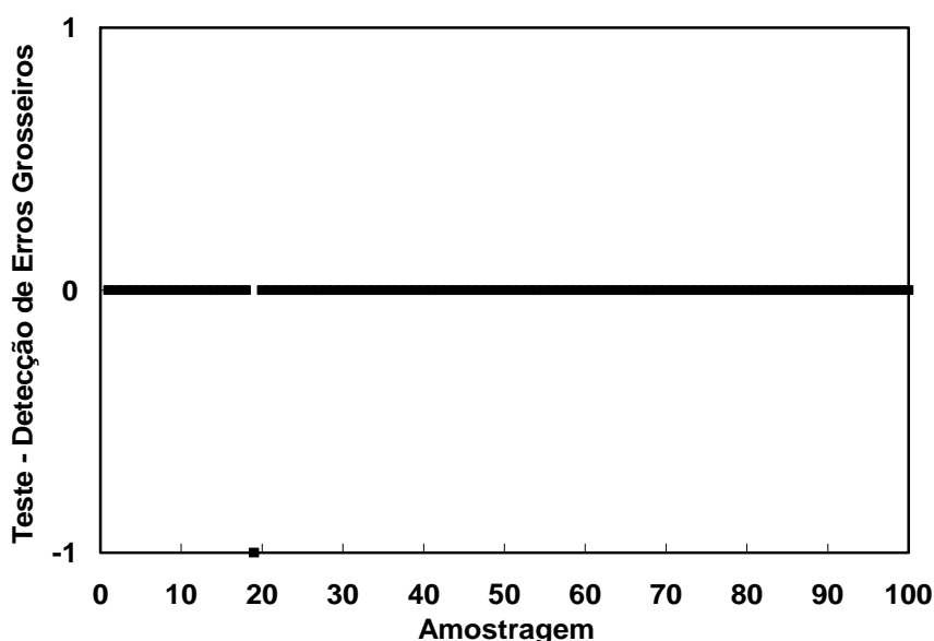
Figura 4.18: Detecção de erros grosseiros nos resíduos.
