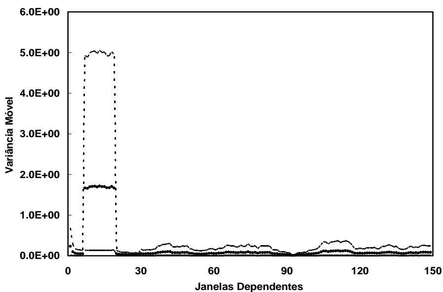
Figura 4.26: Intervalo de confiança (---) e variância móvel (●-).
