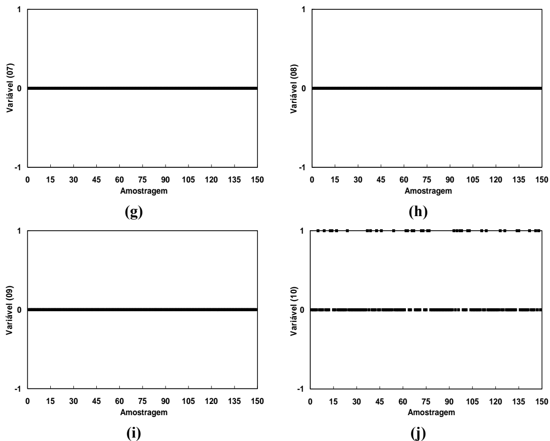
Figura 4.15: Efeito das variáveis independentes sobre a inferência.
