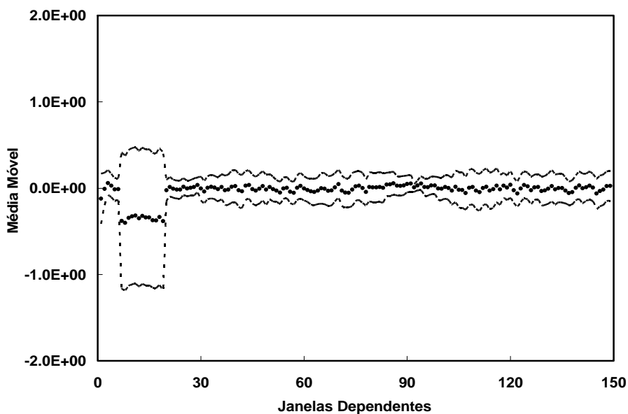
Figura 4.25: Intervalo de confiança (---) e média móvel (●-).
