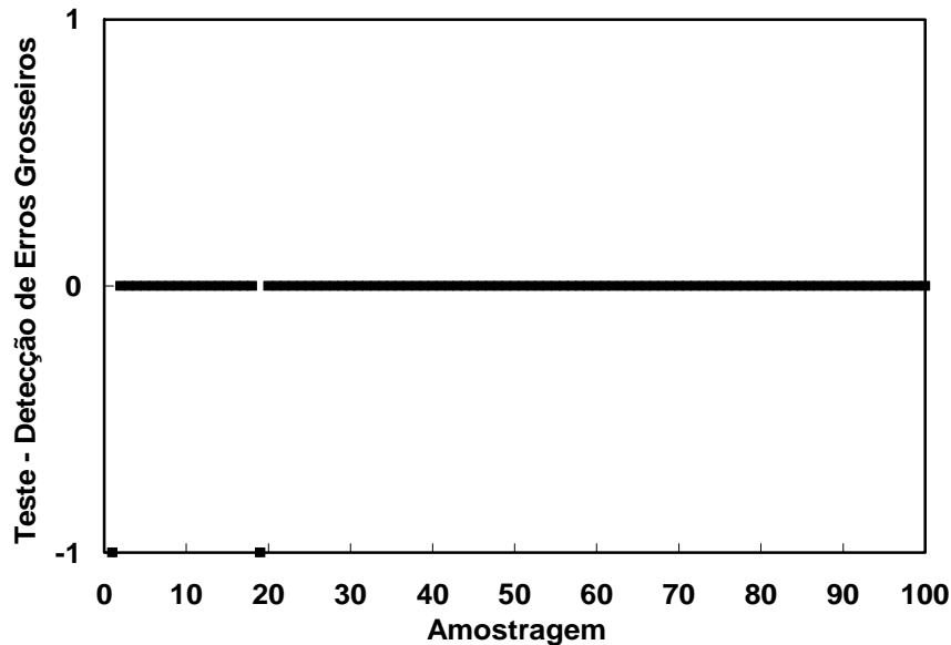
Figura 4.33: Detecção de erros grosseiros nos resíduos.
