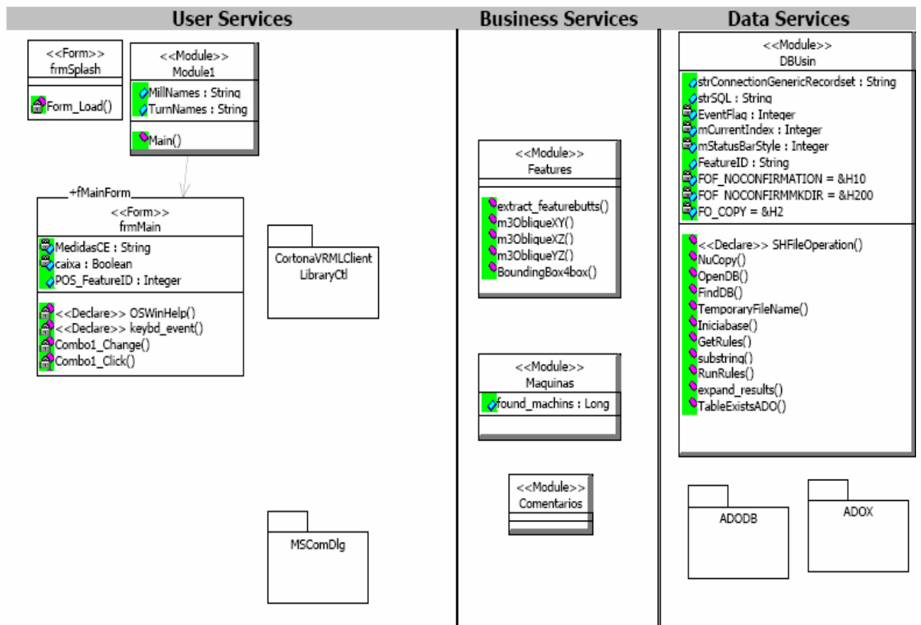
ILUSTRAÇÃO 30 - Diagrama de Classes do UML2, "logical view"
