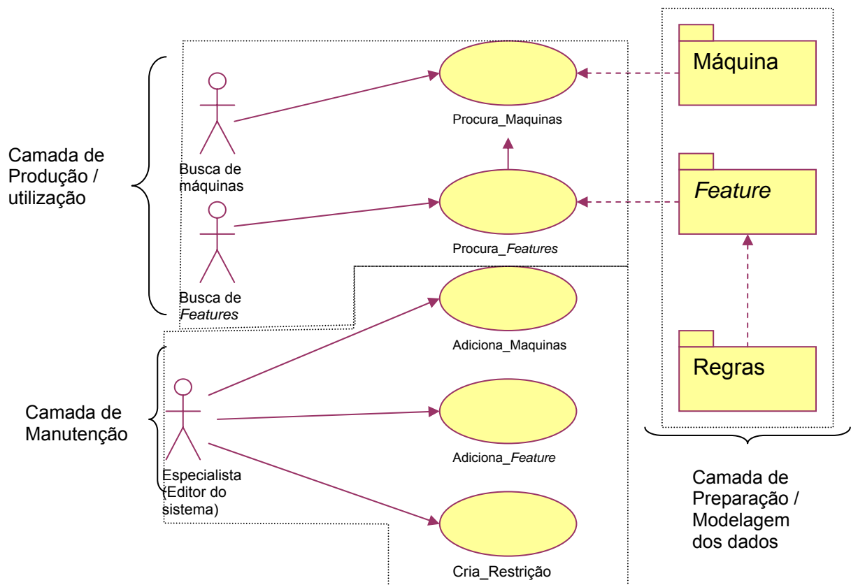
ILUSTRAÇÃO 9 – Esboço do diagrama de caso de uso (UML2) da proposta do sistema
