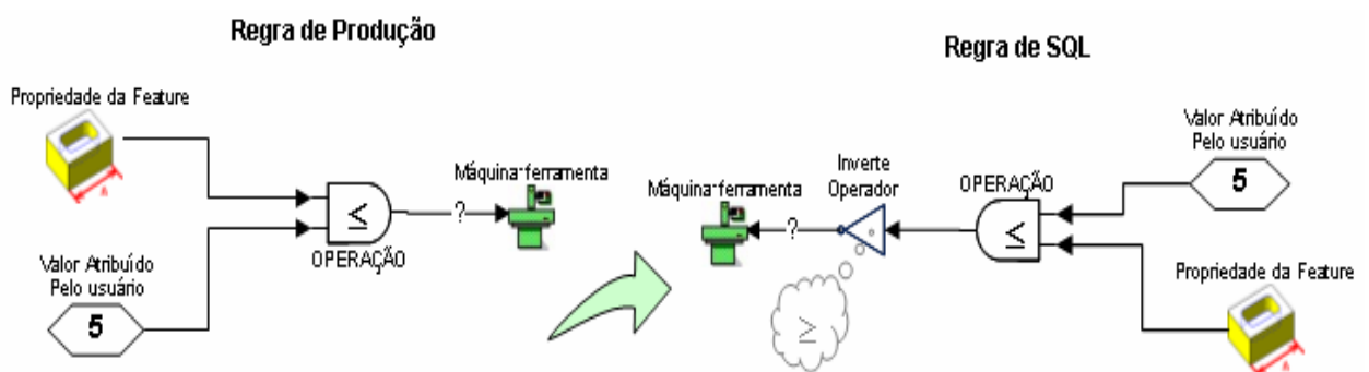
ILUSTRAÇÃO 19 - Conversão de cadeia direta em cadeia reversa.
