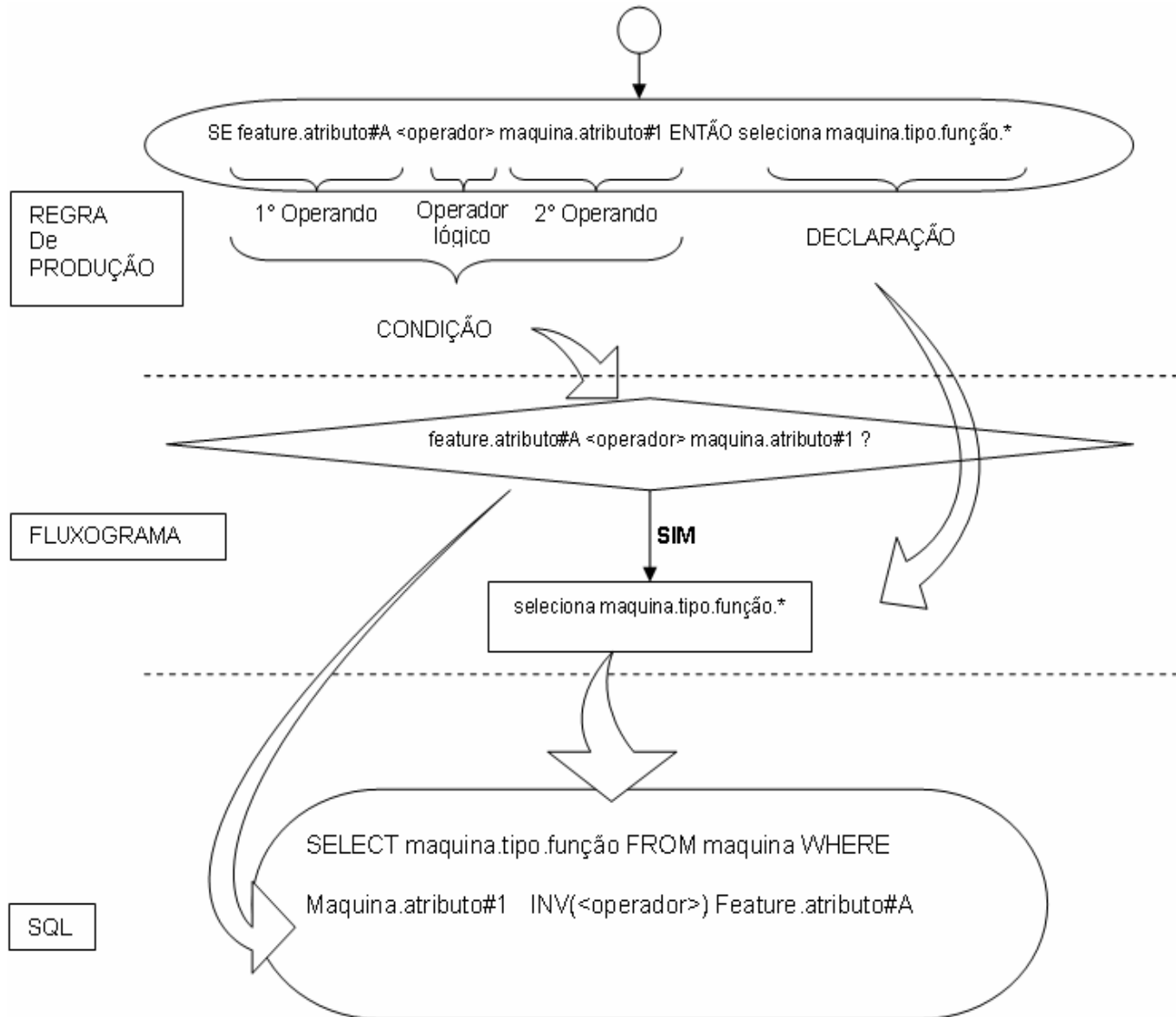
ILUSTRAÇÃO 20 - Detalhe da conversão das regras de cadeia direta em cadeia reversa (SQL)
