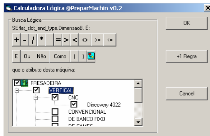
ILUSTRAÇÃO 27 - Cadastro de uma regra ("calculadora lógica")
