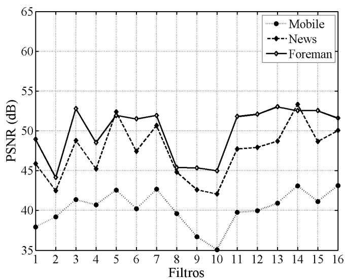
Figura 5.11 Gráfico da PSNR para os vídeos transcodificados.
