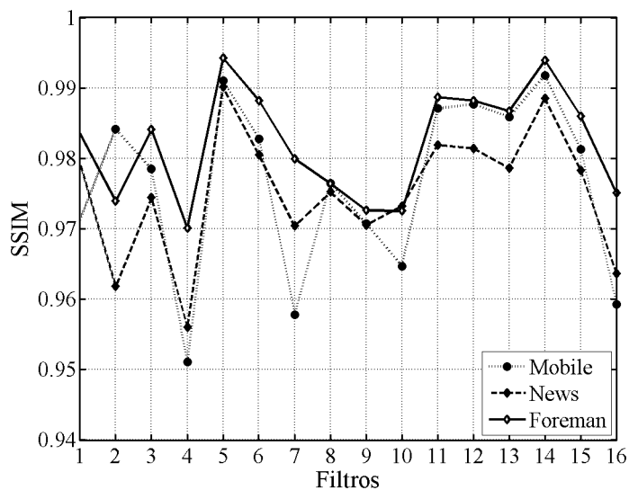
Figura 5.12 Gráfico do SSIM para os vídeos transcodificados.
