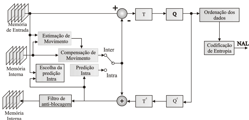
Figura B.1 Estrutura completa de um codificador H.264/AVC.
