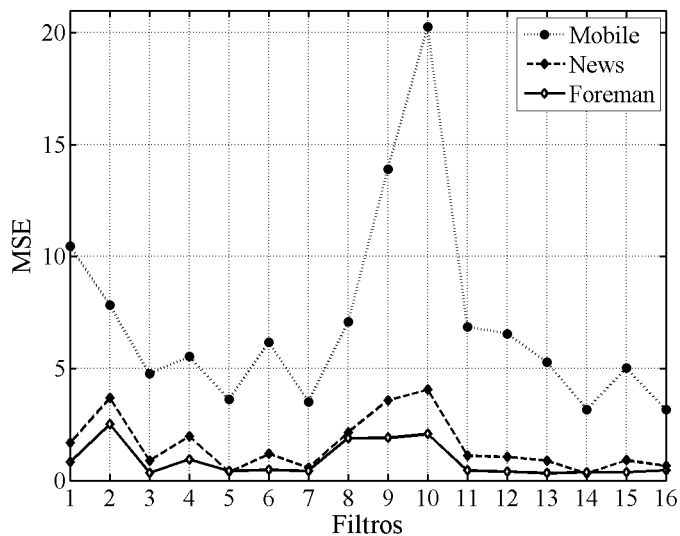
Figura 5.10 Gráfico da MSE para os vídeos transcodificados.
