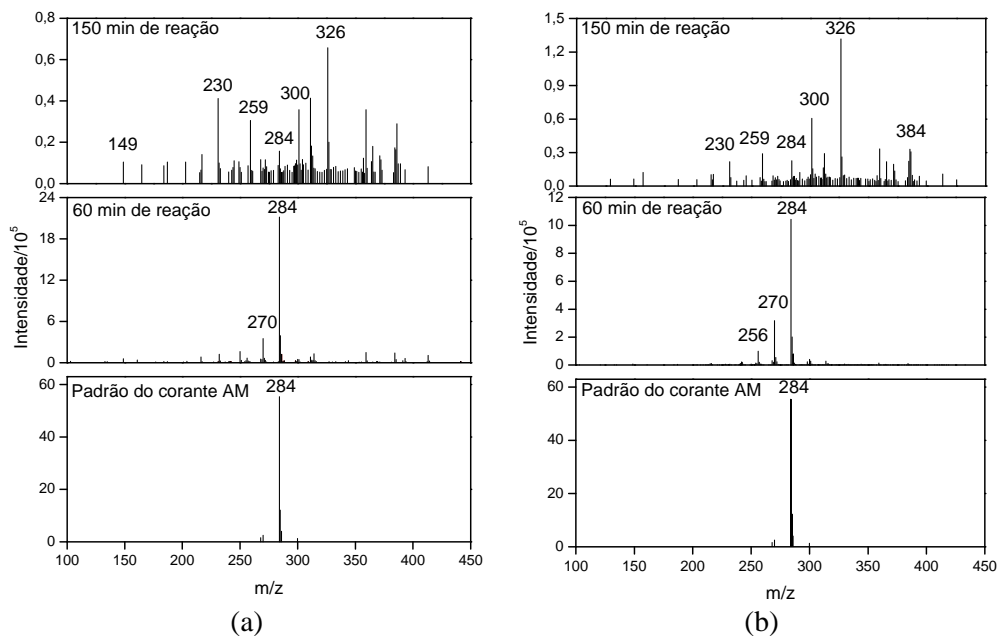
FIGURA 29 – Espectros de massas (ESI-MS) da oxidação do corante AM utilizando-se os catalisadores nióbia//H 2 O 2 30 (a) e nióbia//H 2 O 2 60 (b) na presença de luz UV, em diferentes tempos de reação.
