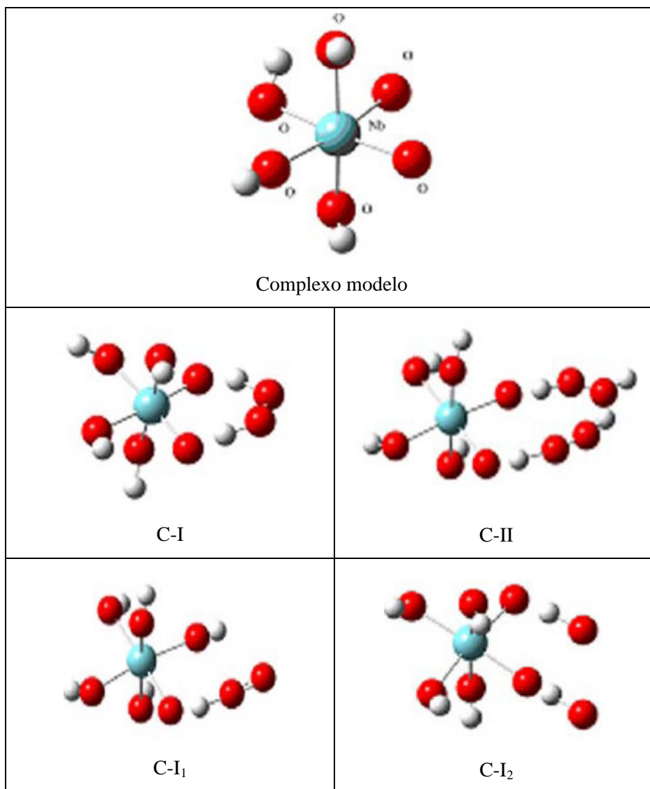
FIGURA 35 – Estruturas modelos para o catalisador (vermelho: oxigênio; azul: nióbio; branco: hidrogênio)
