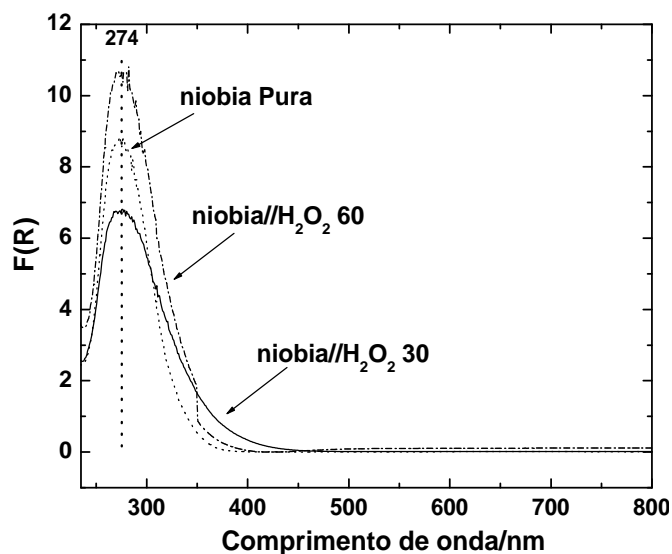
FIGURA 28 – Espectros de UV-vis DRS para nióbia pura, nióbia/H 2 O 2 30 e nióbia/H 2 O 2 60.
