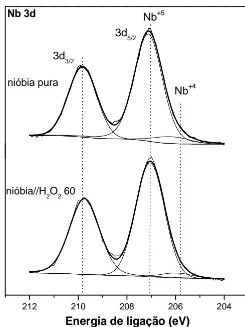
FIGURA 12 – Espectros XPS na região Nb 3d para nióbia pura e nióbia// \text{H}_2\text{O}_2 60.
