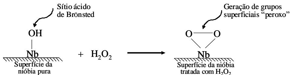
FIGURA 8 – Esquema especulativo da modificação superficial da nióbia após tratamento com peróxido de hidrogênio.
