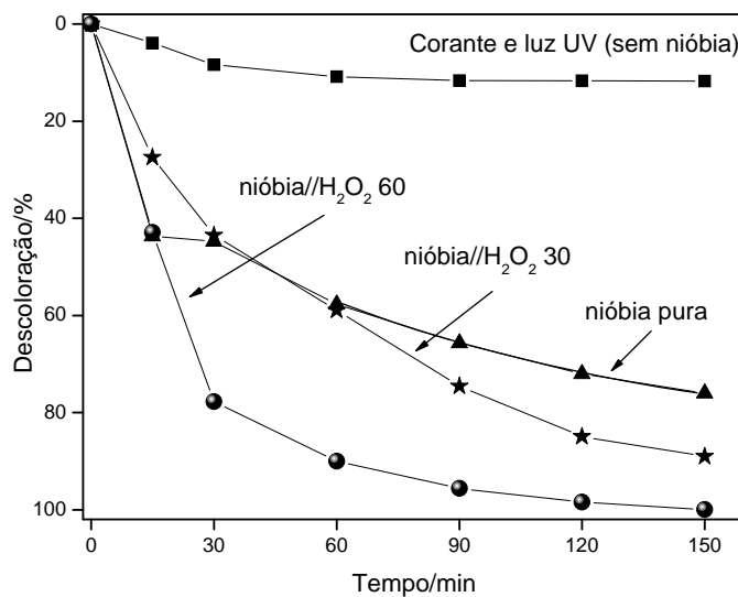
FIGURA 27 – Cinética de oxidação do corante azul de metileno na presença de luz ultravioleta utilizando-se as nióbias como fotocatalisadores.
