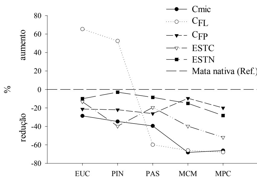
Figura 3. Redução e, ou, aumento nos teores de carbono em diferentes frações orgânicas de Latossolo Vermelho distroférico típico submetido aos sistemas eucalipto (EUC), pinus (PIN), pastagem (PAS), milho no sistema de cultivo mínimo (MCM) e milho no sistema de plantio convencional (MPC), em comparação à mata nativa (MTN). C_{mic} = carbono da biomassa microbiana, C_{FL} = carbono associado à fração leve; C_{FP} = carbono associado à fração pesada (C-areia + C-silte + C-argila); EstC = estoque de C; EstN= estoque de NT. Os dados de EstC e EstN foram obtidos das amostras coletadas na profundidade de 0-0,1 m; os dados dos demais atributos referem-se às amostras da profundidade de 0-0,05 m.
