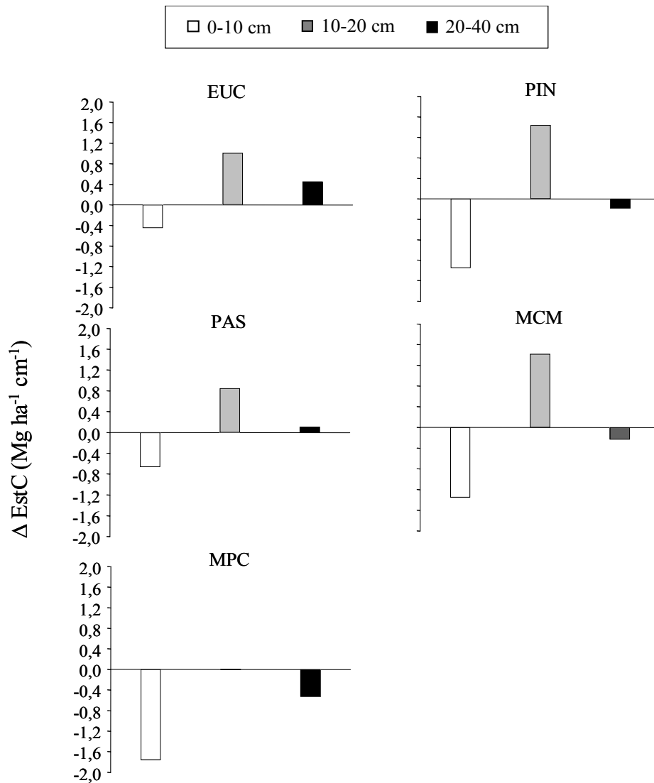
Figura 1. Variação do estoque de carbono ( \Delta \text{EstC} ), nas profundidades de 0-0,1; 0,1-0,2 e 0,2-0,4 m, em relação ao sistema mata nativa (MTN) num Latossolo Vermelho distroférico típico submetido a diferentes sistemas de uso e manejo: EUC: eucalipto; PIN: pinus; PAS: pastagem; MCM: milho no sistema de cultivo mínimo; MPC: milho no sistema de plantio convencional. Valores positivos indicam aumento no estoque de C em relação ao sistema MTN.
