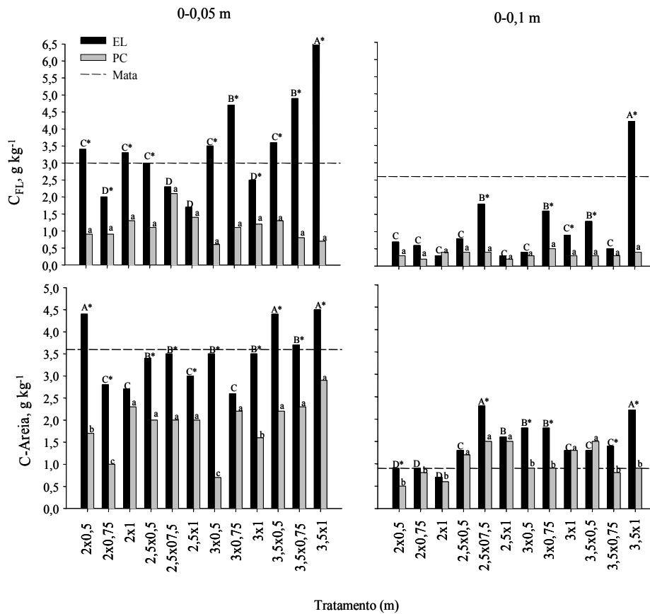
Figura 1A. Teores de carbono nas frações leve ( C_{FL} ) e areia (C-Areia), em diferentes espaçamentos de plantio de cafeeiros implantados em Latossolo Vermelho distroférico típico. EL: amostras coletadas nas entrelinhas; PC: amostras coletadas na projeção das copas. Letras maiúsculas comparam os teores de carbono entre os diferentes espaçamentos de plantio nas amostras coletadas na EL. Letras minúsculas comparam os teores de carbono, entre os diferentes espaçamentos de plantio nas amostras coletadas na PC. Médias seguidas da mesma letra não diferem entre si, pelo teste de Scott-Knott ( p \leq 0,05 ). * Compara os teores de carbono, entre os locais de coleta das amostras de solo (EL e PC) dentro de cada espaçamento. A presença do * designa média estatisticamente superior pelo teste F, a 5% de probabilidade.
