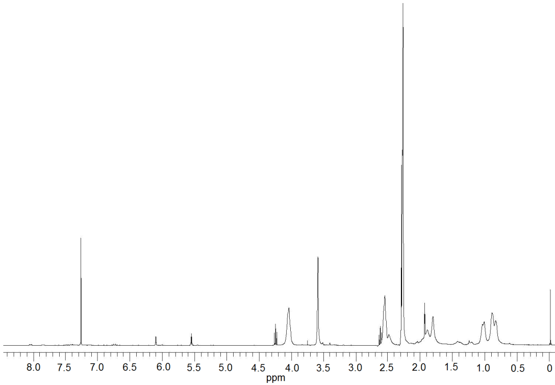
Figura 10 - Espectro de ressonância magnética nuclear de ^1\text{H} de poli(MMA-co-DMAEMA) _3 .
