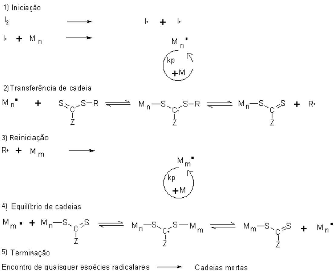
Figura 2 – Esquema da técnica RAFT onde I: iniciador, M: monômero. 25,26
