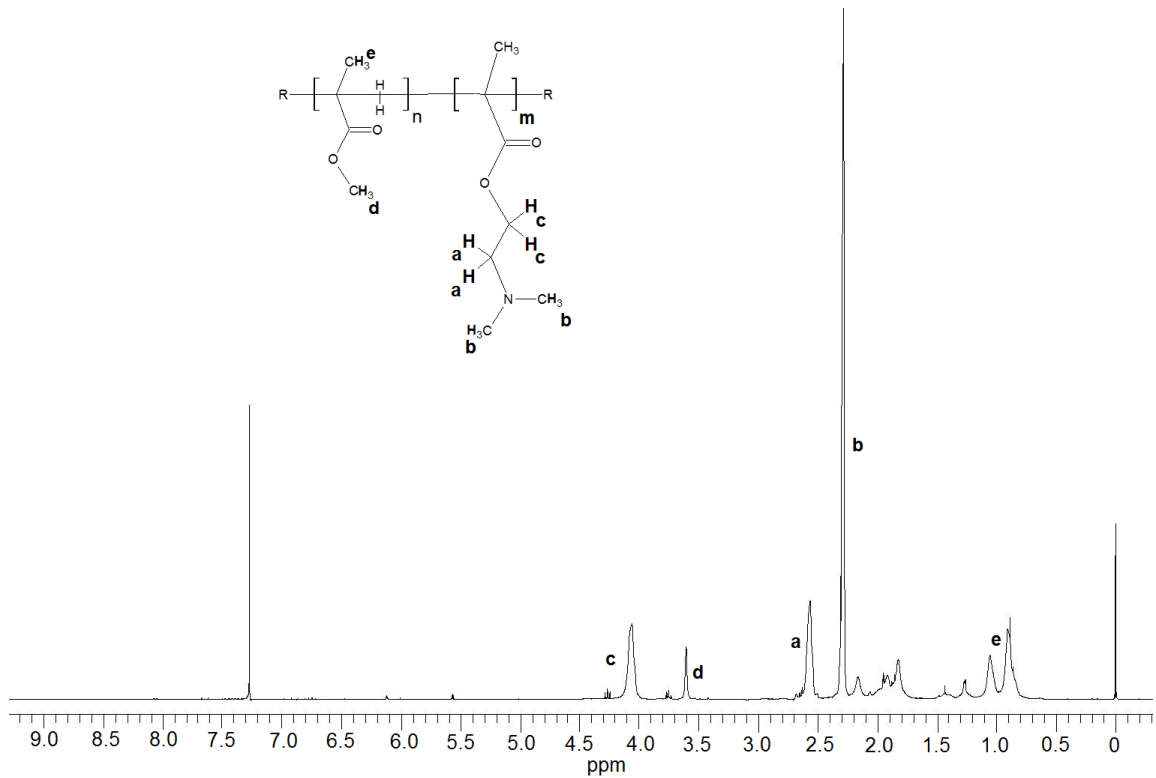
Figura 11 - Espectro de ressonância magnética nuclear de ^1\text{H} de poli(MMA-co-DMAEMA) _4 .
