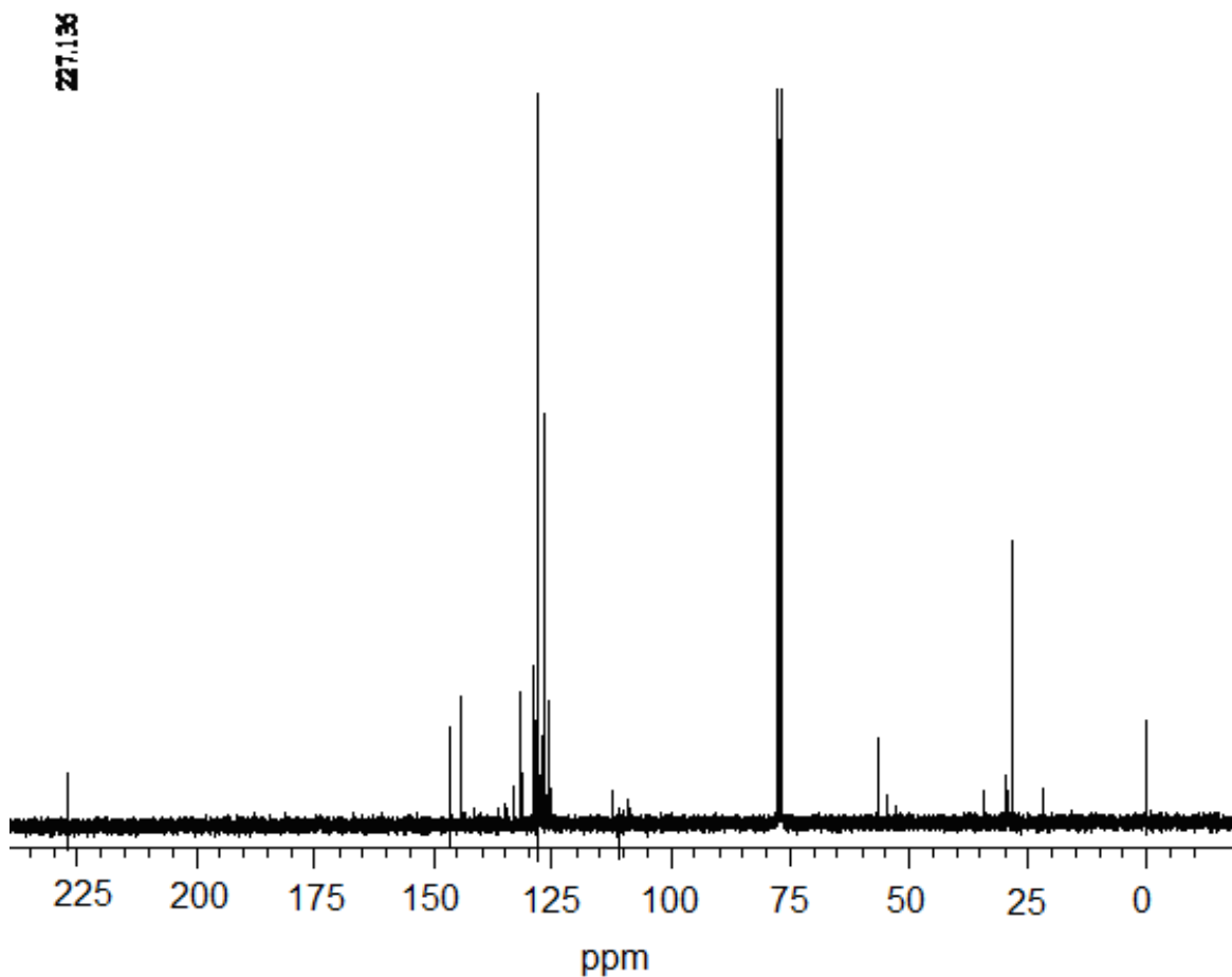
Figura 6 - Espectro de ressonância magnética de ^{13}\text{C} do produto da síntese do DTBC.
