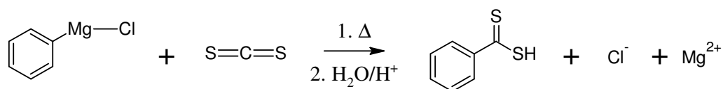
Figura 3 – Esquema da síntese do ácido ditiobenzóico (ADTB).
