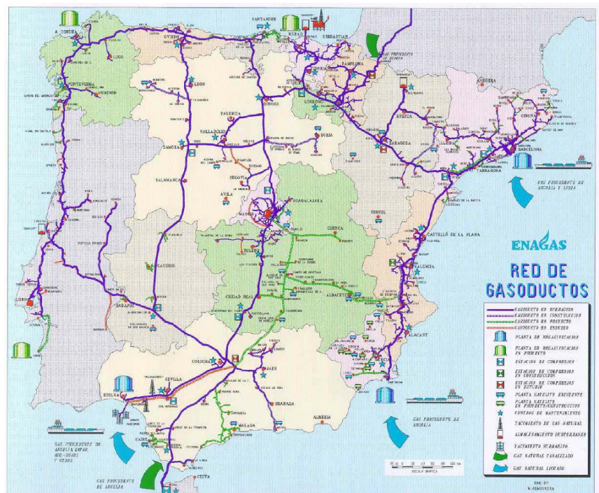
Figura 2.20 - Malha de gasodutos da Espanha e Portugal.
