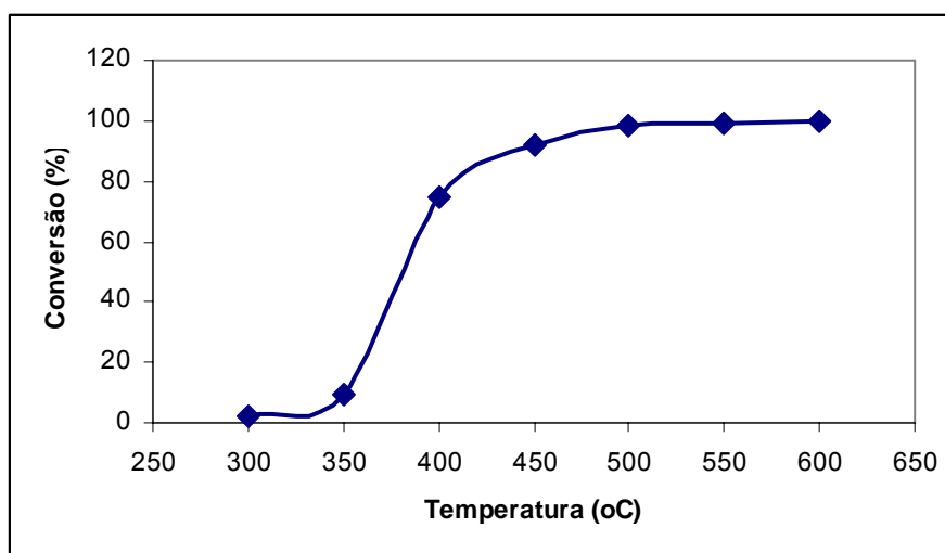
Figura 4.20 Curva de conversão do metano
