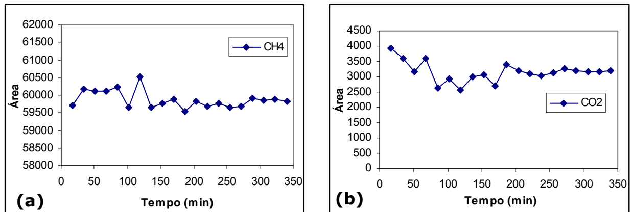
Figura 4.12 - Variação da área dos picos do ensaio a 350°C para (a) metano e (b) CO 2 .
