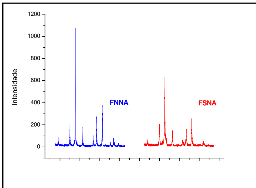
Figura 4.3 - Comparação dos dados de DRX dos produtos sem Calcinação da síntese da ferrita \text{NiFe}_2\text{O}_4 pelas rotas 1 e 2 respectivamente.
