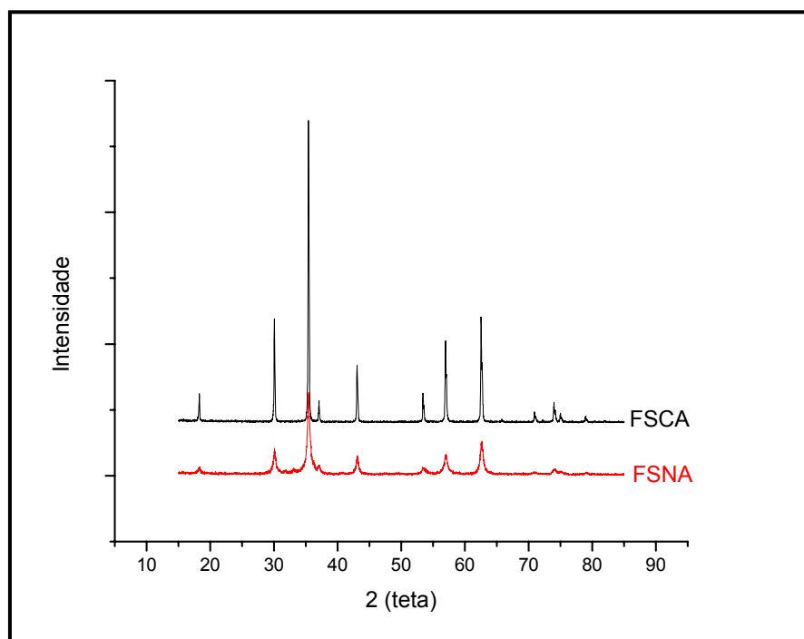
Figura 4.1 - Difração de raios-X para amostras de \text{NiFe}_2\text{O}_4 obtidas da síntese com soluções de nitratos (rota 1)
