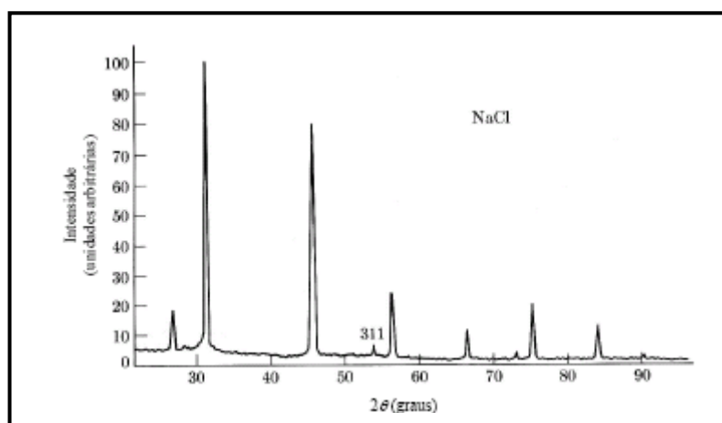
Figura 2.3 Espectro de difração de raios X para uma amostra cristalina de NaCl
