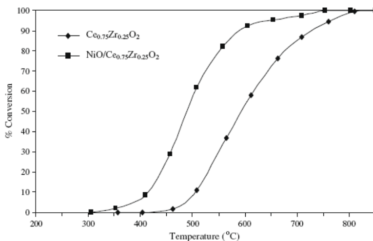
Figura 2.25 - Curva de conversão do metano para Somsak et al
