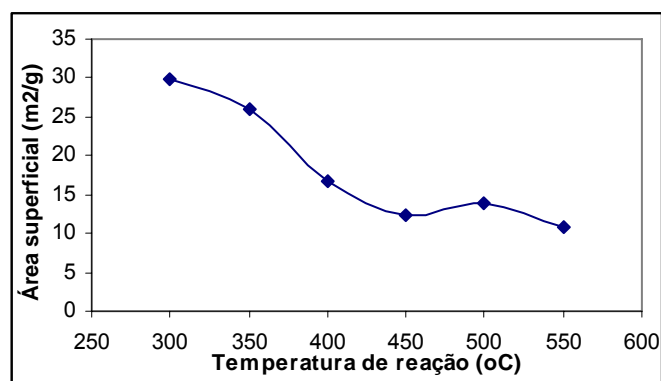
Figura 4.21 - Variação da área superficial com a temperatura de reação
