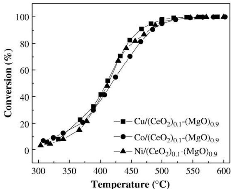
Figura 2.26 - Conversão do metano para Yongxin et al
