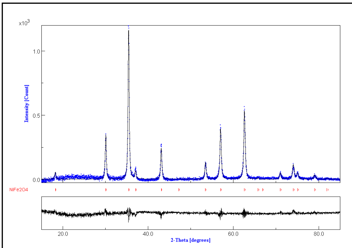
Figura 4.8 - Ajustamento do padrão da ferrita de níquel ao difratograma da amostra sintetizada.
