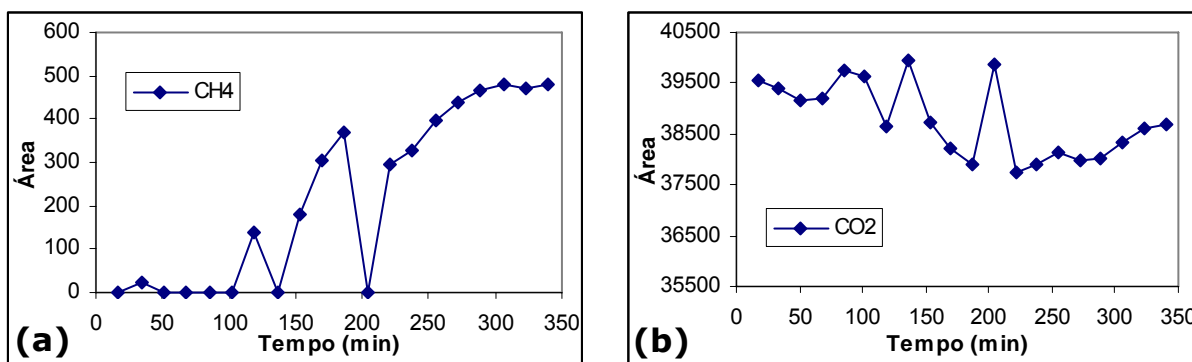
Figura 4.18 - Variação da área dos picos do ensaio a 550°C para (a) metano e (b) CO 2 .
