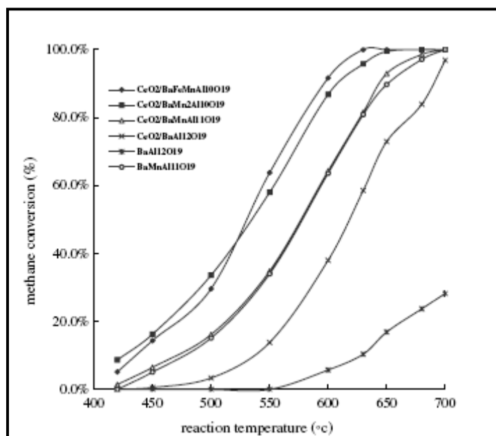
Figura 2.30- Curva de conversão do metano Shunqing e Xiaolai
