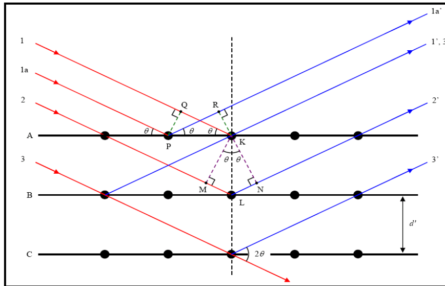
Figura 2.4 - Ilustração para derivação da expressão da lei de Bragg
