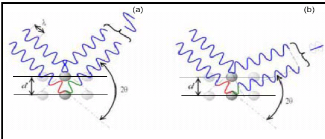
Figura 2.5 - a) Representação da reflexão construtiva e b) reflexão destrutiva.
