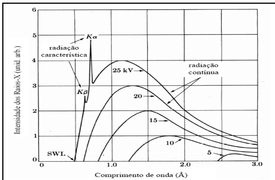
Figura 2.2 Espectro de comprimento de ondas de emissões de raios X
