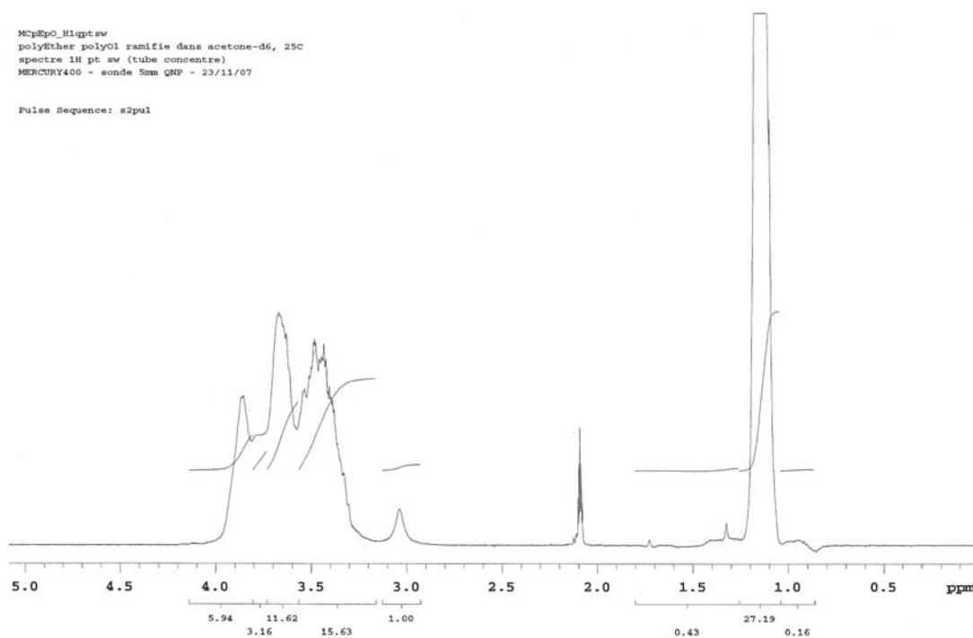
Figura 20 - Espectro de RMN de ^1\text{H} a 400 MHz do polioli poliéter Lupranol ® 3323 em Acetona.
