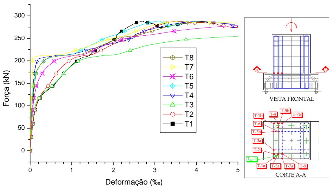
Figura 4.12: Curva força aplicada versus deformação nas armaduras verticais principais e secundárias - Modelo IL5
