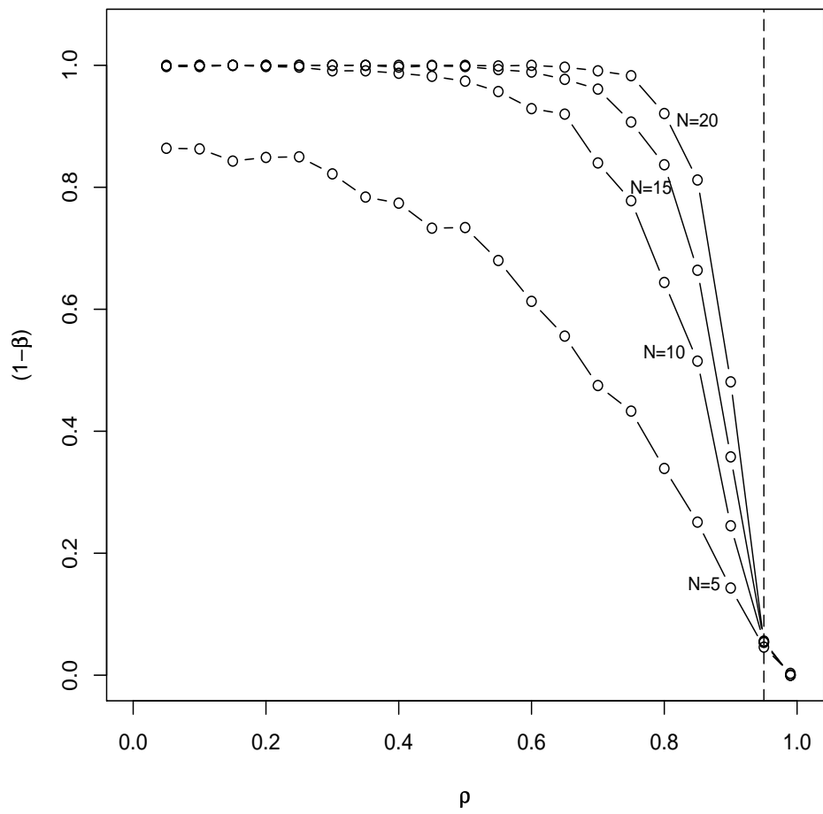
FIGURA 5: Poder do teste considerando número de provadores ( K=2 ) e número de produtos ( N=5, 10, 15, 20 )
