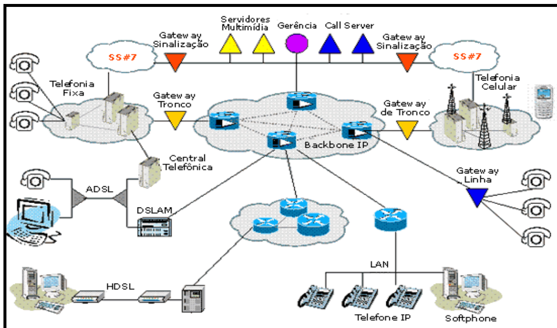
Figura 35 – Arquitetura NGN
