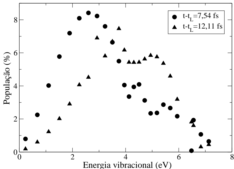
Figura 5.9: População ( \rho_\nu(t) = |\langle \nu | \phi(t) \rangle|^2 ) dos níveis vibracionais ( \nu = 0, 1, 2, \dots, 24 ) dos modos de estiramento O-H em diferentes tempos da propagação do pacote de onda do estado fundamental do dímero de água espacialmente orientado ( \varphi=0 e \theta = \pi/2 ). Os parâmetros do pulso de IV são: t_L=60 fs, \tau_L=7,9 fs, I_L=5,4 \times 10^{14} Wcm ^{-2} , \varphi_L=3,8 rad e \omega_L=0,45 eV.
