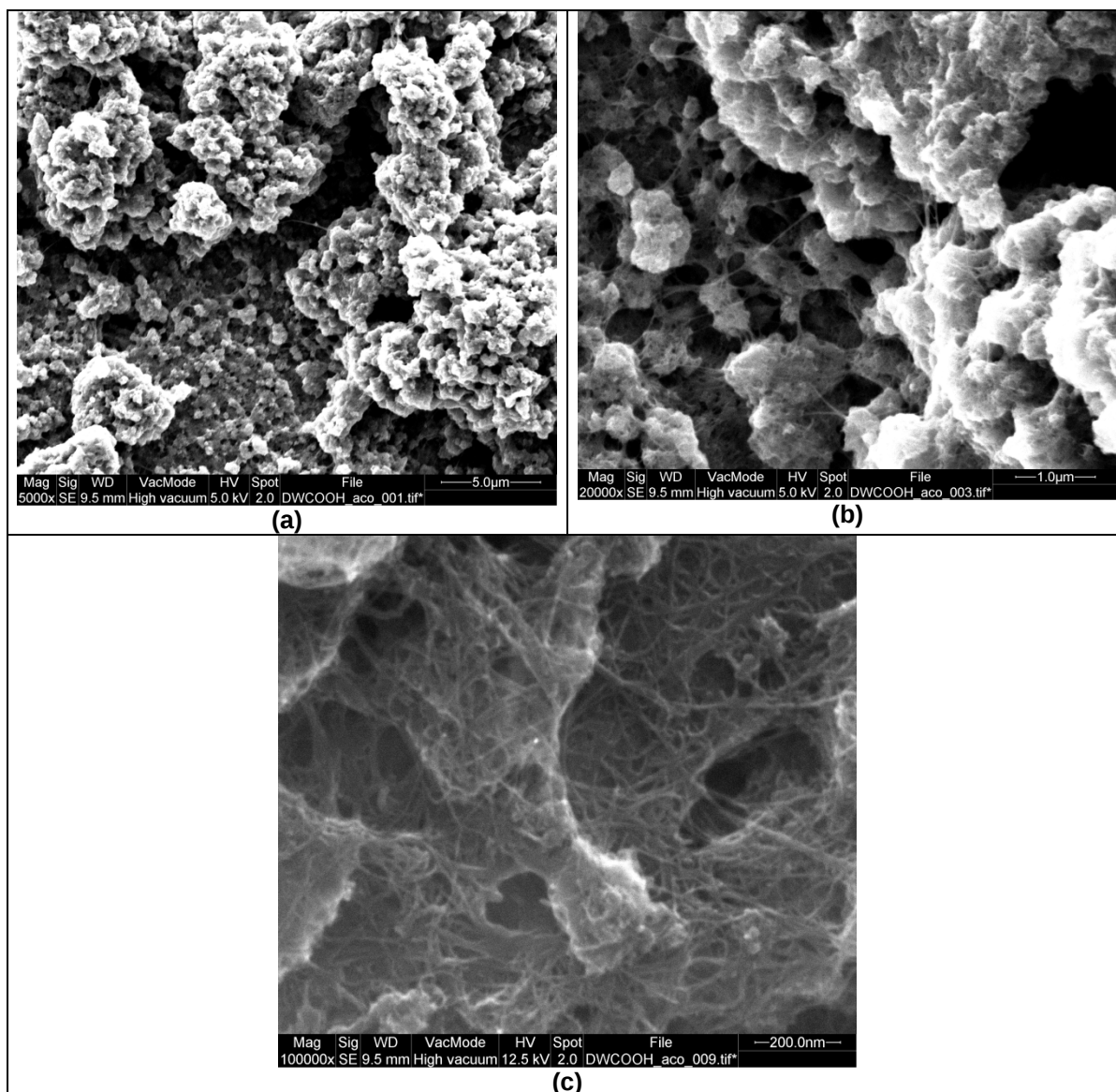
Figura 19: Microscopia Eletrônica de Varredura para o DWCNT-COOH, para diferentes magnitudes: (a) 5000, (b) 20000 e (c) 100000 vezes.
