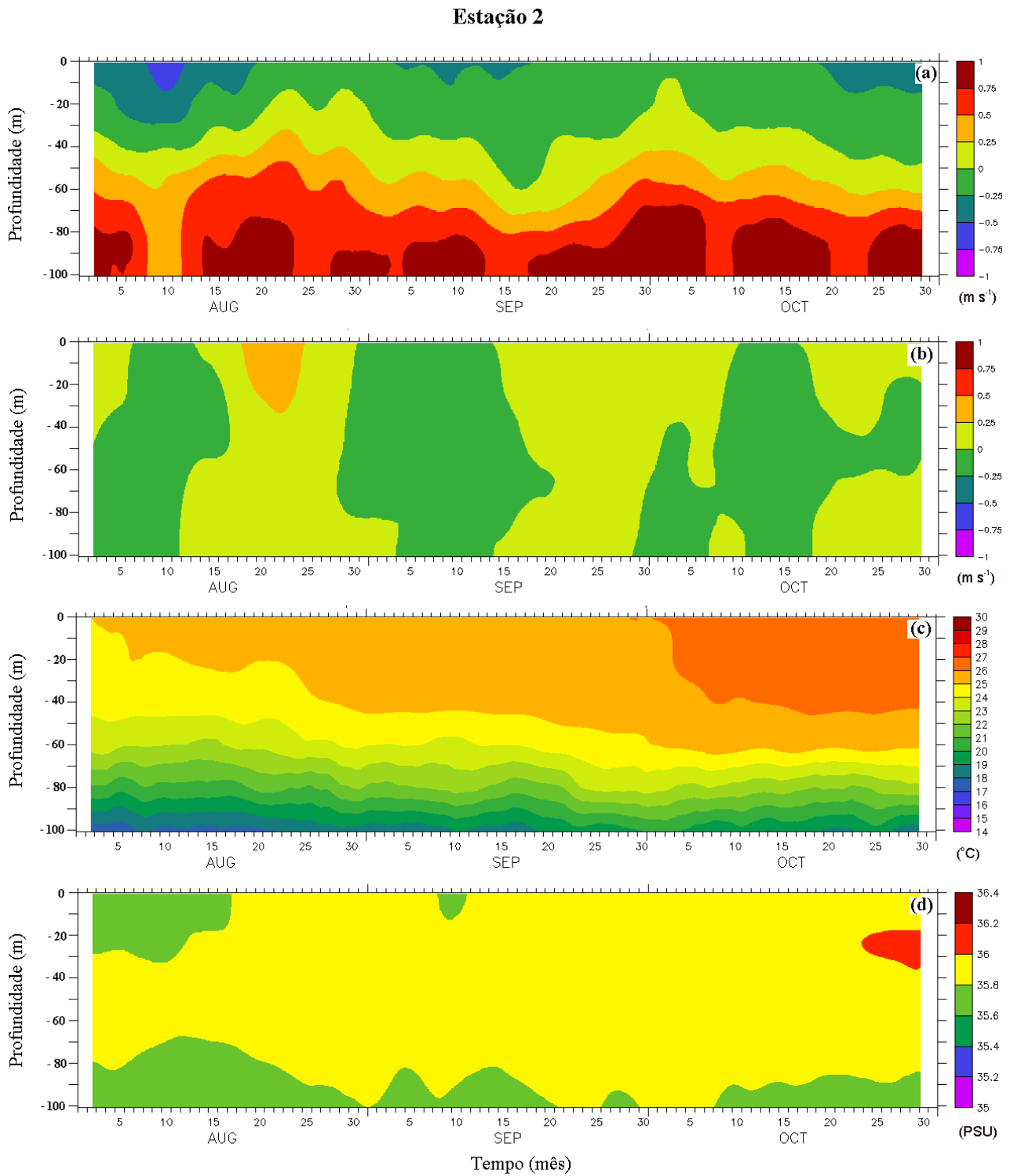
Figura 4.3: Reprodução das variáveis médias com o GOTM para a Estação 2. (a) U ; (b) V ; (c) \Theta e (d) S .
