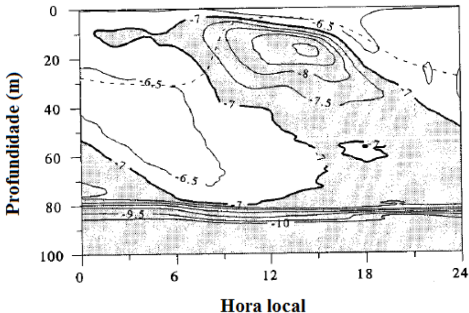
Figura 4.16: Ciclo diurno de \epsilon simulado com LES na camada superior oceânica considerando situações típicas do Oceano Pacífico equatorial. Linha tracejada indica h_{cmo}^{0,01} . Área hachurada indica região de \epsilon < 1 \times 10^{-7} \text{ m}^2 \text{ s}^{-3} , onde os autores consideram turbulência pouco desenvolvida. Adaptado de Wang et al. (1998).
