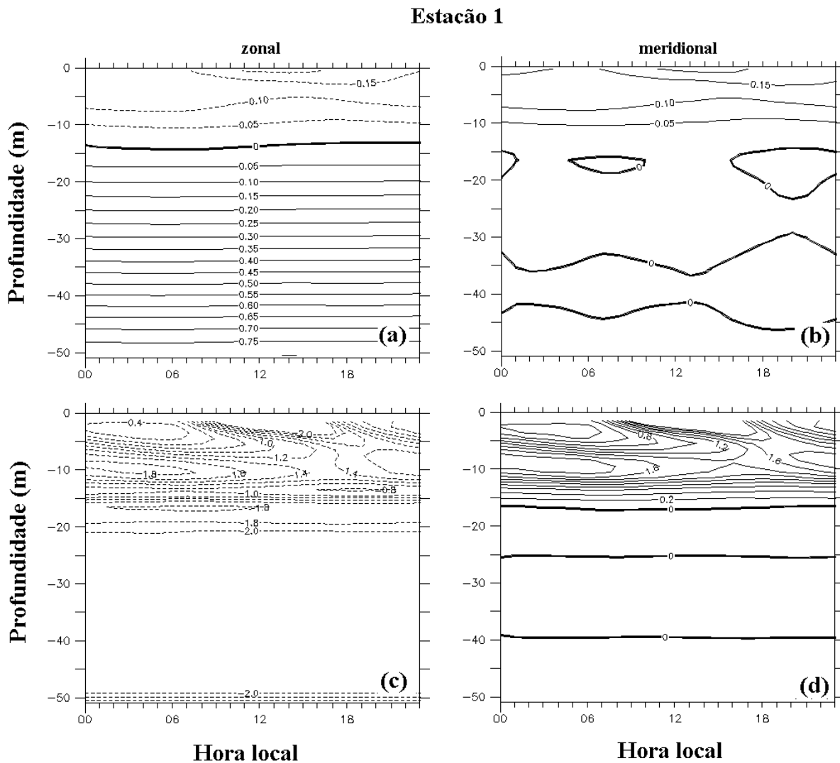
Figura 4.7: Perfis médios diurnos para a Estação 1 de (a) velocidade zonal ( U(z) ); (b) velocidade meridional ( V(z) ); (c) cisalhamento zonal ( \frac{\partial U}{\partial z} ) e (d) cisalhamento meridional ( \frac{\partial V}{\partial z} ). Velocidades em \text{m s}^{-1} e cisalhamento da corrente em 10^{-2} \text{ s}^{-1} . Linhas contínuas indicam valores positivos e linhas tracejadas valores negativos.
