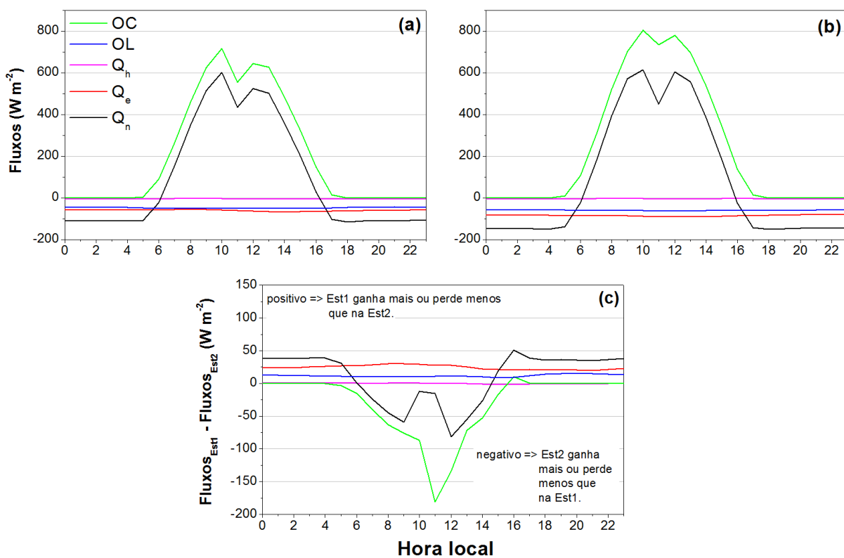
Figura 4.5: Balanço de calor médio diurno para (a) Estação 1 (fevereiro à abril), (b) Estação 2 (agosto a outubro) e (c) diferença dos ciclos diurnos entre as duas estações.
