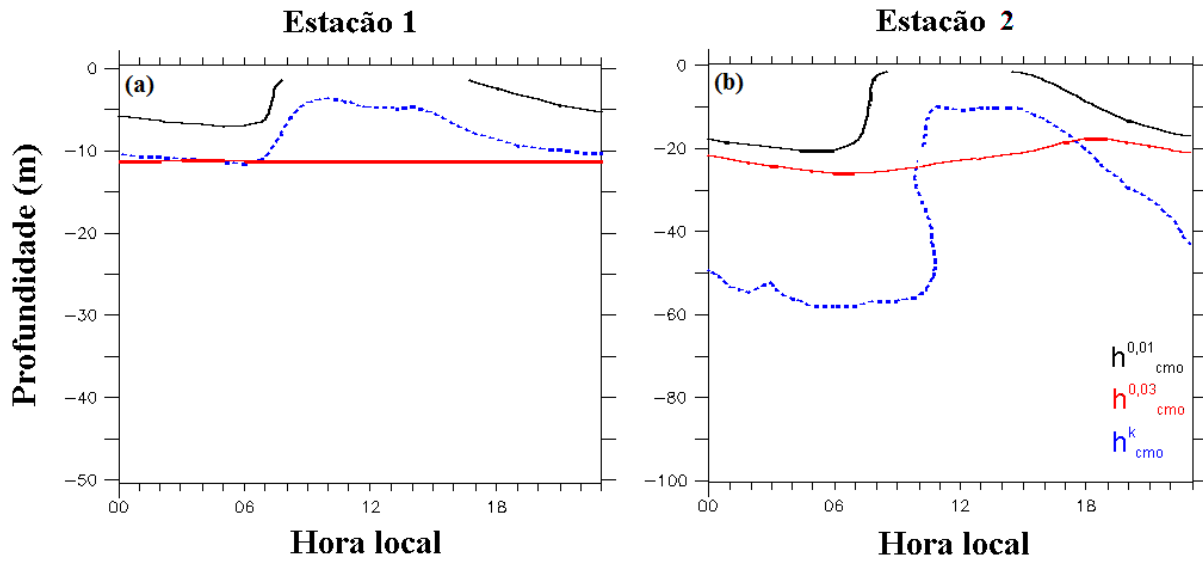
Figura 5.1: Comparação entre as profundidades das camadas de mistura oceânicas estimadas pelos diferentes critérios usados para (a) Estação 1 e (b) Estação 2. h_{cmo}^{0,01} estima a variação diurna da camada de mistura considerando a diferença de densidade de 0,01 \text{ kg m}^{-3} de seu valor na superfície; h_{cmo}^{0,03} é o critério sugerido por de Boyer Montégut et al. (2004) para estimar uma camada de mistura com rápida resposta às forçantes atmosféricas, mas negligenciando as variações diurnas, considerando a diferença de 0,03 \text{ kg m}^{-3} da de seu valor em z = -10 \text{ m} ; h_{cmo}^k é o critério de Burchard and Bolding (2001) para o GOTM usando a energia cinética turbulenta.
