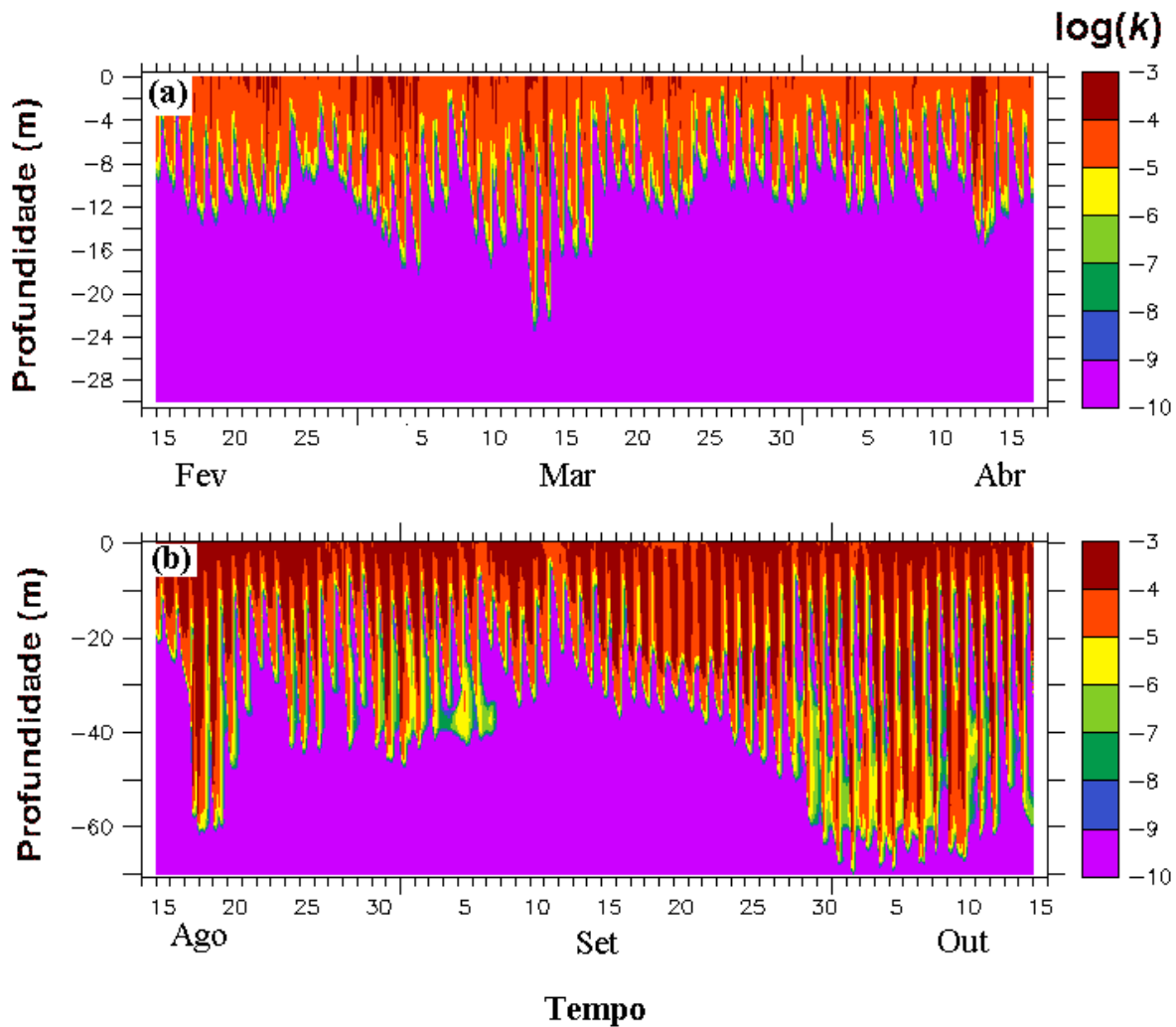
Figura 4.11: Simulação da evolução temporal de \log(k) para (a) Estação 1 e (b) Estação 2.
