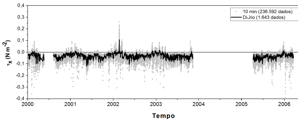
Figura 3.3: Série temporal de \tau_0^x , exemplificando as séries temporais resultantes da metodologia usada para o cálculo dos fluxos turbulentos de superfície e que foram utilizadas para calcular as climatologias horárias.
