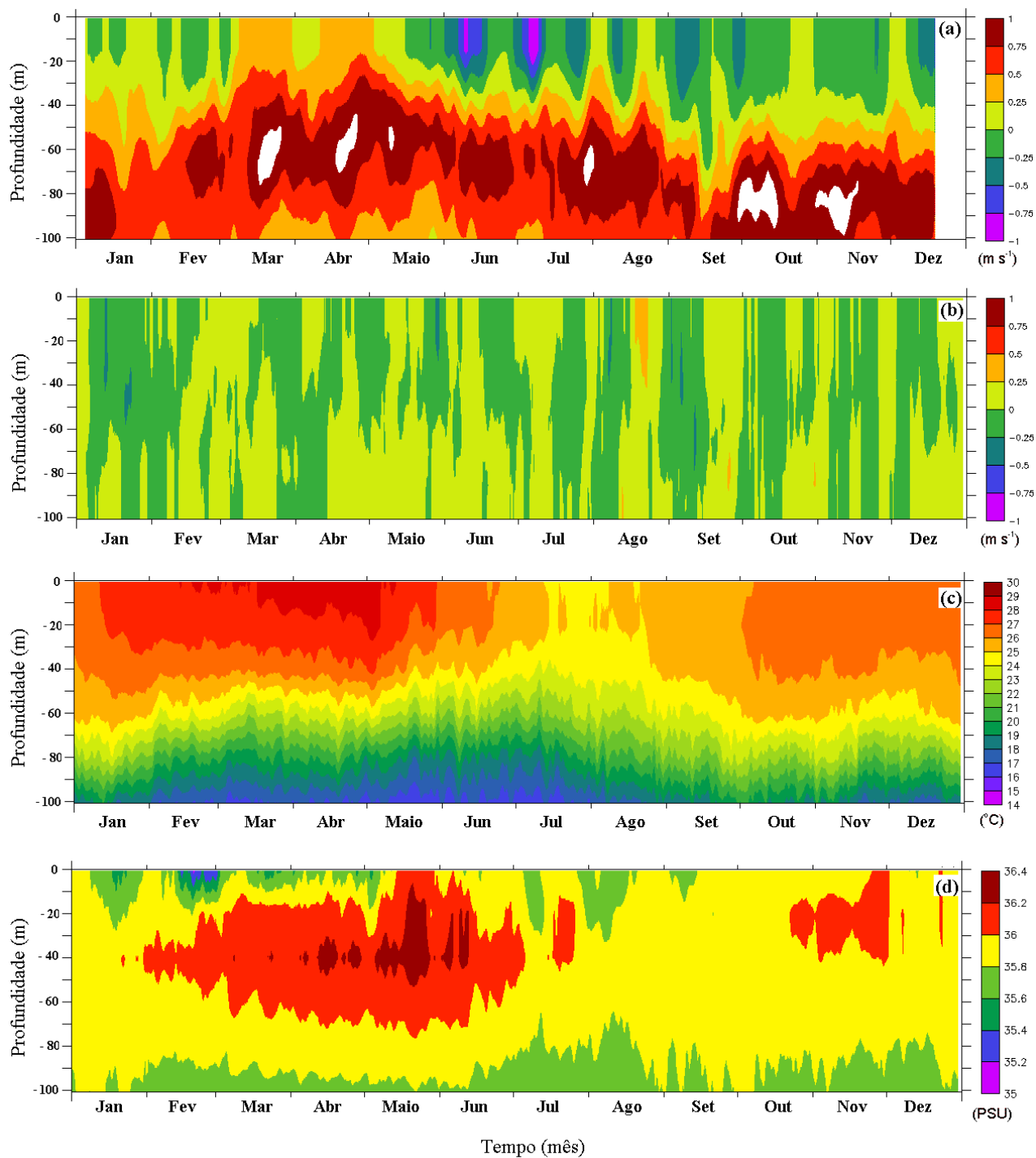
Figura 3.6: Médias horárias climatológicas dos perfis verticais de (a) velocidade zonal e (b) meridional, (c) temperatura e (d) salinidade. Séries temporais usadas nos termos de assimilação de dados na Eq. 2.7. A Tabela 3.2 mostra os períodos das séries temporais usadas para cada variável.
