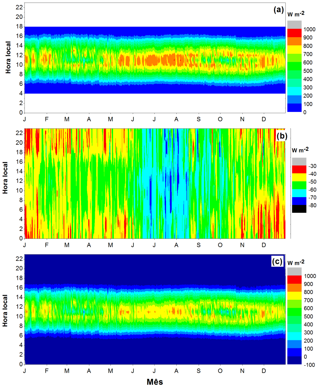
Figura 3.7: Médias horárias climatológicas de (a) balanço de onda curta (incidente do PIRATA e refletida do SRB); (b) balanço de onda longa (SRB) e (c) radiação líquida (OC+OL), usadas como CCS nas simulações com o GOTM. Médias horárias para o período de 1999 a 2005.
