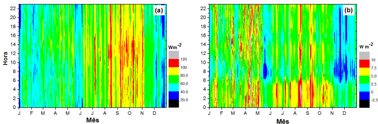
Figura 3.5: Médias horárias climatológicas de (a) fluxo de calor latente e (b) fluxo de calor sensível na superfície. Médias horárias para o período de 2000 a 2006 (Figura 3.3).
