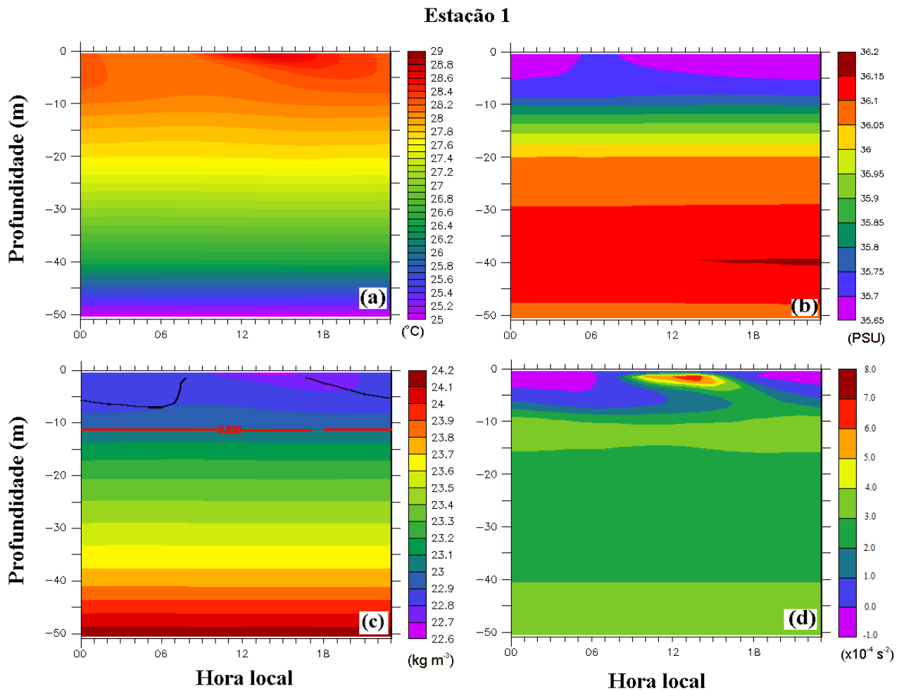
Figura 4.9: Perfis médios diurnos para a Estação 1 de (a) \theta(z) ; (b) S(z) ; (c) \rho(z) - 1000 e (d) N^2(z) . Em (c), a linha preta mostra a profundidade em que \rho(z) difere 0,01 \text{ kg m}^{-3} de seu valor na superfície e a linha vermelha mostra a profundidade em que \rho difere 0,03 \text{ kg m}^{-3} de seu valor em z = -10 \text{ m} .
