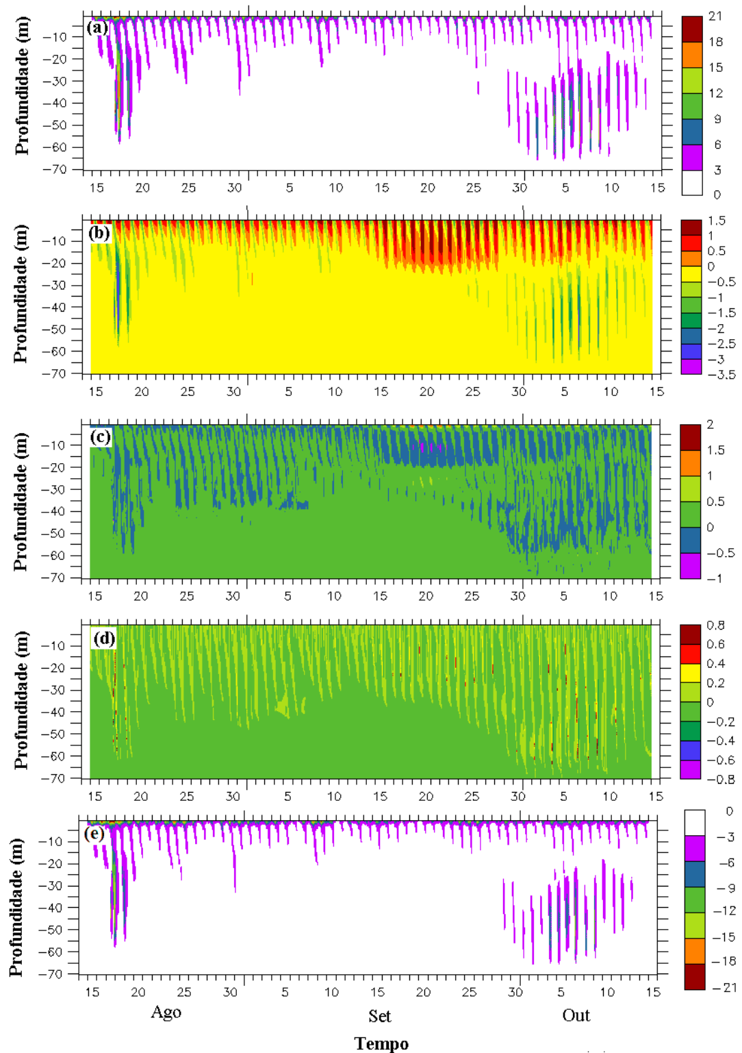
Figura 4.13: Simulação da evolução temporal dos termos da equação de k (Eq. 2.18) para a Estação 1. (a) Produção mecânica; (b) produção/dissipação térmica; (c) difusão vertical; (d) variação local e (d) taxa de dissipação viscosa. Unidade em 10^{-7} \text{ m}^2 \text{ s}^{-3} .
