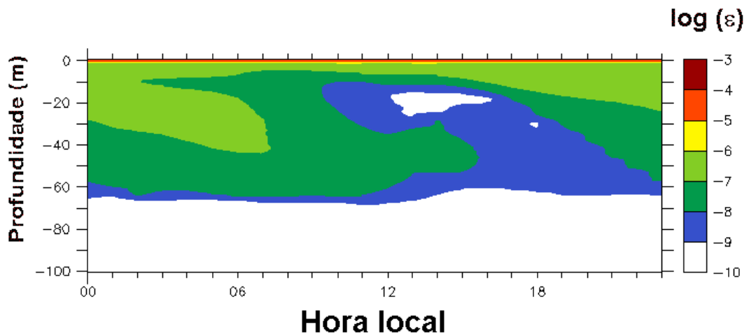
Figura 4.15: Perfil médio diurno de \log(\epsilon) para a Estação 2 (15 de agosto à 30 de outubro).
