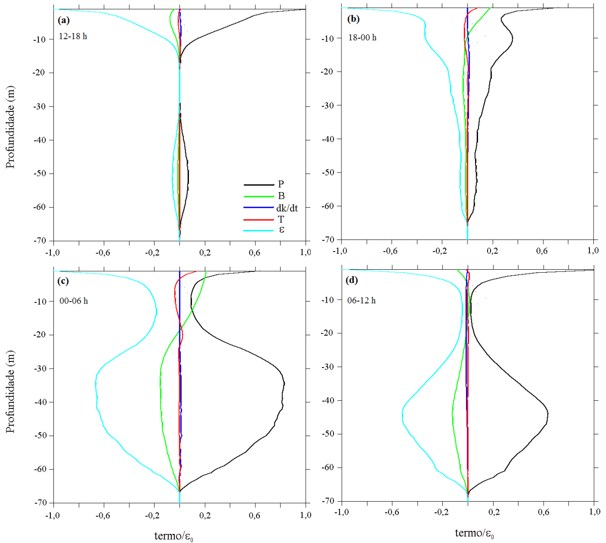
Figura 4.21: Perfis verticais médios dos termos da equação de k (Eq. 2.18) para o período de 01 a 11 de outubro. (a) Média entre 12-18 h; (b) média entre 18-00 h; (c) média entre 00-06 h e (d) média entre 06-12 h. Os termos foram normalizados pela média de \epsilon na superfície em cada intervalo do dia.
