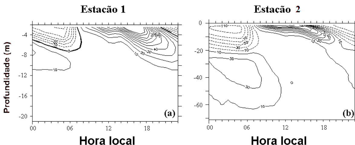
Figura 4.18: Perfil médio diurno do fluxo líquido de calor no oceano ( \text{W m}^{-2} ), para (a) Estação 1 e (b) Estação 2. Linhas tracejadas indicam valores negativos e significam perda de calor.
