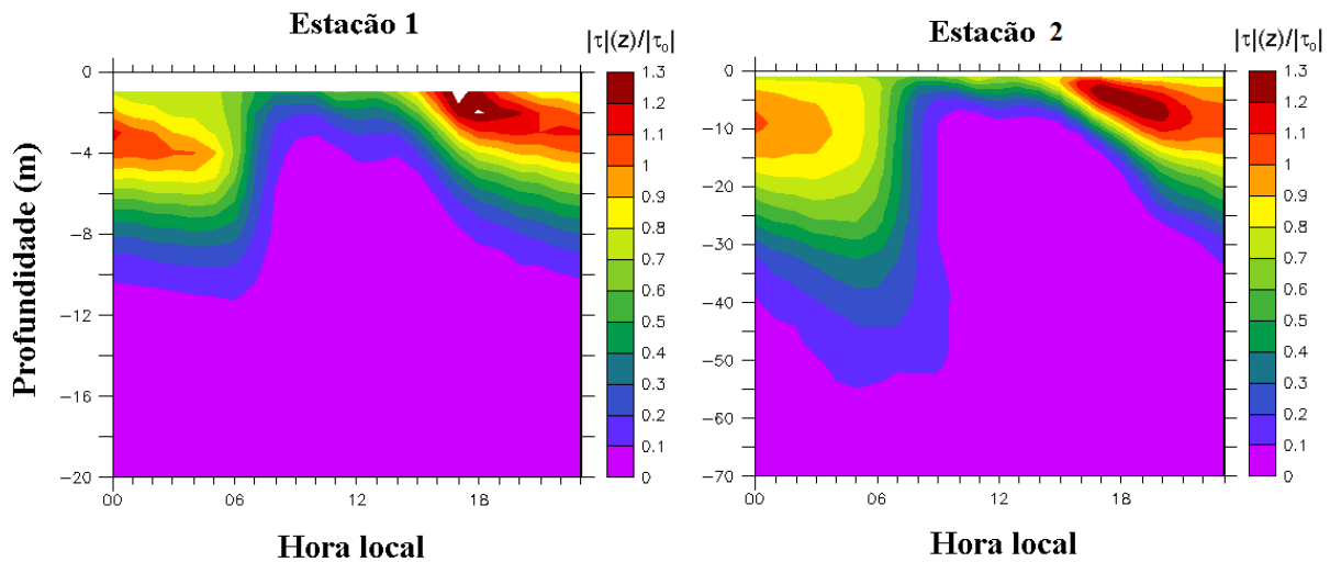
Figura 4.17: Perfil médio diurno do fluxo de momento |\vec{\tau}(z)| normalizado pela tensão de cisalhamento na superfície para (a) Estação 1 e (b) Estação 2.
