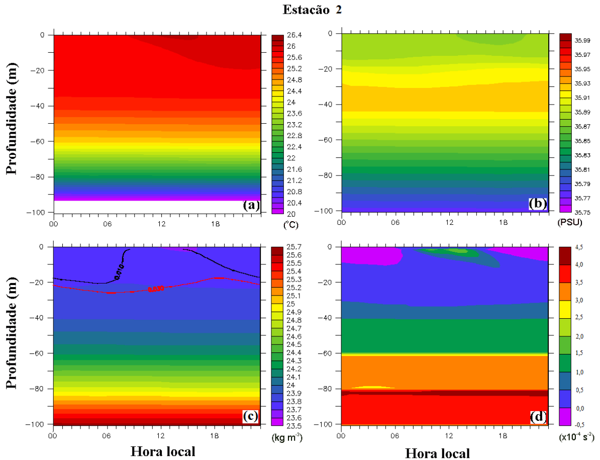
Figura 4.10: Perfis médios diurnos para a Estação 2 de (a) \theta(z) ; (b) S(z) ; (c) \rho(z) - 1000 e (d) N^2(z) . Em (c), a linha preta mostra a profundidade em que \rho(z) difere 0,01 \text{ kg m}^{-3} de seu valor na superfície e a linha vermelha mostra a profundidade em que \rho difere 0,03 \text{ kg m}^{-3} de seu valor em z = -10 \text{ m} .
