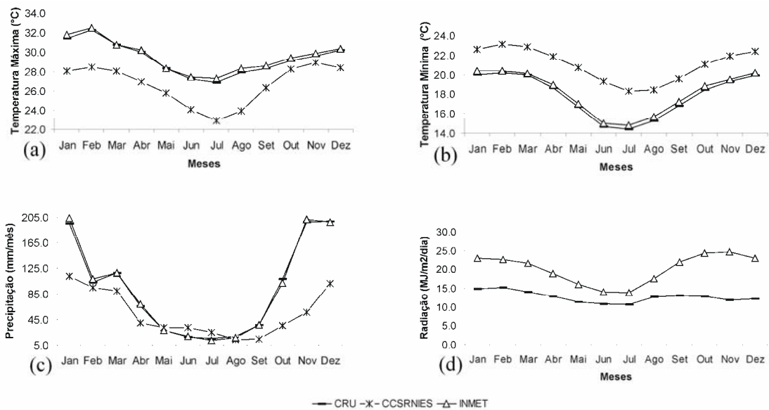
Figura 6 – Comportamento sazonal dos dados do CRU, CCSR/NIES e INMET no período de 1961-1990 na localidade de Governador Valadares, (a) temperatura máxima (°C), (b) temperatura mínima (°C), (c) precipitação (mm) e (d) radiação (MJ m -2 por dia).
