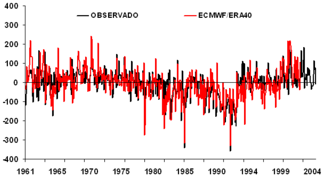
Figura 18F – Anomalias mensais de radiação global incidente dos registros observados e de reanálise do ECMWF/ERA40 para a Mesorregião de Belo Horizonte (MR10), em \text{MJ}/\text{m}^2\text{mês} , no período de 1961 a 2002 para ECMWF/ERA40 e 1961 a 2004 para o observado – PRESENTE.
