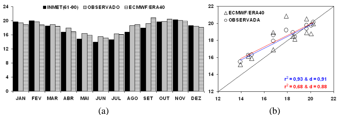
Figura 7G – Climatologia da radiação global incidente, em MJ/m 2 d, da Mesorregião Triângulo Mineiro/Alto Paranaíba (MR11), no período de 1961 a 1990 – PRESENTE (a); validações das séries de dados observados e do ECMWF/ERA40 (na abscissa climatologia oficial do INMET) (b).
