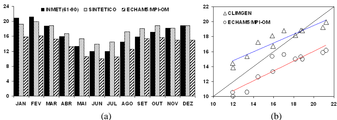
Figura 9D – Climatologia da radiação global incidente, em MJ/m 2 d, da mesorregião Vale do Rio Doce (MR06), no período de 1991 a 2020 – FUTURO (a); validações entre as climatologias das séries simuladas pelo CLIMGEN e o ECHAM5/MPI-OM (na abscissa climatologia oficial do INMET) (b).
