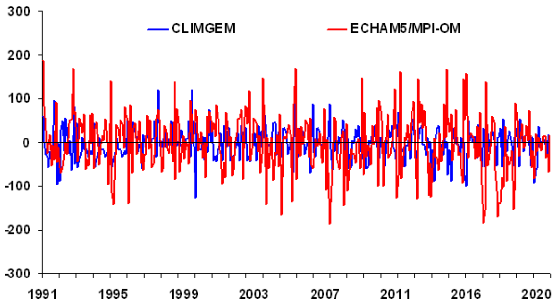
Figura 19F – Anomalias mensais de radiação global total dos registros simulados pelo CLINGEM (séries sintéticas) e ECHAM5/MPI-OM (série dinâmica) para Mesorregião de Belo Horizonte (MR10), em \text{MJ}/\text{m}^2\text{mês} , no período de 1991 a 2020 – FUTURO.
