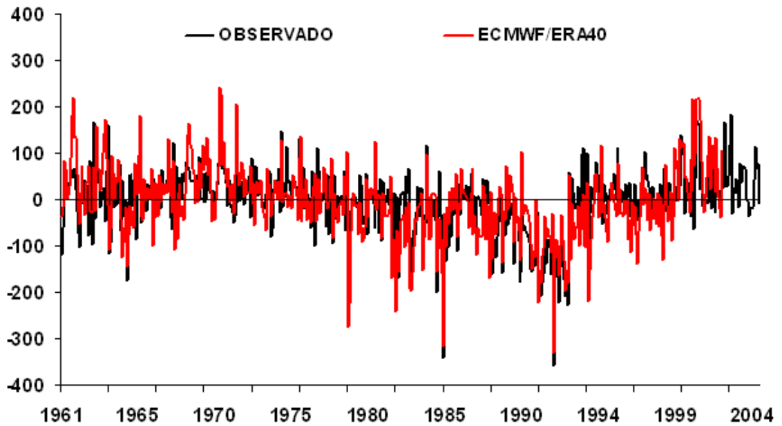
Figura 18H – Anomalias mensais de radiação global incidente dos registros observados e de reanálise do ECMWF/ERA40 para a Mesorregião Zona da Mata Mineira (MR12), em \text{MJ}/\text{m}^2\text{mês} , no período de 1961 a 2002 para ECMWF/ERA40 e 1961 a 2004 para o observado – PRESENTE.
