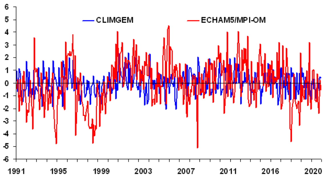
Figura 15B – Anomalias mensais de temperatura máxima a partir de “registros simulados pelo CLINGEM (séries sintéticas) e ECHAM5/MPI-OM (série dinâmica)” para mesorregião Sul e Sudoeste de Minas (MR01), em °C, no período de 1991 a 2020 – FUTURO.
