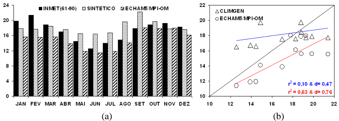
Figura 9E – Climatologia da radiação global incidente, em MJ/m 2 d, da mesorregião Central Mineira (MR09), no período de 1991 a 2020 – FUTURO (a); validações entre as climatologias das séries simuladas pelo CLIMGEN e o ECHAM5/MPI-OM (na abscissa climatologia oficial do INMET).
