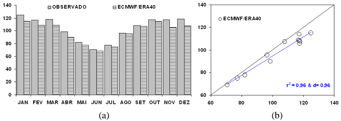
Figura 10F – Climatologia da evapotranspiração de referência mensal, em mm, da Mesorregião de Belo Horizonte (MR10), no período de 1961 a 1990 – PRESENTE (a); validações das séries de dados em reanálise do ECMWF/ERA40 (na abscissa climatologia oficial do INMET) (b).
