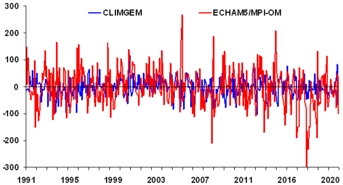
Figura 18G – Anomalias mensais de radiação global total dos registros simulados pelo CLIMGEM (séries sintéticas) e ECHAM5/MPI-OM (série dinâmica) para Triângulo Mineiro/Alto Paranaíba (MR11), em MJ/m 2 mês, no período de 1991 a 2020 – FUTURO.
