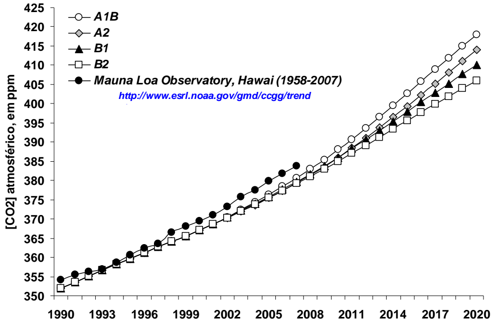
Figura 2A – Concentrações de CO 2 na atmosfera medida (NOAA) e simulada (IPCC, 2001 e 2007), em ppmv.
