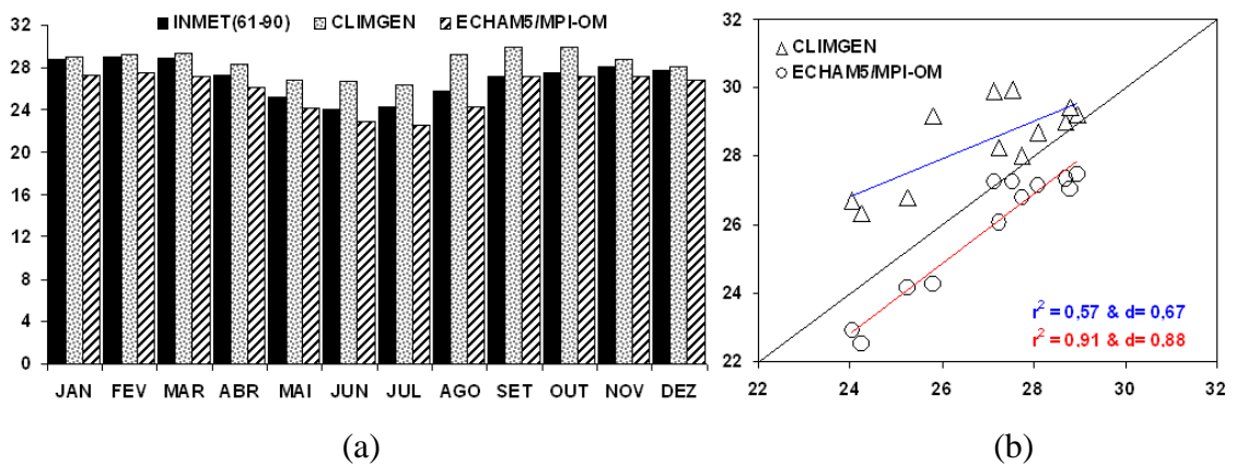
Figura 5B – Climatologia da temperatura máxima, em °C, da mesorregião Sul e Sudoeste de Minas Gerais (MR01), no período de 1991 a 2020 – FUTURO (a); validações entre as climatologias das séries simuladas pelo CLIMGEN e o ECHAM5/MPI-OM (na abscissa climatologia oficial do INMET) (b).
