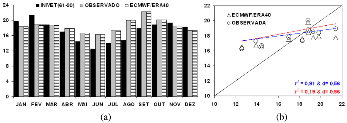
Figura 8E – Climatologia da radiação global incidente, em MJ/m 2 d, da mesorregião Central Mineira (MR09), no período de 1961 a 1990 – PRESENTE (a); validações das séries de dados observados e do ECMWF/ERA40 (na abscissa climatologia oficial do INMET) (b).
