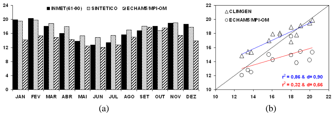
Figura 9F – Climatologia da radiação global incidente, em MJ/m 2 d, da Mesorregião de Belo Horizonte (MR10), no período de 1991 a 2020 – FUTURO (a); validações entre as climatologias das séries simuladas pelo CLIMGEN e o ECHAM5/MPI-OM (na abscissa climatologia oficial do INMET) (b).
