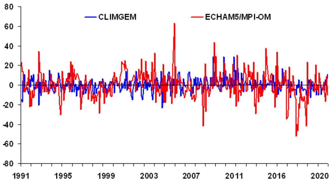
Figura 23 – Anomalias mensais de evapotranspiração de referência estimada com registros meteorológicos simulados pelo CLIMGEM (séries sintéticas) e ECHAM5/MPI-OM (série dinâmica) para a mesorregião Jequitinhonha (MR04), em mm/mês, no período de 1991 a 2020 – FUTURO.
