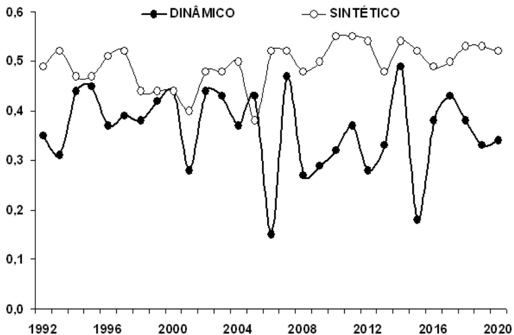
Figura 52 – Índice de colheita do cultivar BR201. Impactos e projeções do clima por meio de séries meteorológicas dinâmicas (ECHAM5/MPI-OM) e sintéticas (CLIMGEN) para mesorregião do Triângulo Mineiro e Alto Paranaíba (MR11).
