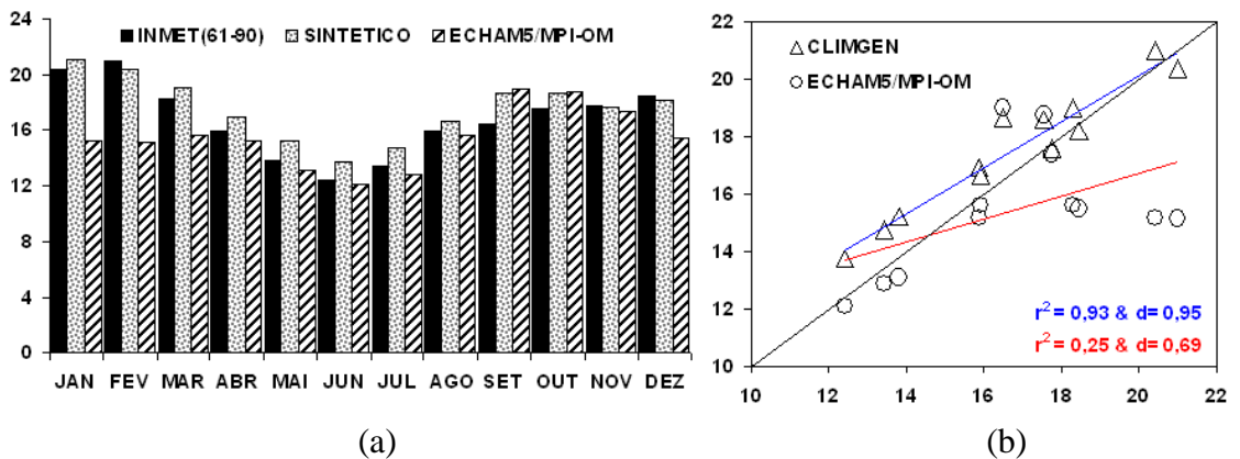
Figura 11 – Climatologia da radiação global incidente, em MJ/m 2 d, da mesorregião Jequitinhonha (MR04), no período de 1991 a 2020 – FUTURO (a); validações entre as climatologias das séries simuladas pelo CLIMGEN e o ECHAM5/MPI-OM (na abscissa climatologia oficial do INMET) (b).
