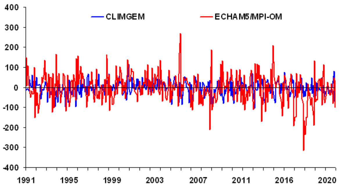
Figura 19H – Anomalias mensais de radiação global total dos registros simulados pelo CLINGEM (séries sintéticas) e ECHAM5/MPI-OM (série dinâmica) para Mesorregião Zona da Mata Mineira (MR12), em \text{MJ}/\text{m}^2\text{mês} , no período de 1991 a 2020 – FUTURO.
