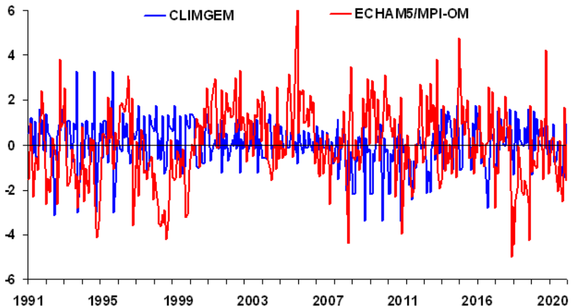
Figura 14G – Anomalias mensais de temperatura máxima a partir de “registros simulados pelo CLIMGEM (séries sintéticas) e ECHAM5/MPI-OM (série dinâmica)” para Mesorregião Triângulo Mineiro/Alto Paranaíba (MR11), em °C, no período de 1991 a 2020 – FUTURO.
