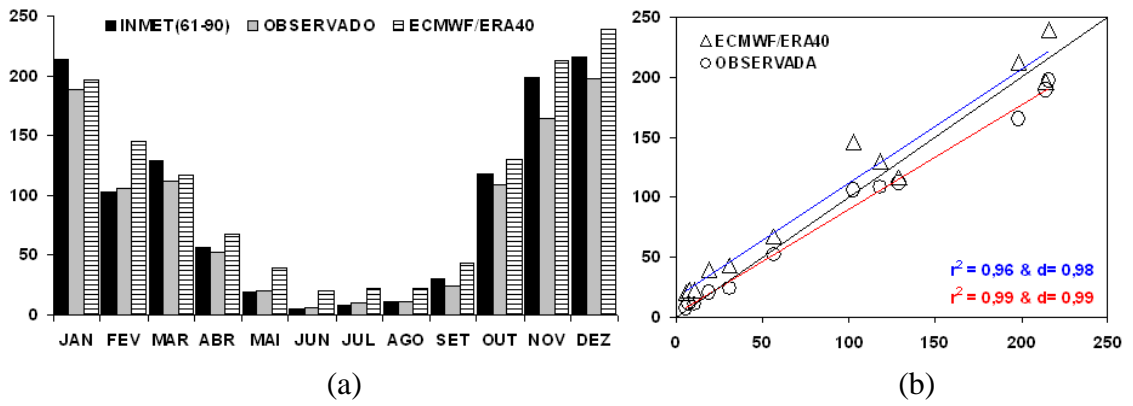
Figura 4 – Climatologia da precipitação acumulada mensal da mesorregião Jequitinhonha (MR04), em mm, no período de 1961 a 1990 – PRESENTE (a); validações das séries de dados observados e do ECMWF/ERA40 (na abscissa climatologia oficial do INMET) (b).
