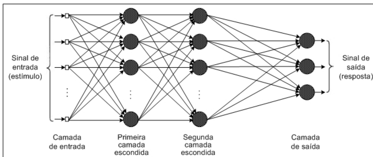
Figura 2 - Rede neural MLP com duas camadas escondidas e uma camada de saída
