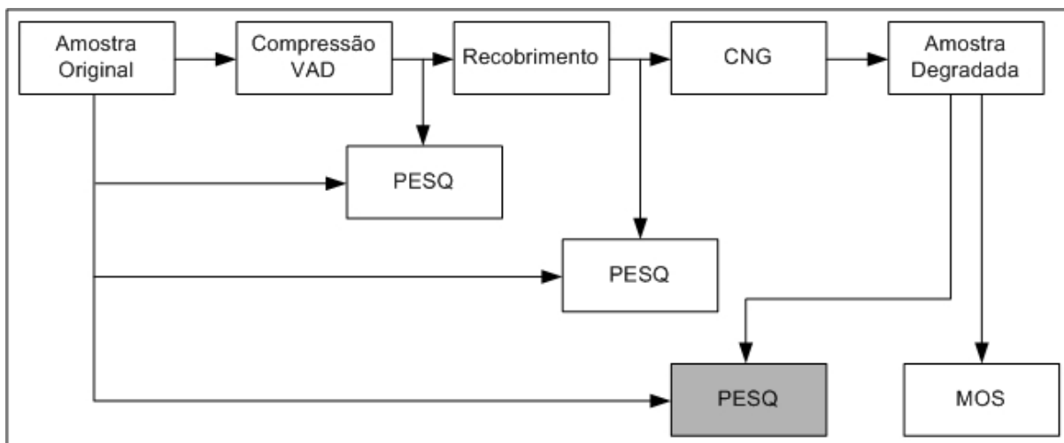
Figura 32 - Diagrama de blocos do cenário com destaque para o sinal avaliado pelo PESQ - com ruído de conforto
