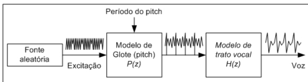
Figura 7 - Modelo de predição linear da voz Fonte: Vasegui (2000)
