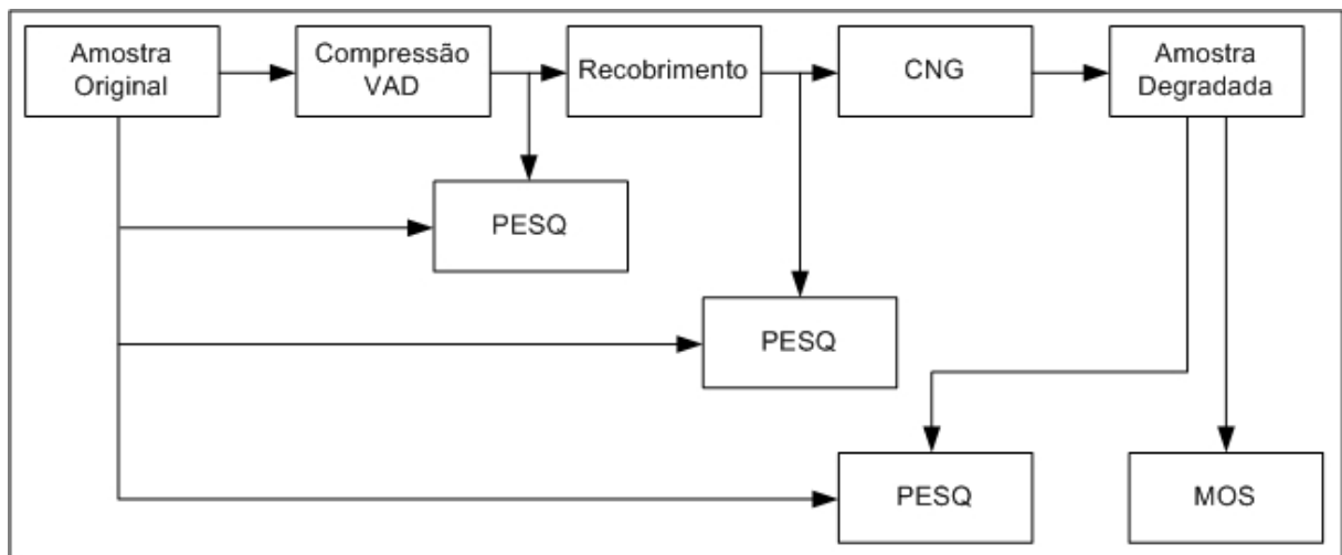
Figura 25 - Diagrama de blocos do sistema a ser implementado e sinais a serem avaliados pelo PESQ e pelo MOS
