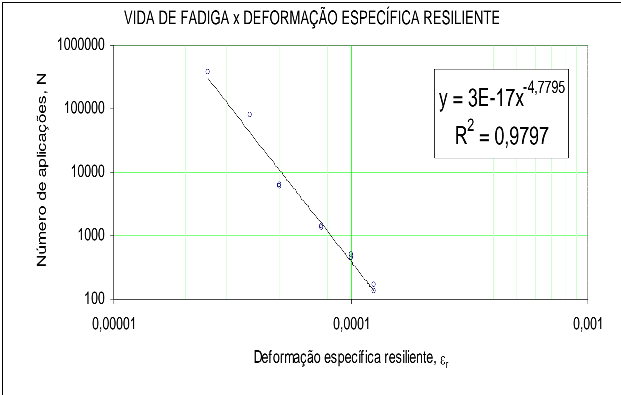
Gráfico A6 – Vida de fadiga x deformação específica resiliente ( 100 % de lodo como filler )
