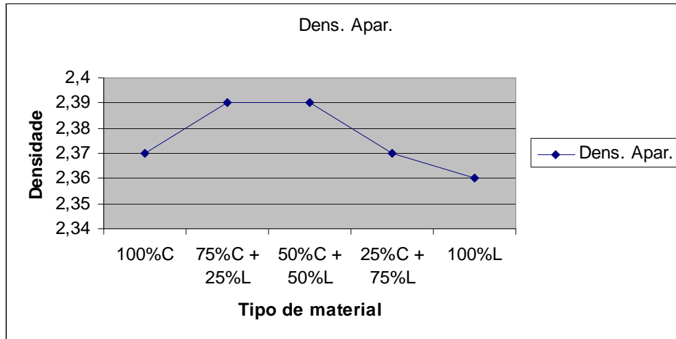
Figura 45 – Evolução da densidade aparente com a quantidade de lodo deste estudo
