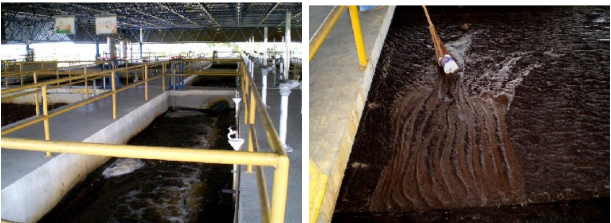
Figura 12 – Vista parcial da ETA 2; Figura 13 – Coleta do lodo na ETA 2 (Fotos do autor: ETA da Ponta do Ismael, 2007).
