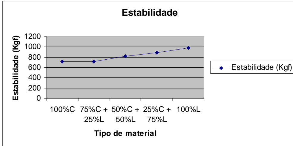
Figura 47 – Evolução da estabilidade com a quantidade de lodo deste estudo
