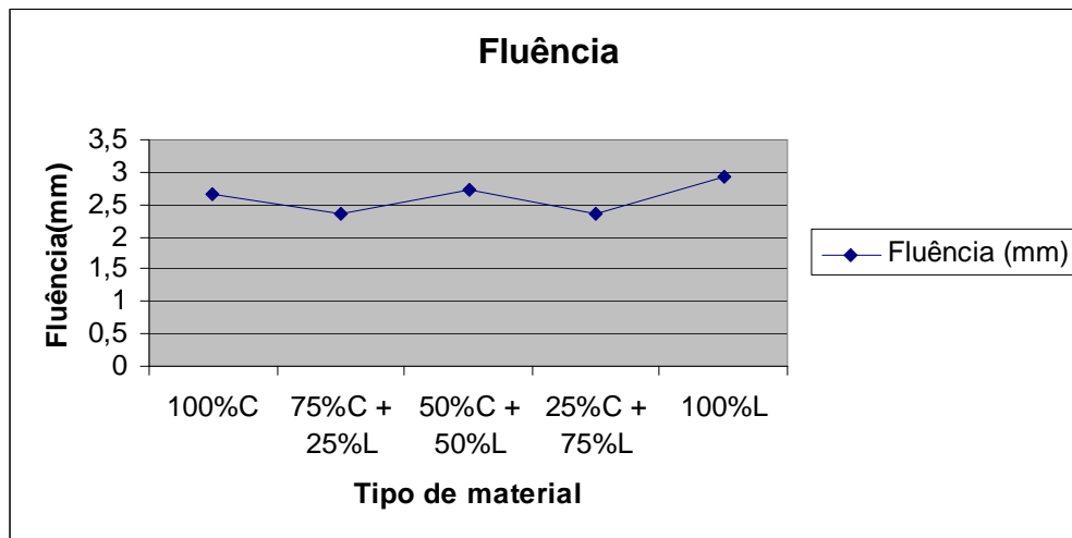
Figura 48 – Evolução da fluência com a quantidade de lodo deste estudo
