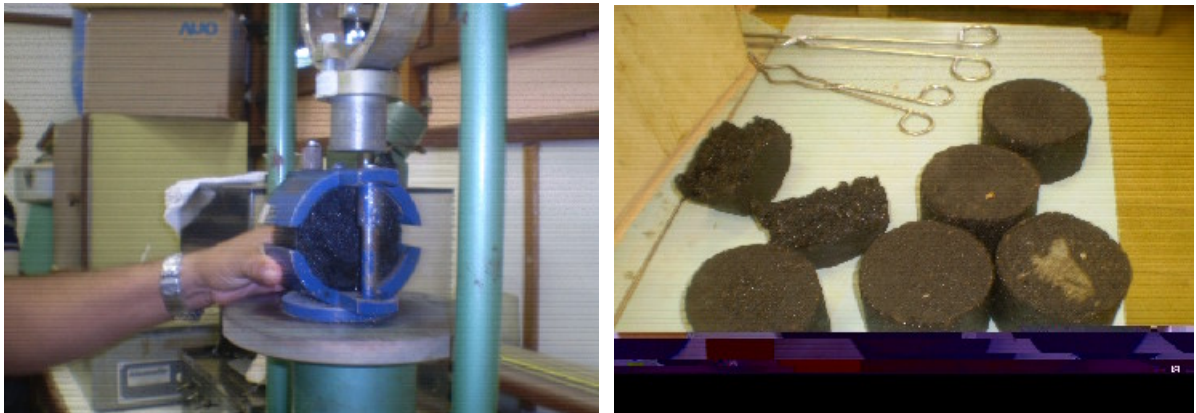
Figura 23 - Ensaio Marshall; Figura 24 - Corpo de prova rompido no ensaio Marshall (Fotos do autor: Laboratório de Pavimentação da UFAM, 2007).
