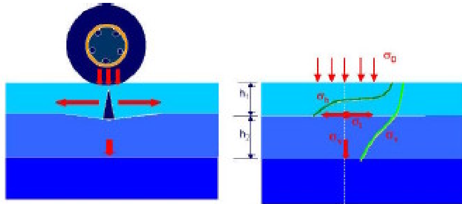
Figura 3 – Tensões em um pavimento (MEDINA, 1997)
