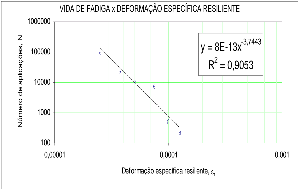
Gráfico A5 – Vida de fadiga x deformação específica resiliente ( 50 % de lodo como filler )
