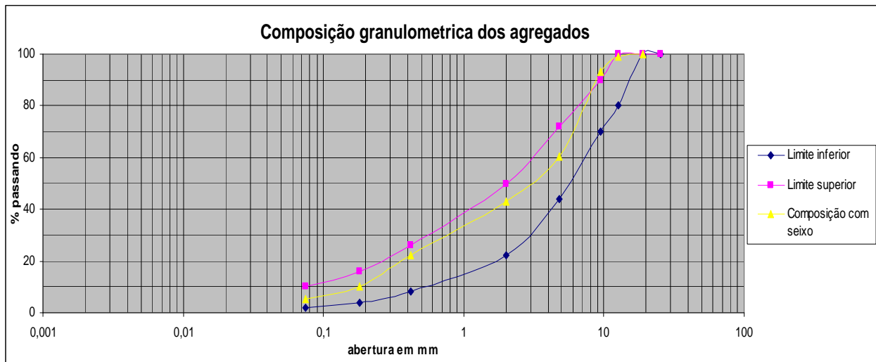
Figura 38 - Composição granulométrica dos agregados utilizado nesta pesquisa
