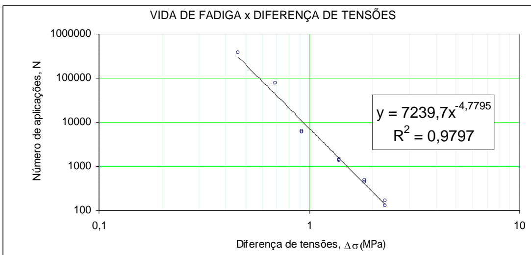
Figura 52 –Vida de fadiga x diferença de tensões de CBUQ com 100 % de lodo
