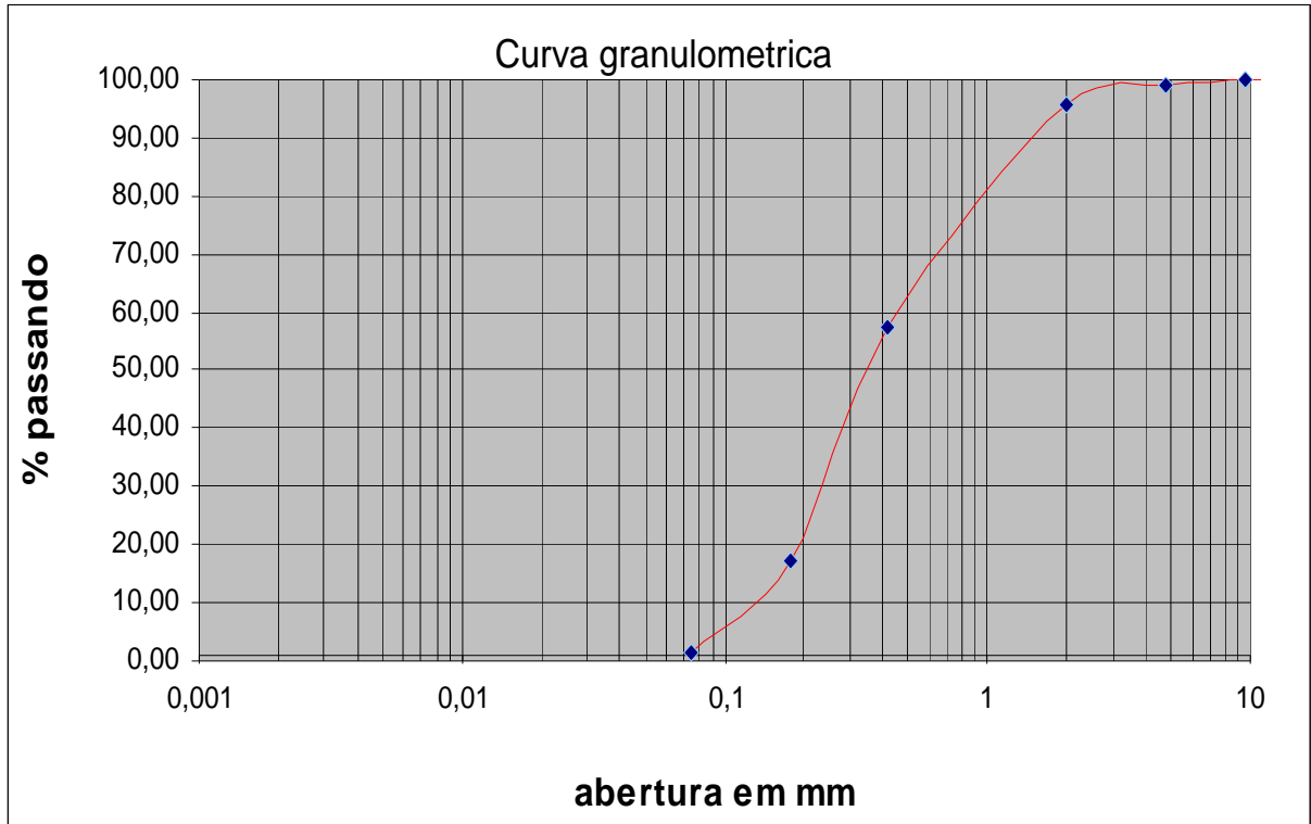
Figura 1 – Curva granulométrica do agregado miúdo (areia)
