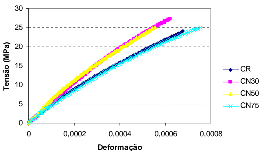
FIGURA 4.6 – Relação tensão versus deformação para as argamassas da primeira etapa – 28 dias
