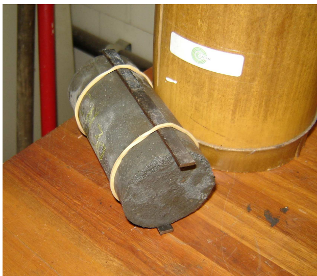
FIGURA 3.19 – Peças metálicas usadas no ensaio de tração por compressão diametral
