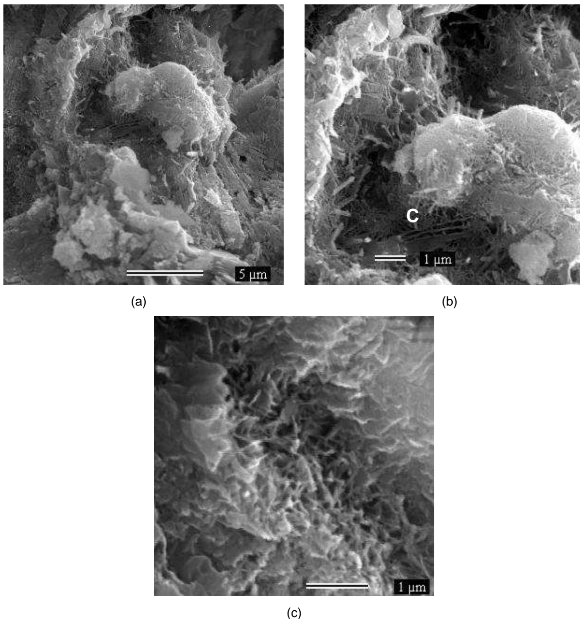
FIGURA 4.12 – Microscopia da amostra CN75 aos 28 dias. (a) Ampliação de 5.000x. (b) Ampliação de 10.000x. (c) Ampliação de 20.000x
