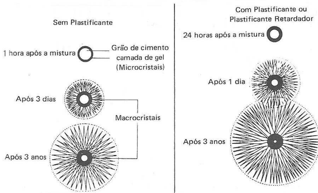
FIGURA 2.5 – Seqüência de hidratação e endurecimento na pasta de cimento Fonte: BAUER, 1994.
