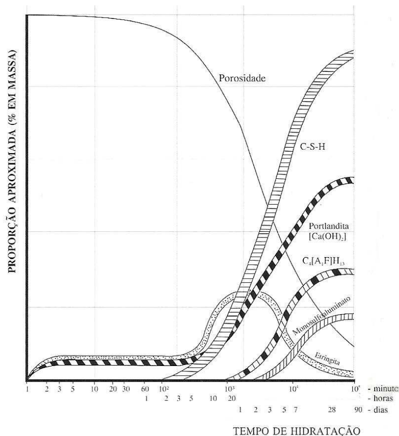
FIGURA 2.1 – Curvas aproximadas da evolução das fases hidratadas e da porosidade da pasta de cimento em função do tempo de hidratação
