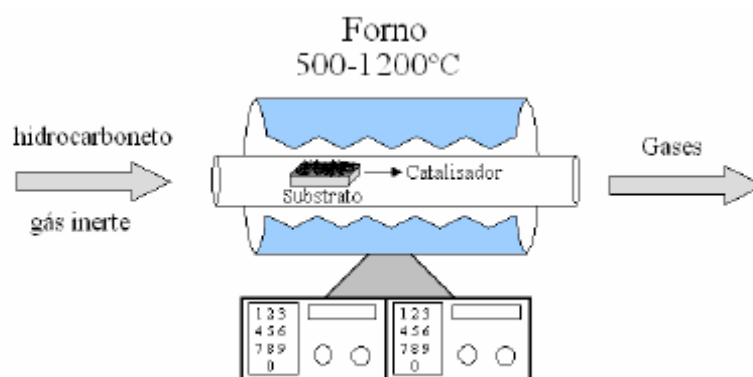
FIGURA 2.16 – Desenho esquemático do processo CVD Fonte: COUTO, 2006.
