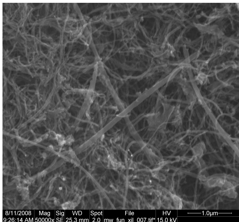
FIGURA 3.9 – Microscopia eletrônica de varredura dos nanotubos funcionalizados. (a) Ampliação de 8.000x. (b) Ampliação de 20.000x. (c) Ampliação de 50.000x
