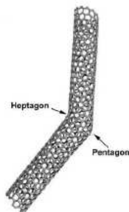
FIGURA 2.14 – Curvatura de nanotubo devido à presença de um pentágono na rede hexagonal Fonte: HINOJOSA, 2007.
