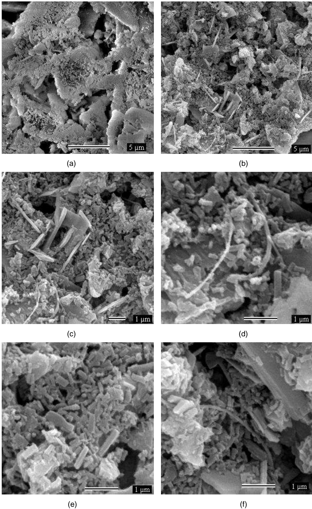
FIGURA 3.14 – Microscopia do traço 6. (a) e (b) Ampliação de 5.000x. (c) Ampliação de 10.000x. (d), (e) e (f) Ampliação de 20.000x
