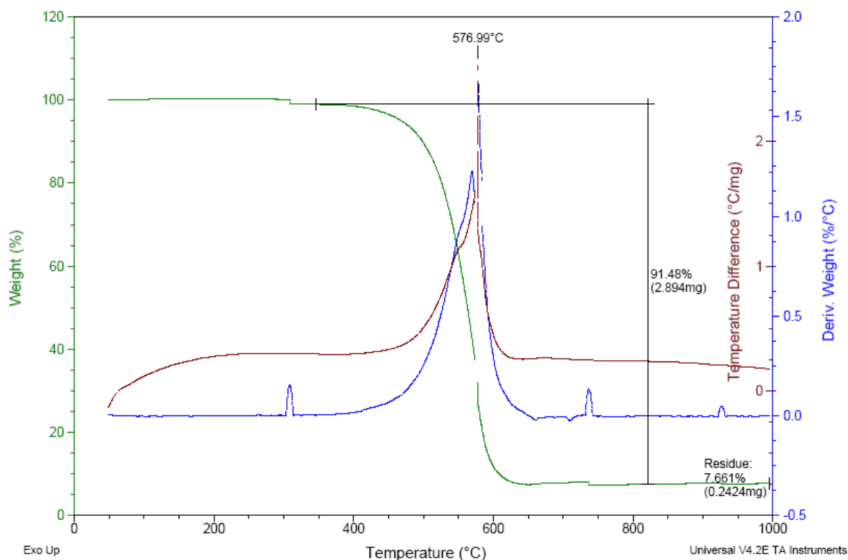
FIGURA 3.10 – Curva de termogravimetria (TG) e análise térmica diferencial (ATD) dos nanotubos funcionalizados
