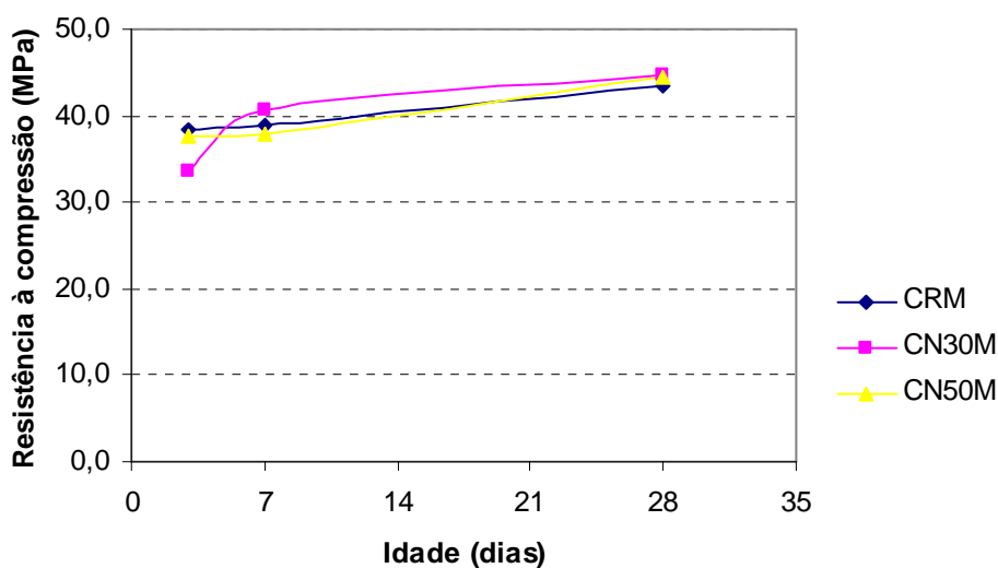
FIGURA 4.2 – Evolução da resistência à compressão – Segunda etapa
