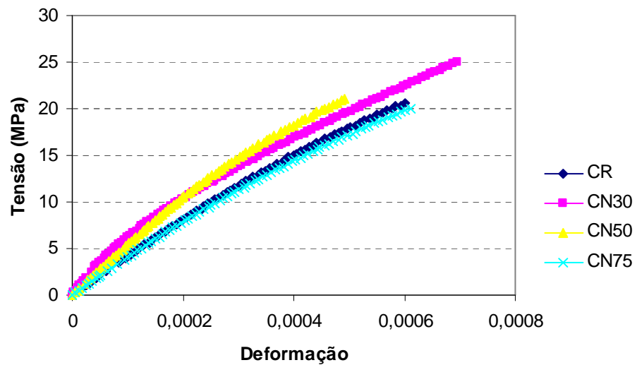
FIGURA A.2 – Relação tensão versus deformação para as argamassas da primeira etapa – 7 dias
