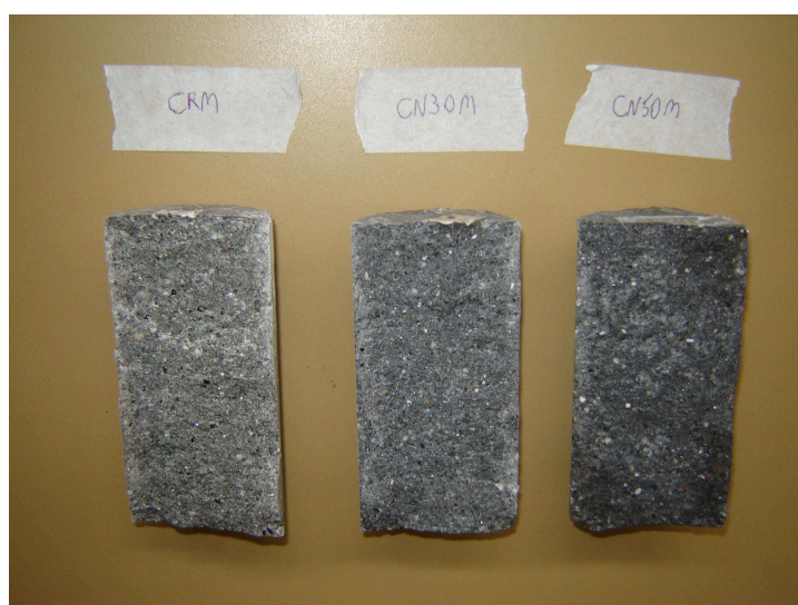
FIGURA 4.5 – Coloração dos três traços realizados na segunda etapa: CRM, CN30M e CN50M (da esquerda para direita)
