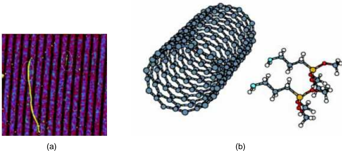
FIGURA 1.1 – (a) Nanotubos depositados em superfície funcionalizada por moléculas orgânicas. (b) Simulação de um nanotubo (em cinza) aderido a moléculas orgânicas
