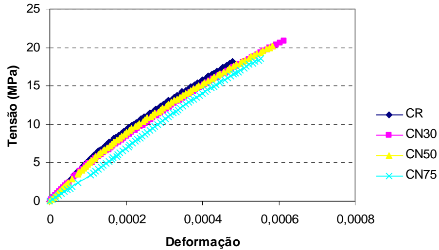
FIGURA A.1 – Relação tensão versus deformação para as argamassas da primeira etapa – 3 dias
