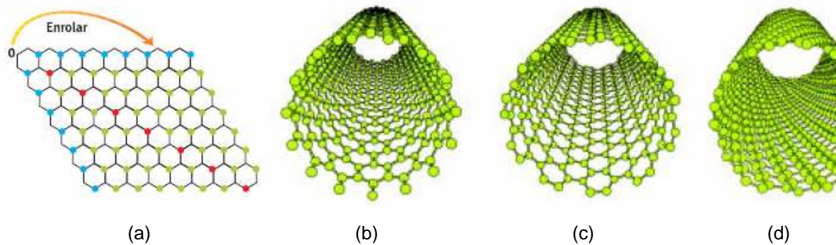
FIGURA 2.12 – Enrolamento de uma folha de grafeno. (a) Folha de grafeno aberta. (b) Nanotubo tipo ziguezague. (c) Nanotubo tipo poltrona. (d) Nanotubo tipo espiral Fonte: CAPAZ e CHACHAM, 2003.
