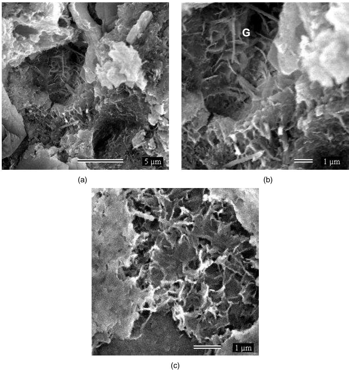
FIGURA 4.15 – Microscopia da amostra CN50M aos 28 dias. (a) Ampliação de 5.000x. (b) Ampliação de 10.000x. (c) Ampliação de 15.000x
