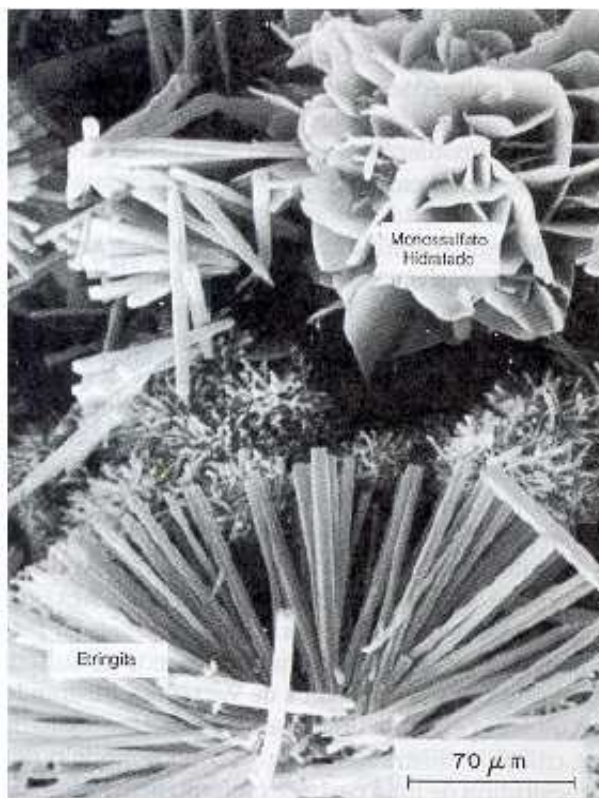
FIGURA 4.8 – Microscopia da pasta de cimento Portland hidratada Fonte: MEHTA e MONTEIRO, 1994.
