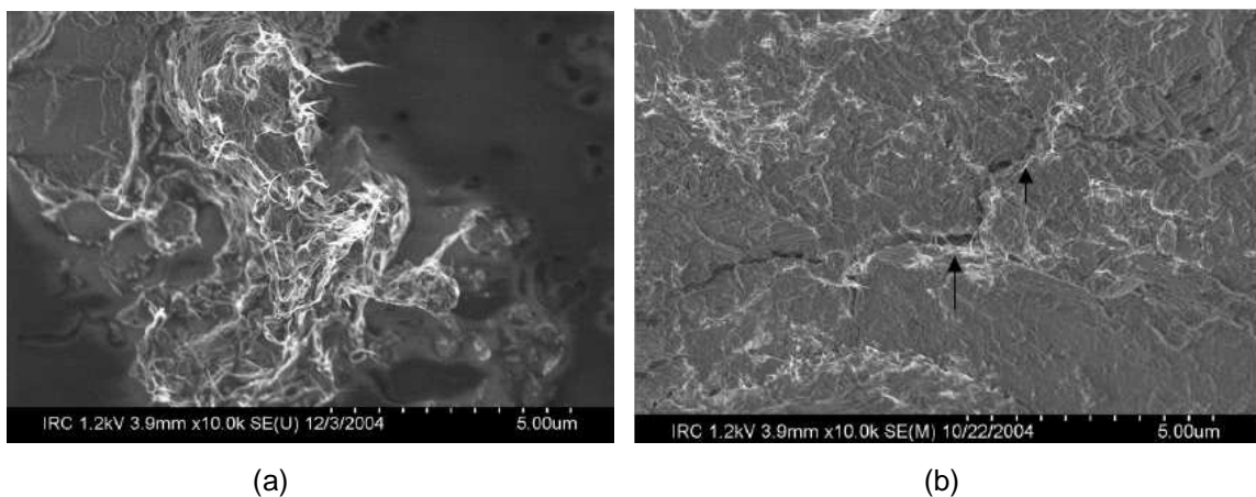
FIGURA 2.21 – (a) Distribuição de feixes de nanotubos de carbono em uma amostra de cimento não hidratada. (b) Imagem de uma fratura superficial em amostra hidratada aos 3 dias Fonte: MAKAR et al. , 2005.
