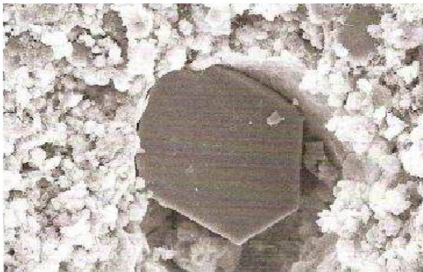
FIGURA 2.4 – Microscopia eletrônica de poro preenchido com cristal hexagonal de hidróxido de cálcio Fonte: PAULON, 2005.
