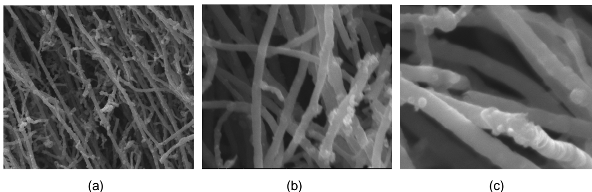
FIGURA 3.4 – Detalhe dos nanotubos produzidos por CVD. (a) Ampliação de 15.000x. (b) Ampliação de 50.000x. (c) Ampliação de 100.000x
