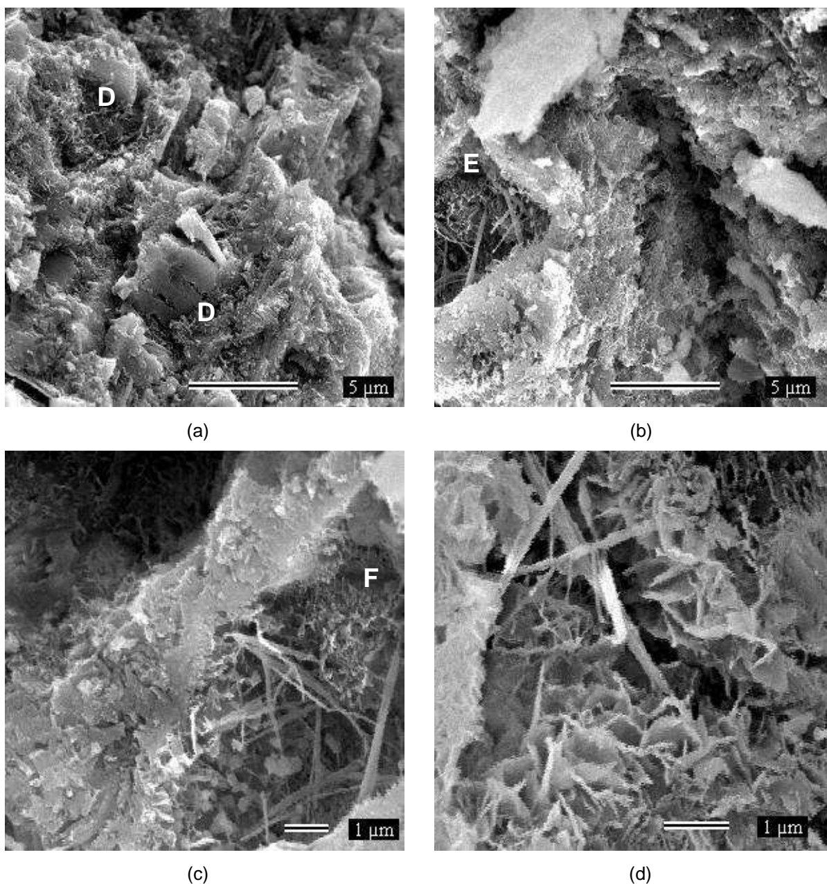
FIGURA 4.14 – Microscopia da amostra CN30M aos 28 dias. (a) e (b) Ampliação de 5.000x. (c) Ampliação de 10.000x. (d) Ampliação de 15.000x
