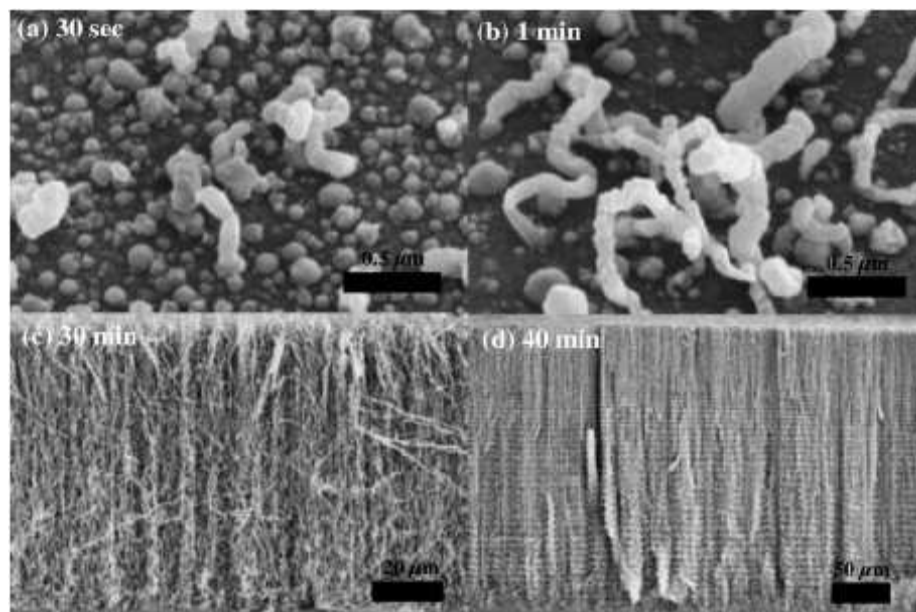
FIGURA 2.18 – MEV do crescimento de NTC pelo método CVD, em função do tempo Fonte: HUH et al. , 2006.
