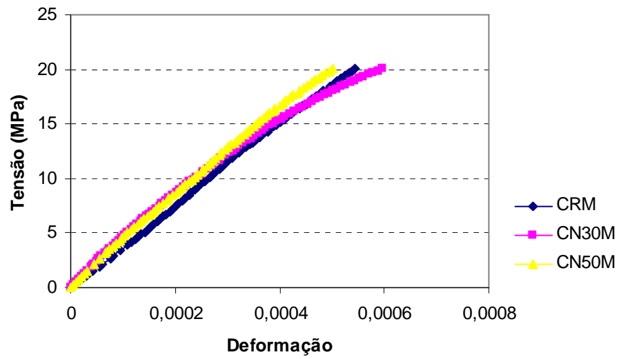
FIGURA A.3 – Relação tensão versus deformação para as argamassas da segunda etapa – 3 dias
