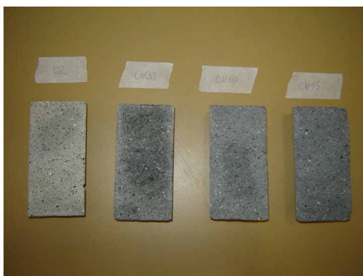
FIGURA 4.3 – Coloração dos quatro traços realizados na primeira etapa: CR, CN30, CN50 e CN75 (da esquerda para direita)
