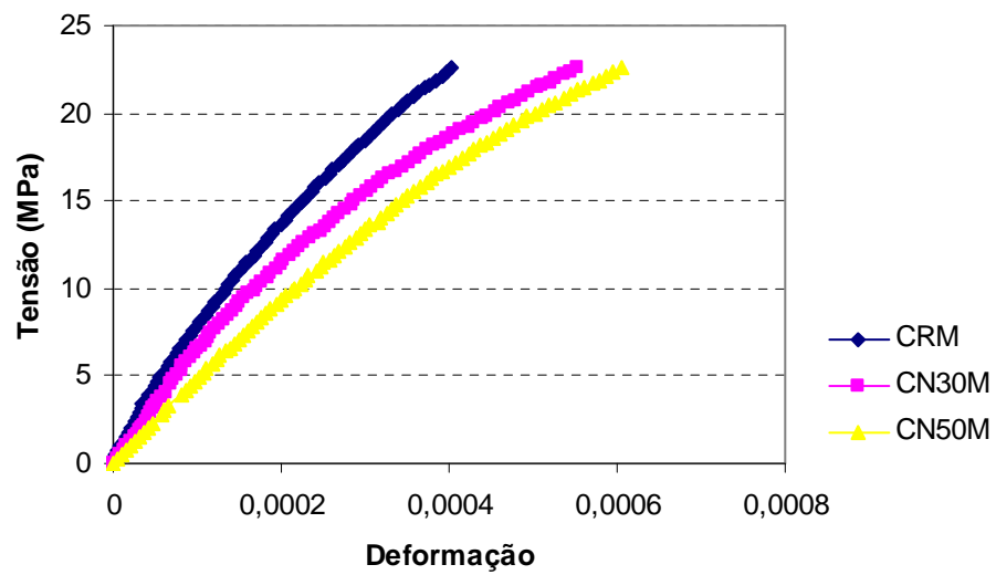
FIGURA A.4 – Relação tensão versus deformação para as argamassas da segunda etapa – 7 dias
