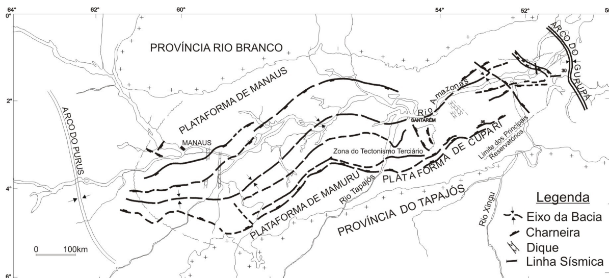
Figura 2.17 - Compartimentação tectônica da Bacia do Amazonas (Wanderley Filho 1991).
