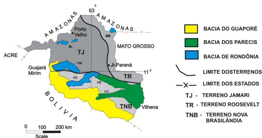
Figura 2.3 - A porção sudoeste do Cráton Amazônico dividida em terrenos geológicos (modificado de Amorim et al. 1999).
