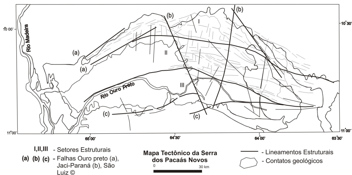
Figura 2.8 - Mapa Tectônico da Serra dos Pacaás Novos.
