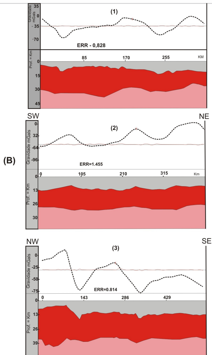
Figura 3.12 - Mapa gravimétrico da Baía dos Parecís (A) com os perfis gravimétricos modelados (B), apresentando a camada sedimentar (cinza), sobre o embasamento cristalino (vermelho).
