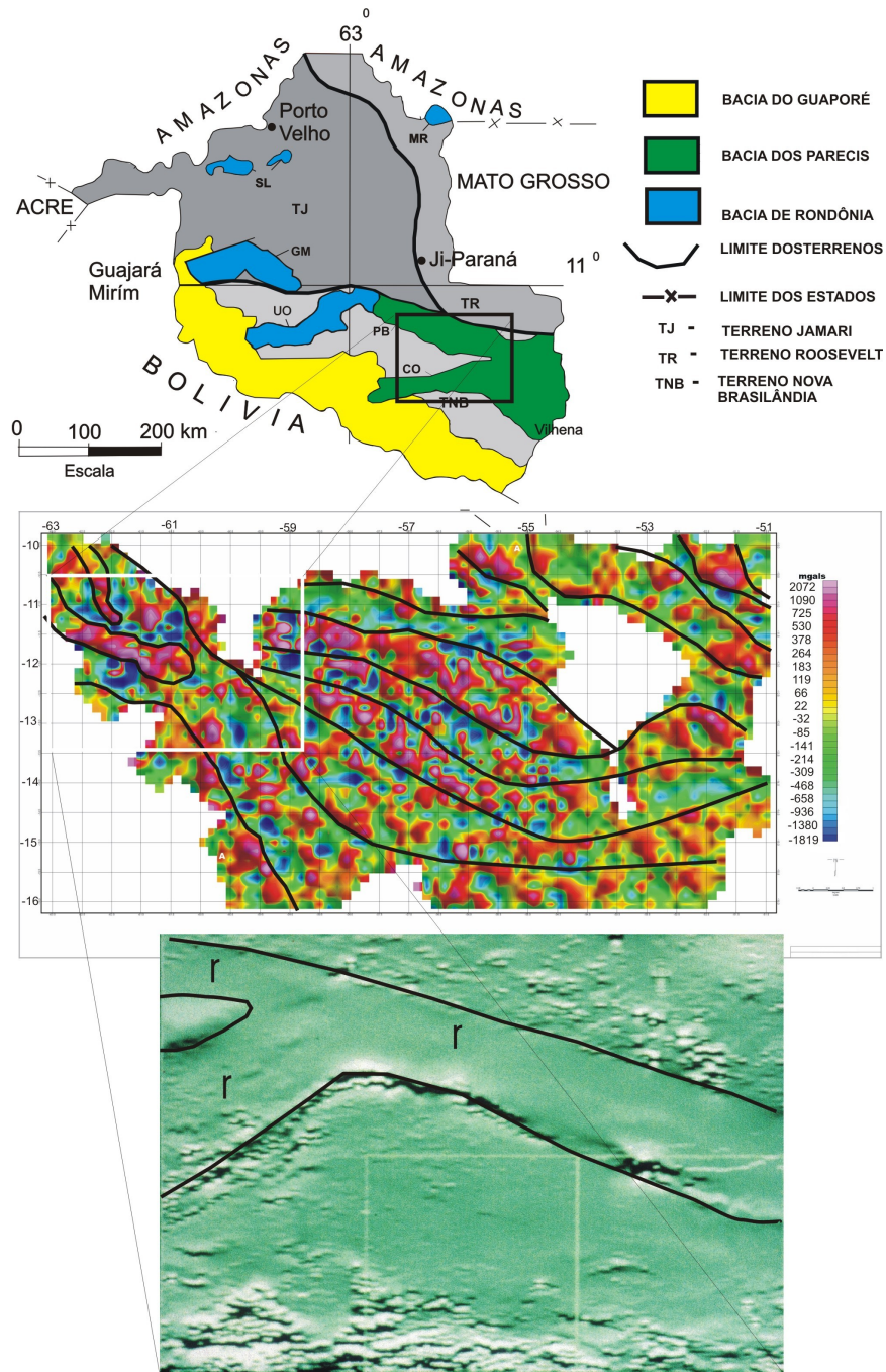
Figura 3.51 - Imagem magnética de pseudoiluminação da porção oeste da Bacia dos Parecis, mostrando os riftes precursores da mesma (textura lisa), embasada na interpretação do mapa magnético de contagem total .
