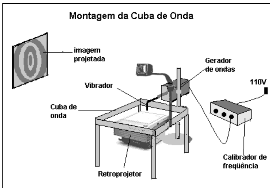
FIGURA - 2 Cuba de onda
