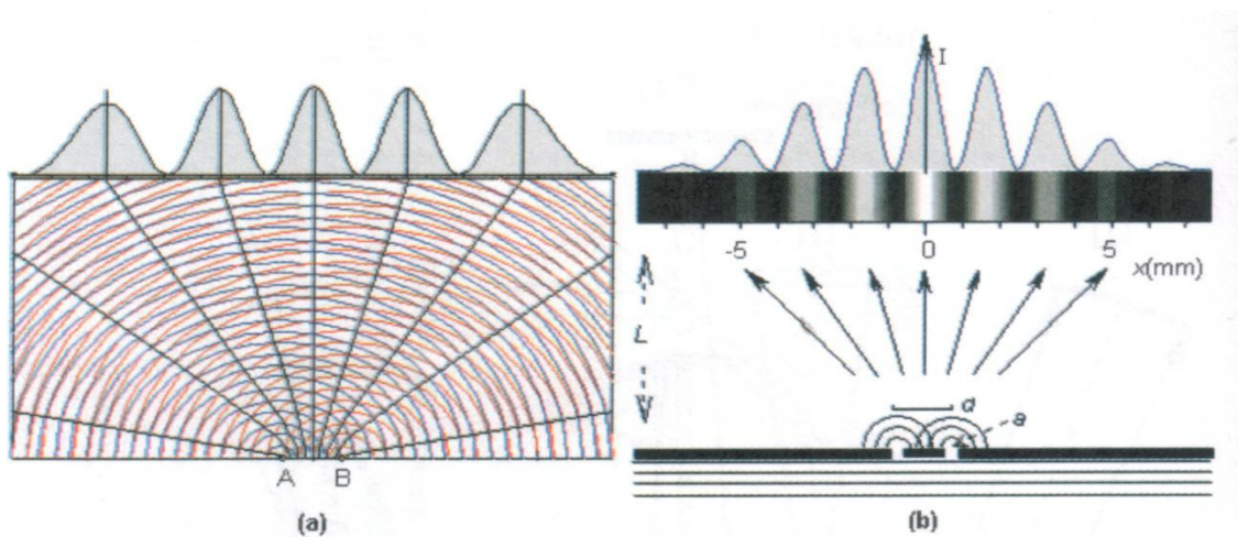
FIGURA - 3 Difração e figuras de interferência (a) e Interferência modulada pela difração (b)
