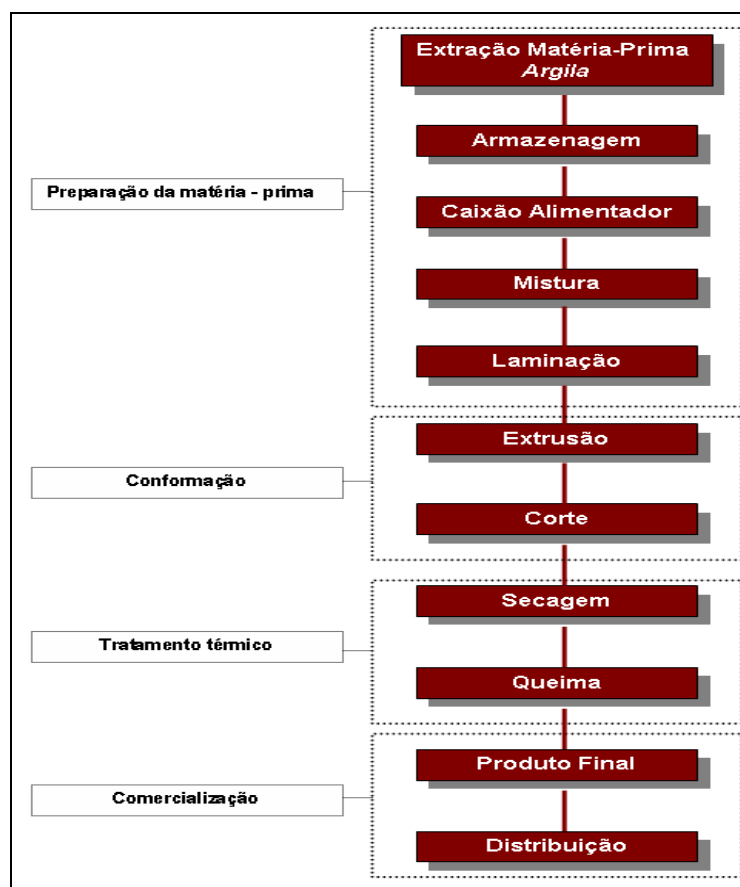
Figura 5.2 – Fluxograma do processo produtivo.
