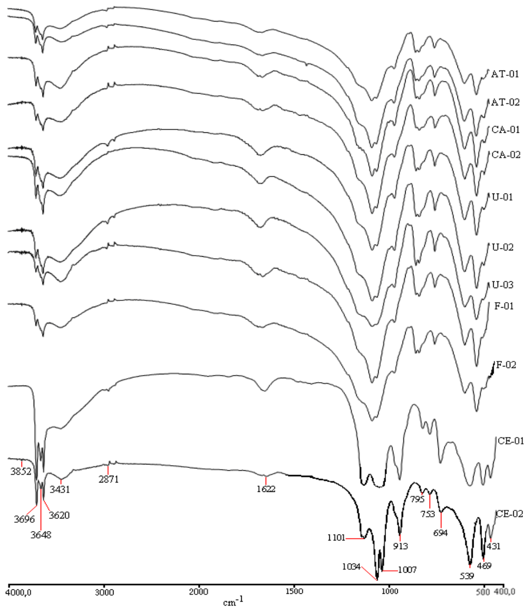
Figura 4.11 – Espectros de Infravermelho Amapá Telhas 01 (AT-01), Amapá Telhas 02 (AT-02), Calandrini 01 (CA-01), Calandrini 02 (CA-02), União 01 (U-03), União 02 (U-02), União 03 (U-03) Fortaleza 01 (F-01), Fortaleza 02 (F-02), Corte de Estrada 01 (CE-01) e Corte de Estrada 02 (CE-02).
