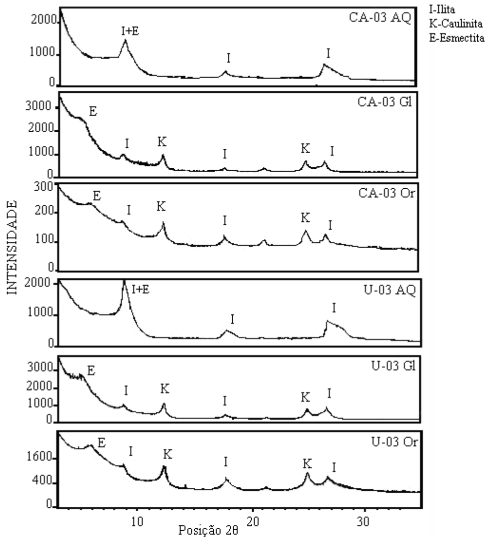
Figura 4.6 – Difractogramas de lâminas orientadas, tratadas com etilenoglicol e aquecidas a 500 °C das amostras: União 03 (U-03), Calandrini 03 (CA-03).
