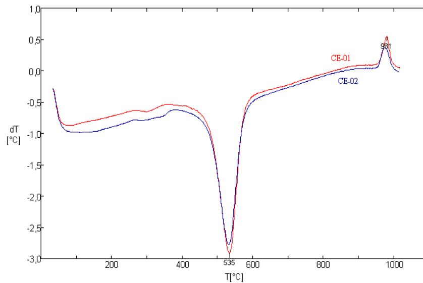
Figura 4.10 – Termogramas das Análises Térmicas Diferenciais (DTA) das amostras Corte de Estrada - 01 (CE-01) e Corte de Estrada-02 (U-03).
