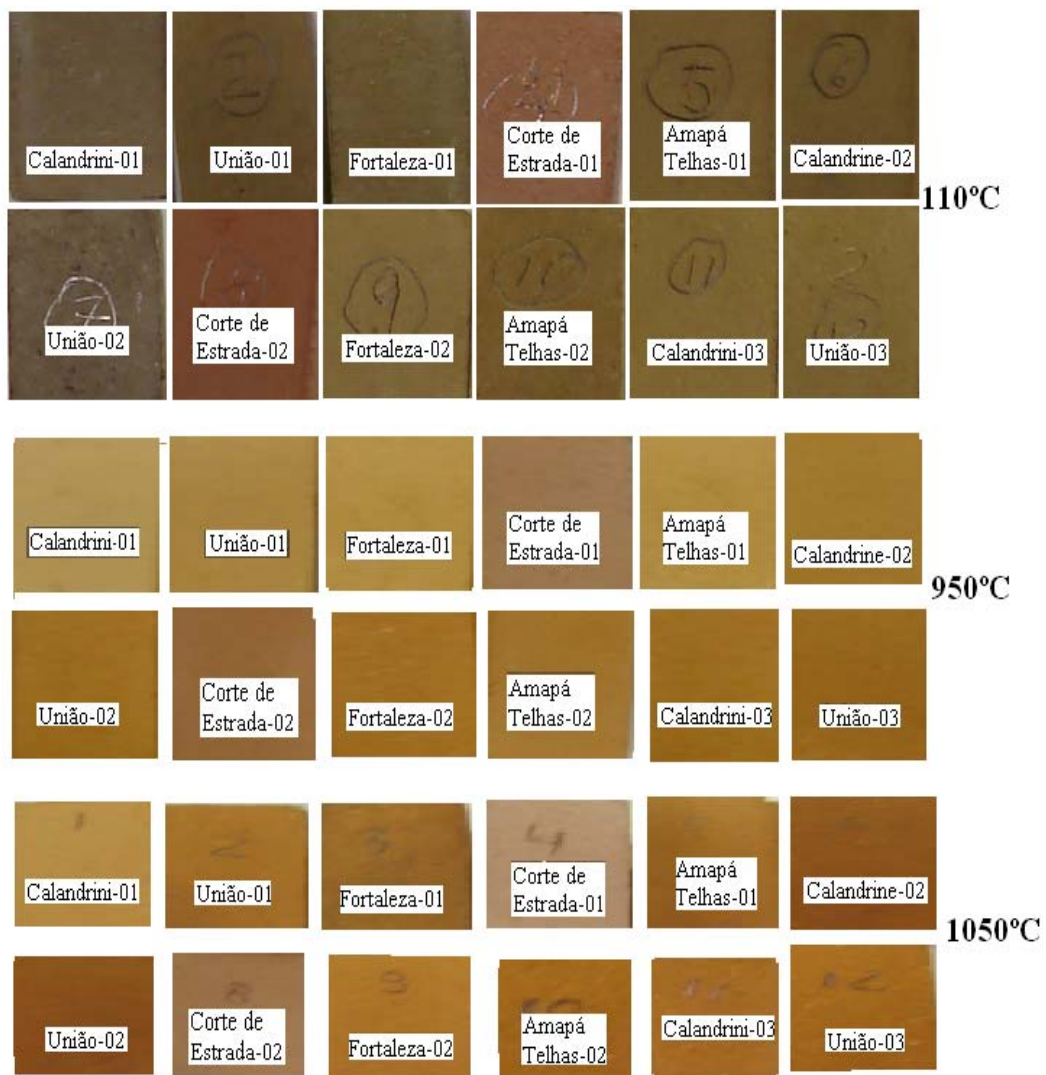
Figura 4.13 – Corpos de provas secos a 110°C, queimados a 950°C e a 1050°C.
