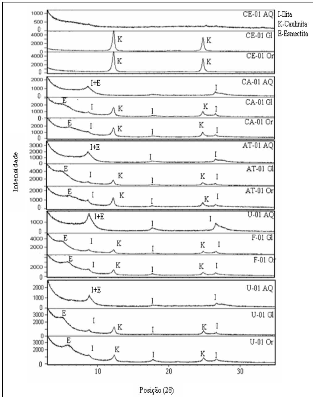
Figura 4.2 – Difratogramas de lâminas orientadas (OR), tratadas com etilenoglicol (GL) e aquecidas a 500°C (AQ) das amostras: Amapá Telhas 01 (AT-01), União 01 (U-01), Corte de Estrada 01 (CE-01) e Fortaleza 01 (F-01) e Calandrini 01 (CA-01).
