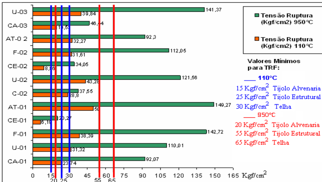
Figura 4.14 – Relação entre os valores medidos para tensão de ruptura à flexão das amostras estudadas e valores-limites recomendados para fabricação de tijolos de alvenaria, estrutural e telhas.
