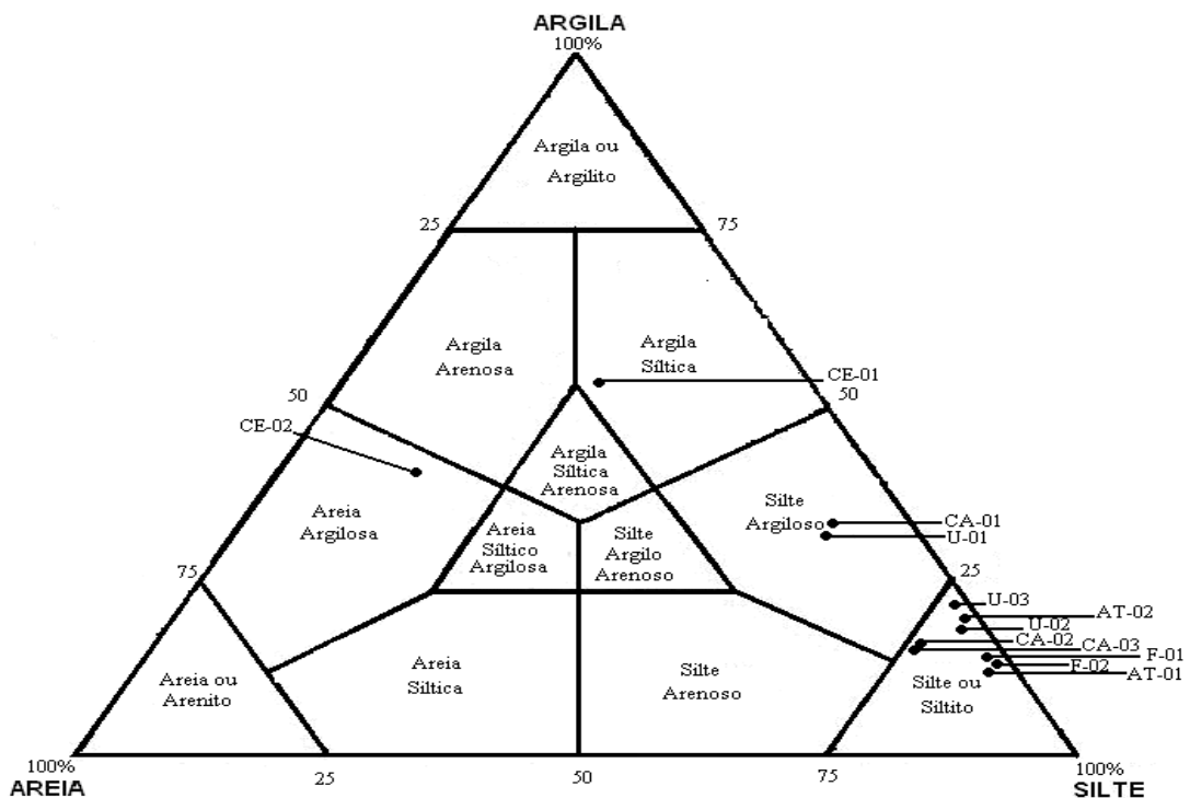
Figura 4.12 – Classificação litológica através da análise granulométrica de acordo com Shepard (apud Suguio, 1973).
