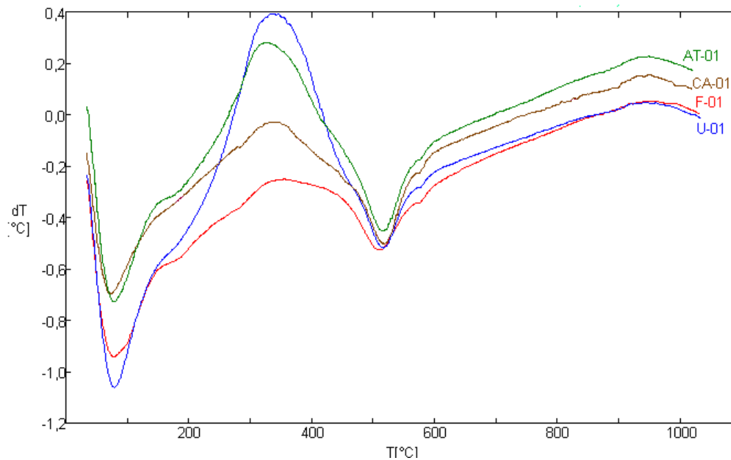
Figura 4.7 – Termogramas de Análise Térmica Diferencial (DTA) das amostras: Amapá Telhas 01 (AT-01), Calandrini 01 (CA-01), Fortaleza 01 (F-01), União 01 (U-01).
