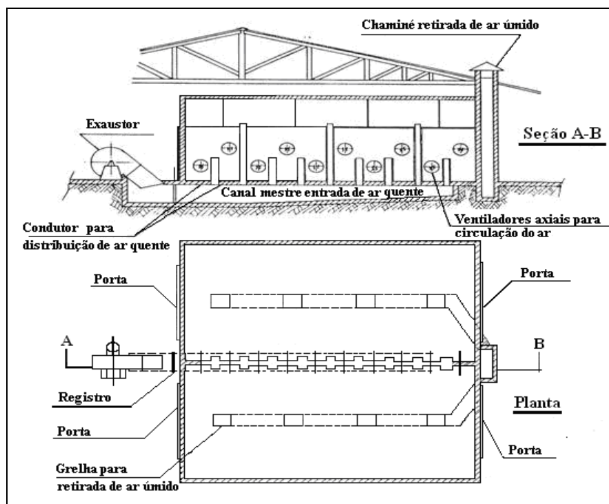
Figura 5.9 – Desenho esquemático de estufas artificiais.
