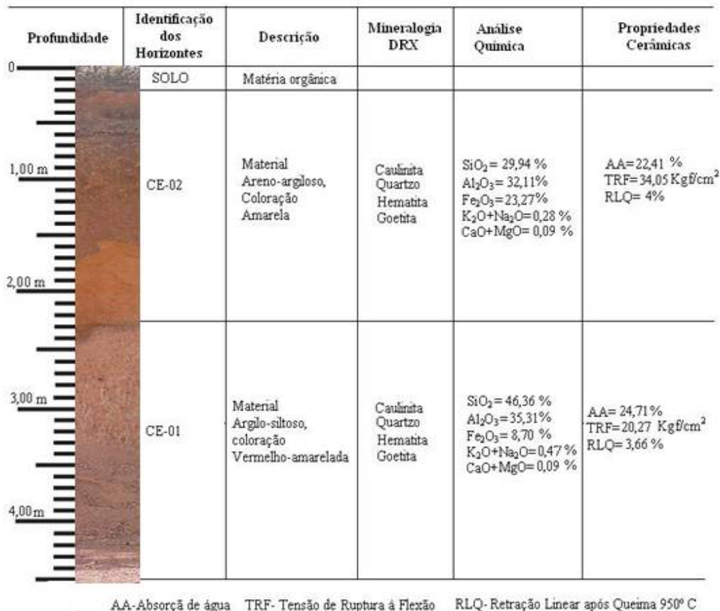
Figura 4.21 – Coluna Litoestratigráfica do Corte de Estrada relacionada com as análises mineralógicas (DRX), químicas e propriedades tecnológicas (AA, TRF e RLQ).
