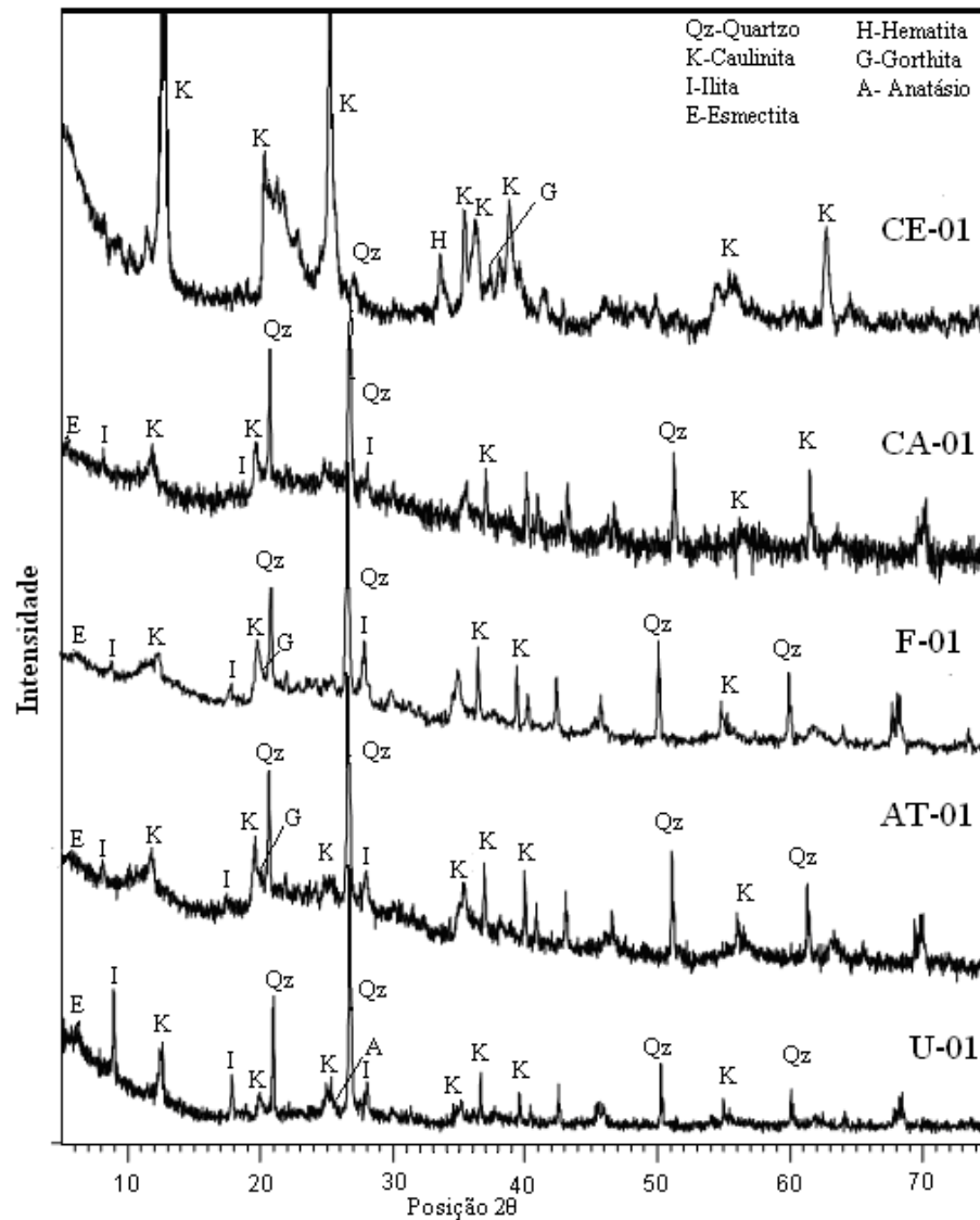
Figura 4.1 – Difatogramas das amostras presentes no nível 1: União 01(U-01), Fortaleza 01 (F-01), Corte de Estrada 01 (CE-01), Calandrine 01 (CA-01), Amapá Telhas 01 (AT-01).
