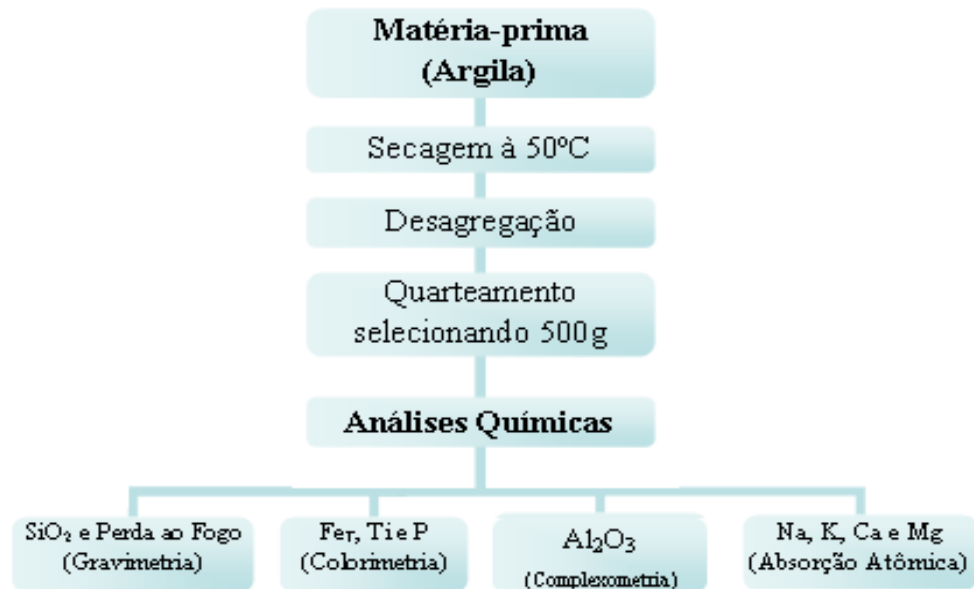
Figura 3.5 – Fluxograma de tratamento de amostras para a análise química.
