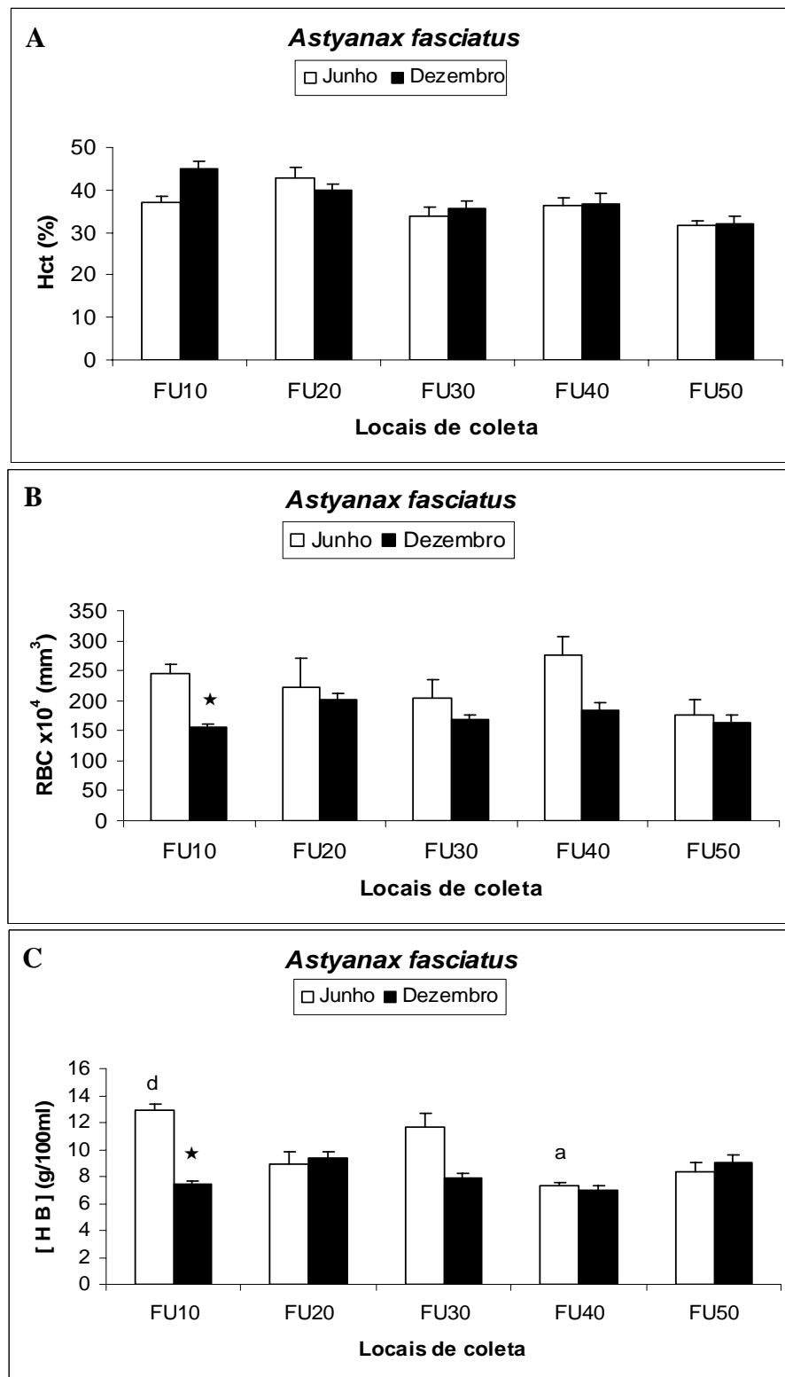
Figura 1. Médias \pm erro padrão de A. hematócrito (Hct), B. número total de eritrócitos (RBC) e C. concentração de hemoglobina ([HB]) de A. fasciatus coletados em cinco diferentes locais da UHE de Furnas: FU10 (Turvo); FU20 (Guapé); FU30 (Barranco alto); FU40 (Fama) e FU50 (Porto Fernandes) durante os meses de Junho e Dezembro/2006. a, b, c, d, e: indicam diferença em relação aos locais FU10; FU20; FU30; FU40 e FU50. ★: indica diferença entre a coleta de Junho e Dezembro/2006.
