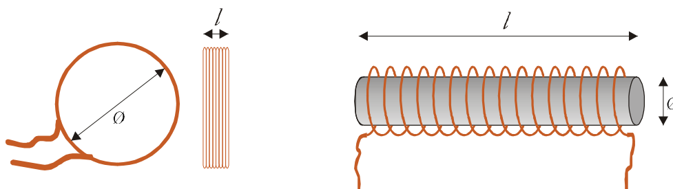
Figura 28: Formas de bobina avaliadas para bobina de leitura (a) bobina tipo anel. (b) bobina tipo solenóide.
