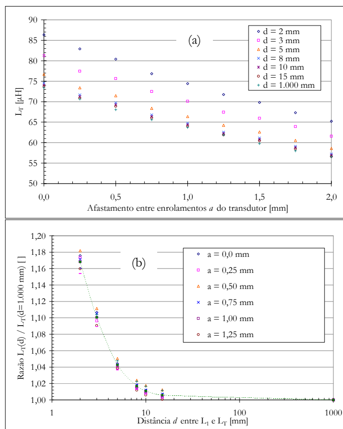
Figura 46: Comportamento da indutância própria do transdutor (a) em relação ao afastamento entre seus enrolamentos e diferentes distâncias de acoplamento e (b) a razão entre os valores de L_T com e sem a presença de L_1 para diferentes afastamentos – a linha tracejada representa a média dos valores.
