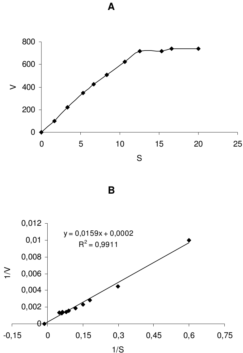
Figura 20. Efeito da concentração de catecol na atividade da PPO. (V) Atividade enzimática (UA/mL); (S) concentração de substrato (mmol/L). (A) Gráfico de Michaelis-Menten; (B) gráfico duplo recíproco Lineweaver-Burk.
