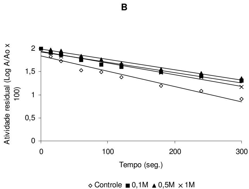
Figura 27. Efeito do KCl na inativação térmica da PPO de atemóia. (A) 55°C; (B) 60°C. A PPO purificada foi incubada na presença de 0, 0,1M, 0,5M e 1M de KCl, a inativação térmica acompanhada conforme descrito em material e métodos.
